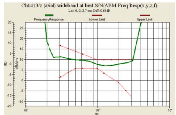
Fig. 7.4 WCDMA Band IV Ch1413
