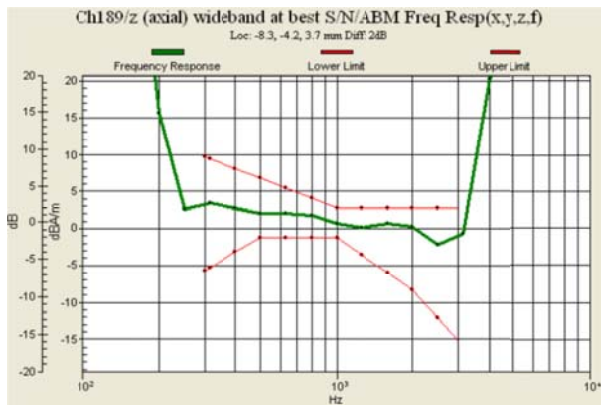
Fig 7.1 GSM850 Ch189
