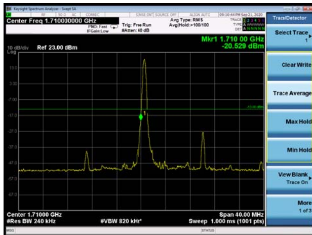
EN-DC_2A_n66 20MHz QPSK 100%RB CH-Low
