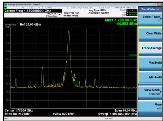
EN-DC_2A_n66 20MHz QPSK 100%RB CH-High
