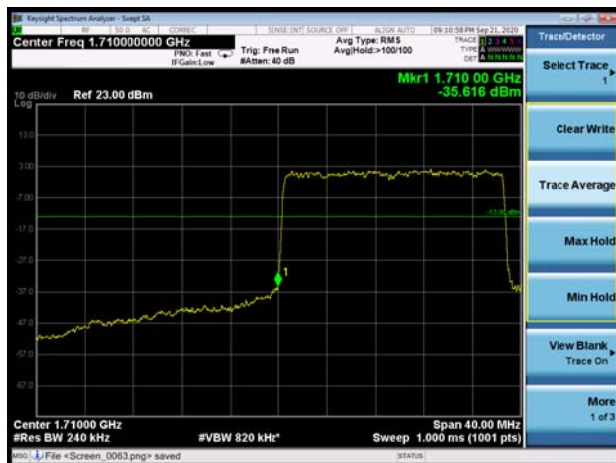
EN-DC_2A_n66 20MHz 16QAM 1RB CH-Low
