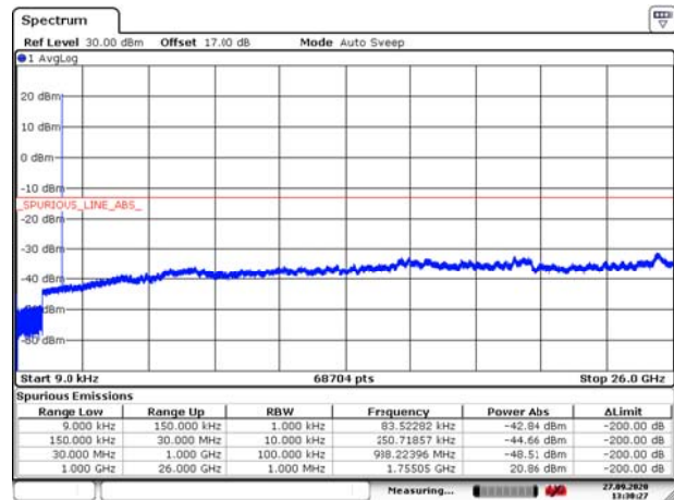
EN-DC_2A_n66 10MHz CH- Low 9kHz~26GHz
