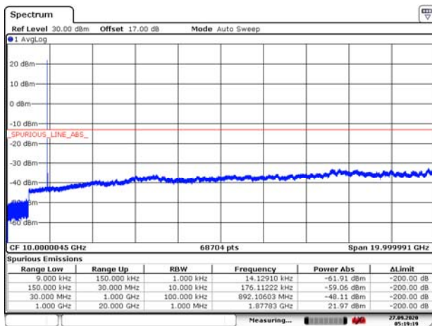
EN-DC_5A_n2 5MHz CH-Middle 9kHz~20GHz
