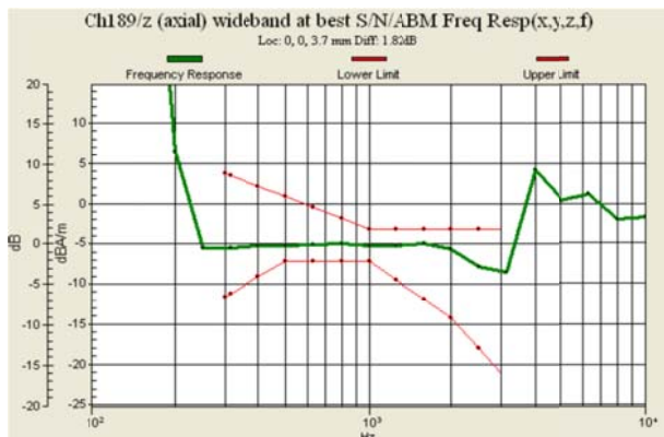
Fig 7.1 GSM850 Ch189
