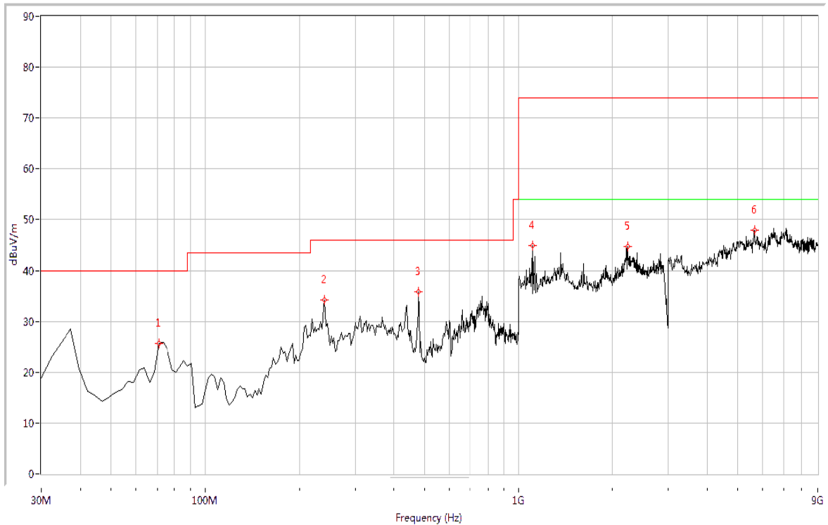
(Plot B: 30MHz – 9GHz, Test Antenna Horizontal)
