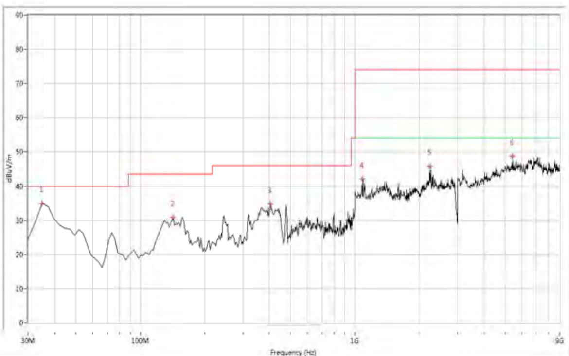
(Plot A: 30MHz – 9GHz, Test Antenna Vertical)
