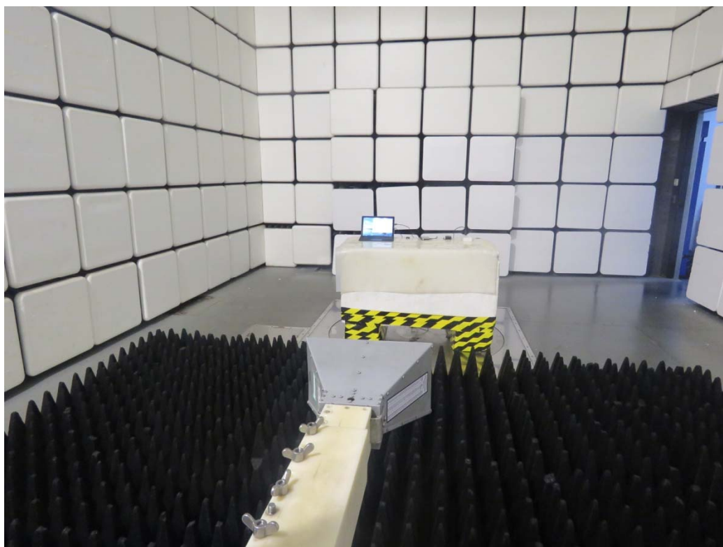
1GHz-18GHz
