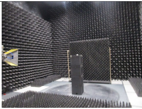
1-18 GHz
