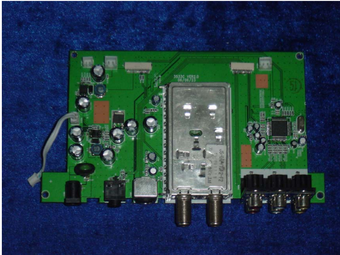
PCB Top
