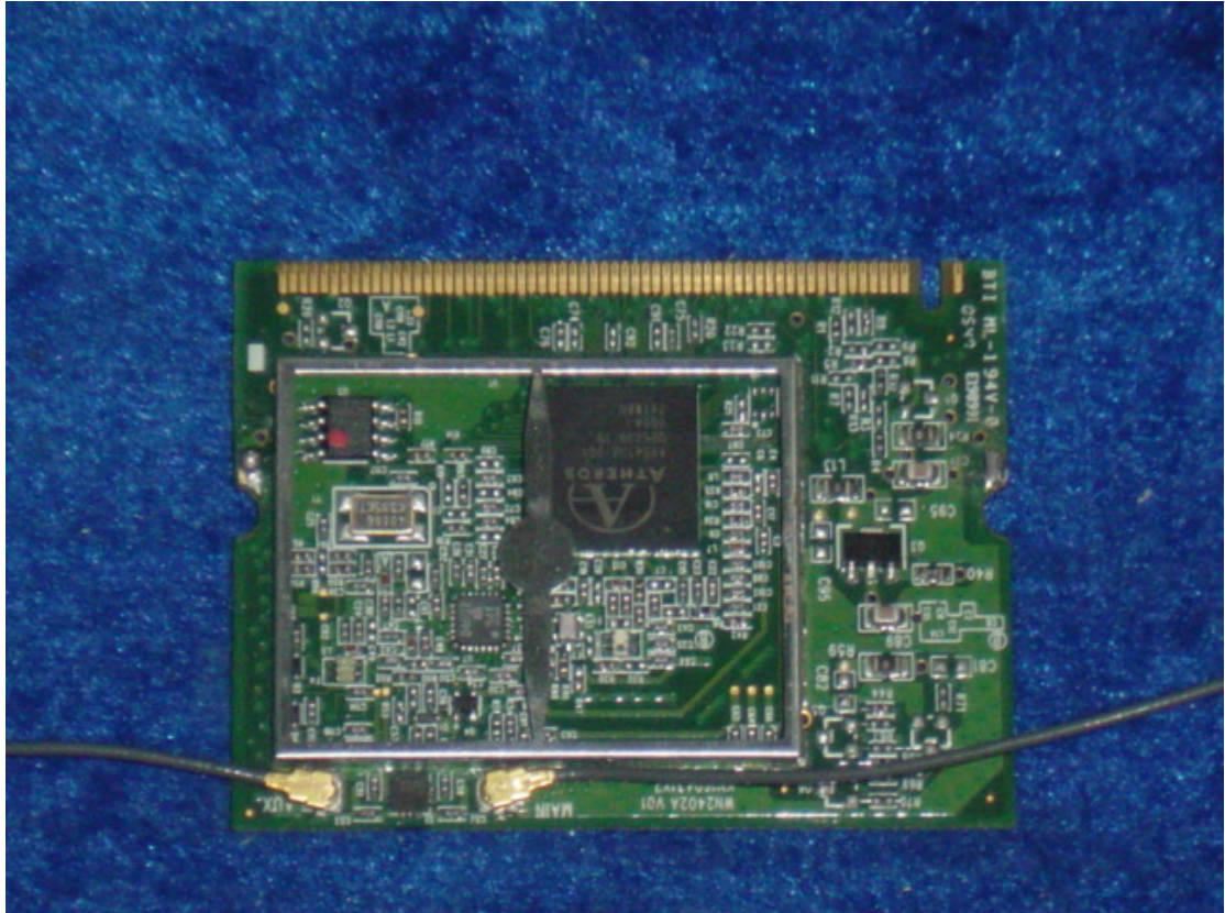
PCB Bottom
