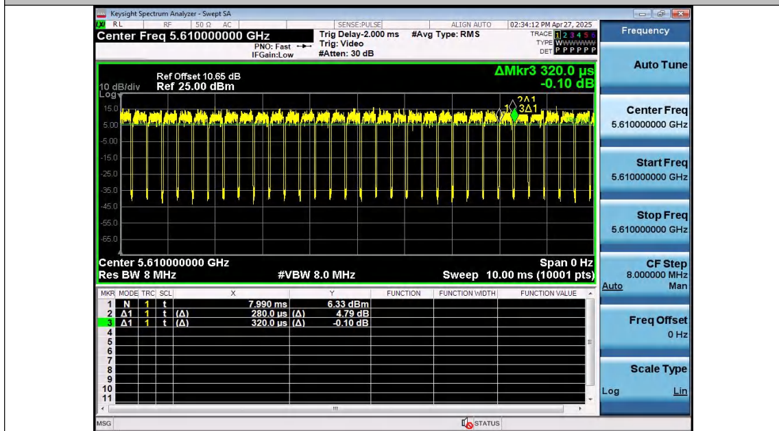
NTNV-11AX80SISO-Ant1-5610
