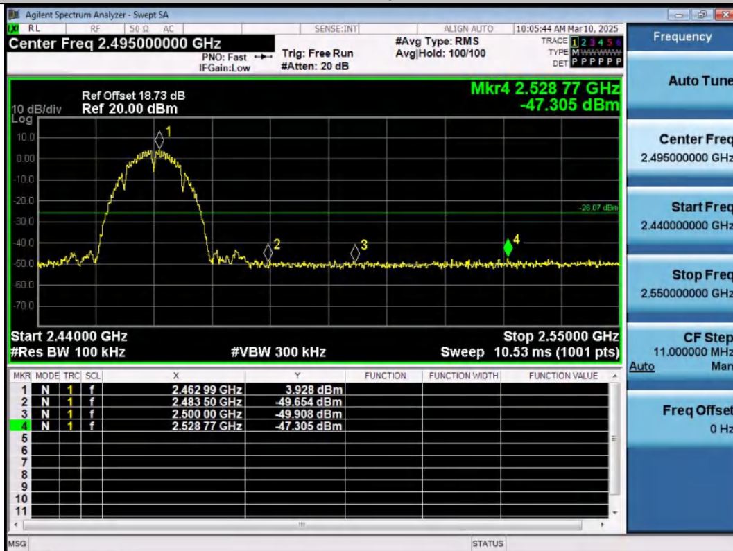
11B-Ant2-2462-PASS
