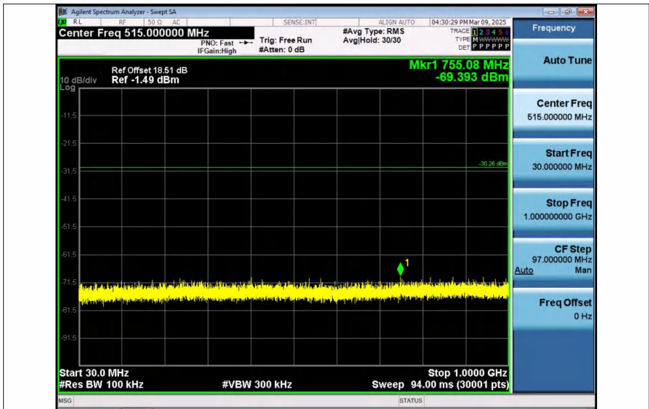
11G-Ant1-2412-30~1000-PASS
