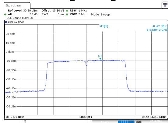
802.11ac80_5610MHz_Chain 0
