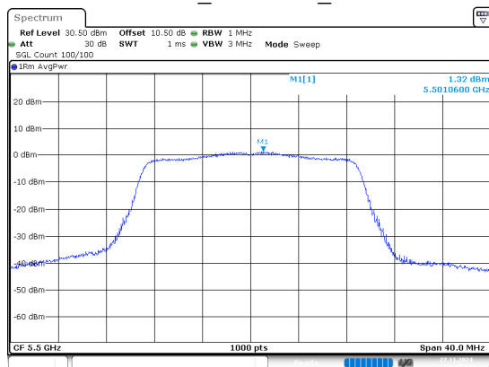
802.11n20_5500MHz_Chain 0
