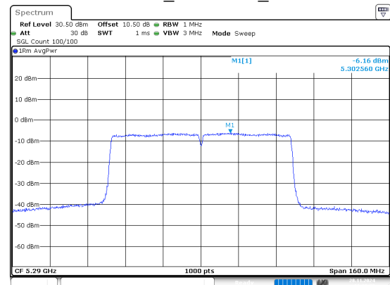
802.11ac80_5290MHz_Chain 1
