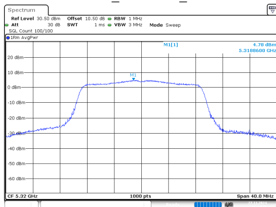
802.11n20_5320MHz_Chain 0
