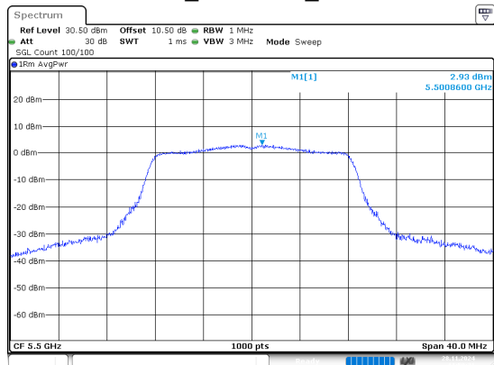
802.11a_5500MHz_Chain 1
