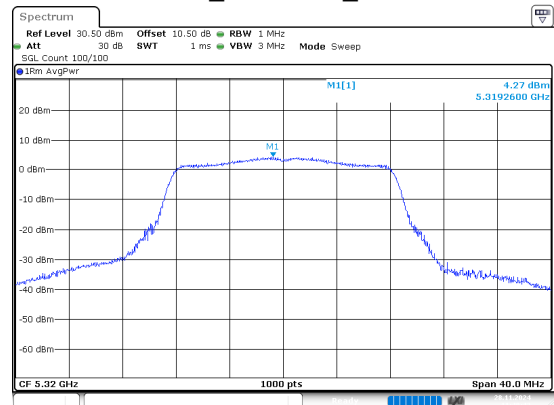
802.11a_5320MHz_Chain 1
