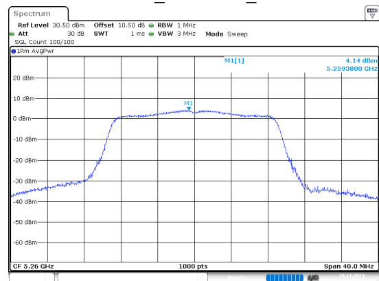
802.11n20_5260MHz_Chain 1
