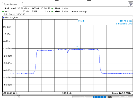
802.11ac80_5610MHz_Chain 1
