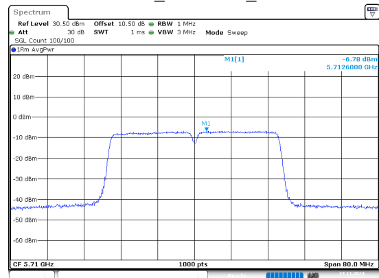
802.11n40_5710MHz_Chain 0
