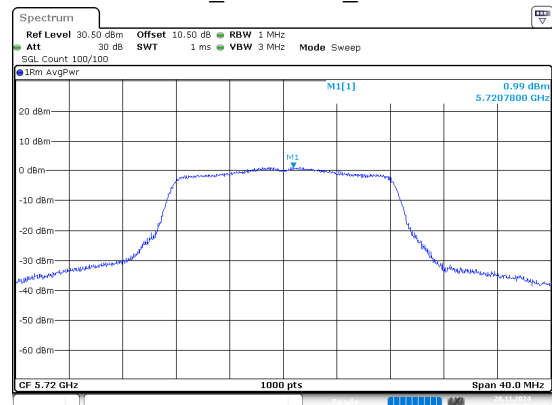
802.11a_5720MHz_Chain 1
