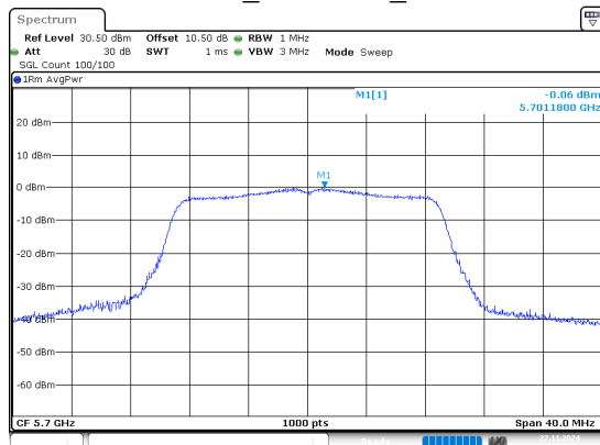
802.11n20_5700MHz_Chain 0
