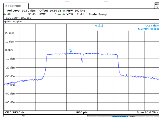
802.11n40_5795MHz_Chain 1
