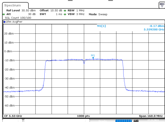
802.11ac80_5530MHz_Chain 0
