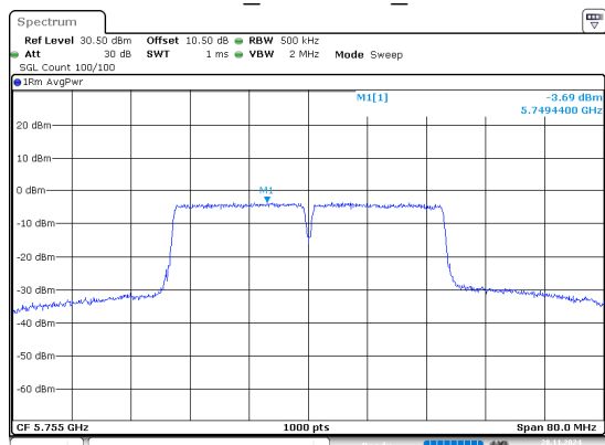
802.11n40_5755MHz_Chain 1
