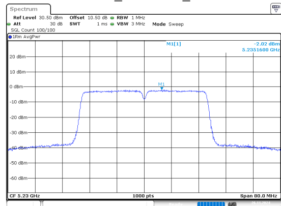
802.11n40_5230MHz_Chain 0
