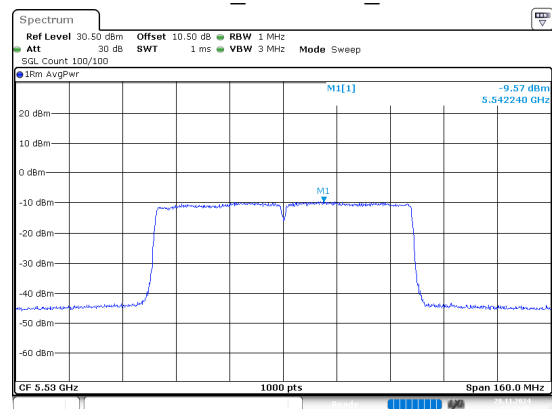
802.11ac80_5530MHz_Chain 1
