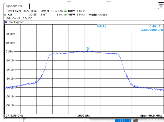
802.11n20_5580MHz_Chain 0
