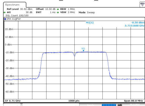
802.11n40_5710MHz_Chain 1
