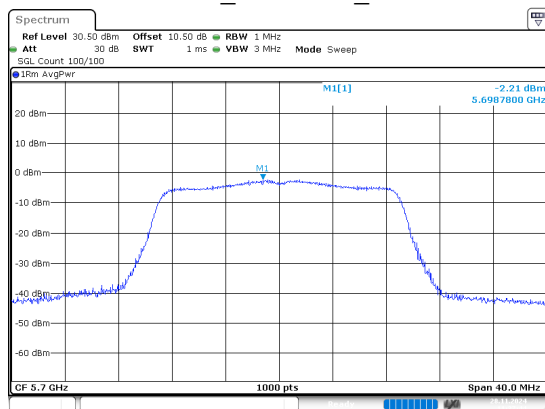
802.11n20_5700MHz_Chain 1
