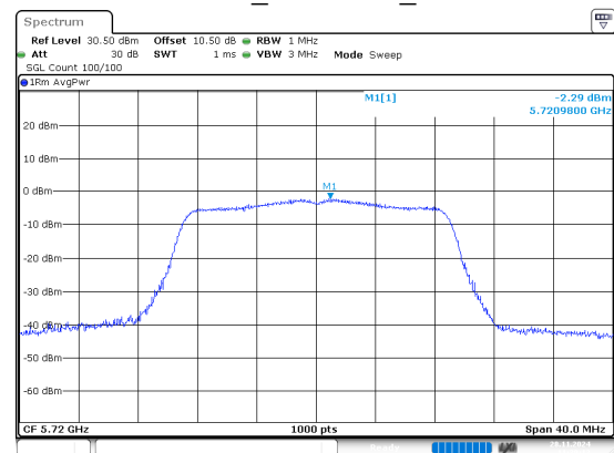
802.11n20_5720MHz_Chain 1
