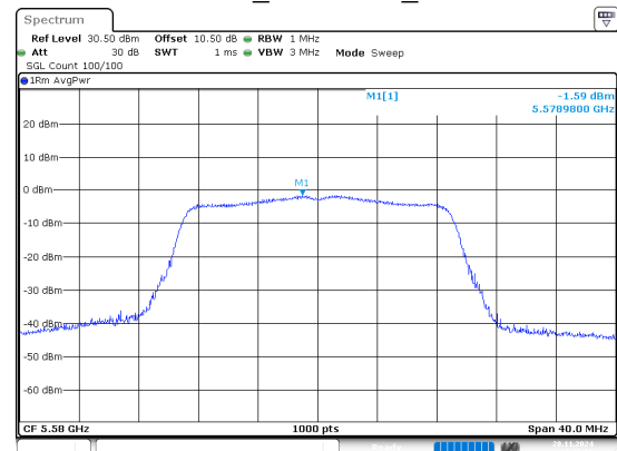
802.11n20_5580MHz_Chain 1
