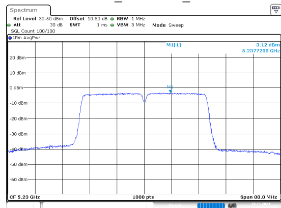
802.11n40_5230MHz_Chain 1
