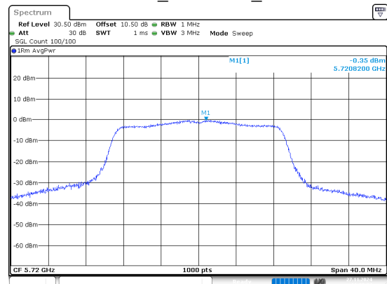
802.11n20_5720MHz_Chain 0
