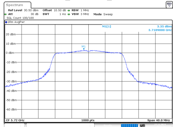
802.11a_5720MHz_Chain 0
