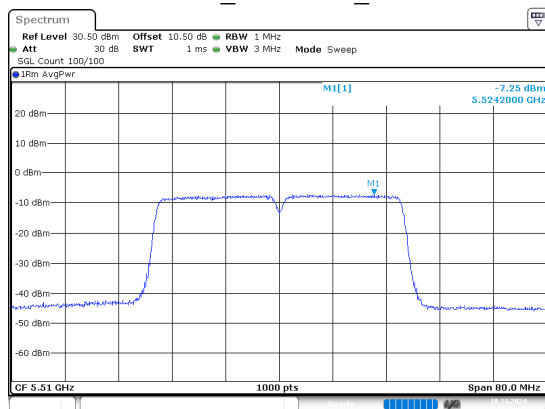
802.11n40_5510MHz_Chain 1
