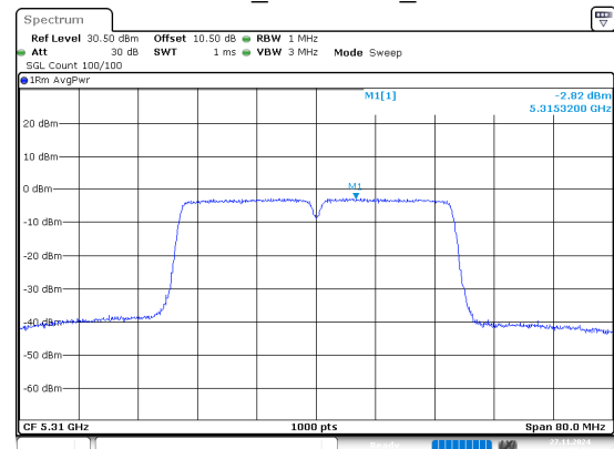
802.11n40_5310MHz_Chain 0
