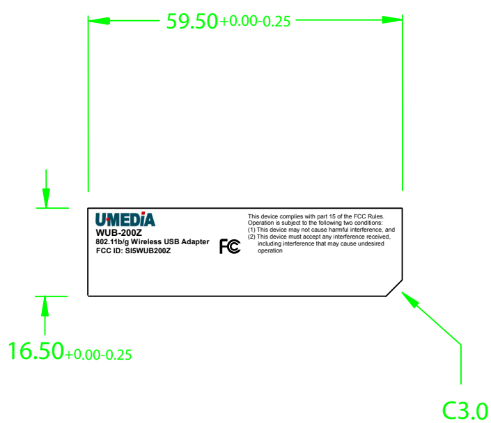
WUB-200Z_Label Dim.
