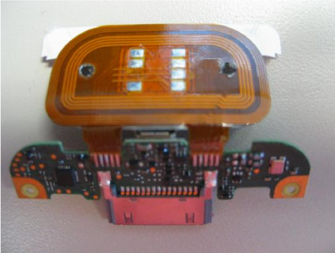
Top side
