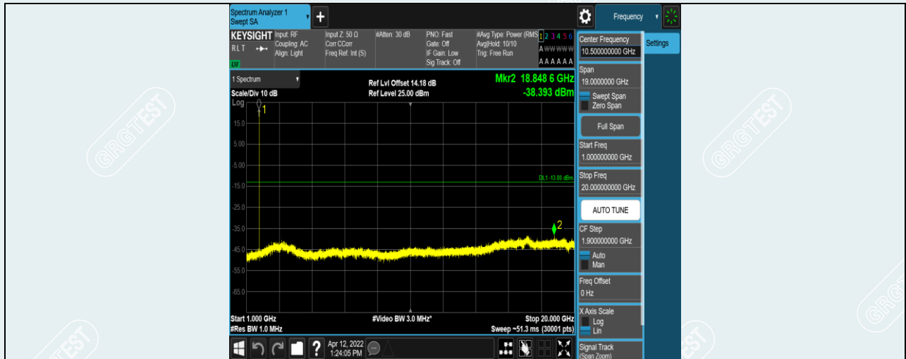
Band4-5MHz-QPSK-20175-1RB#0-Range2:1000~20000MHz
