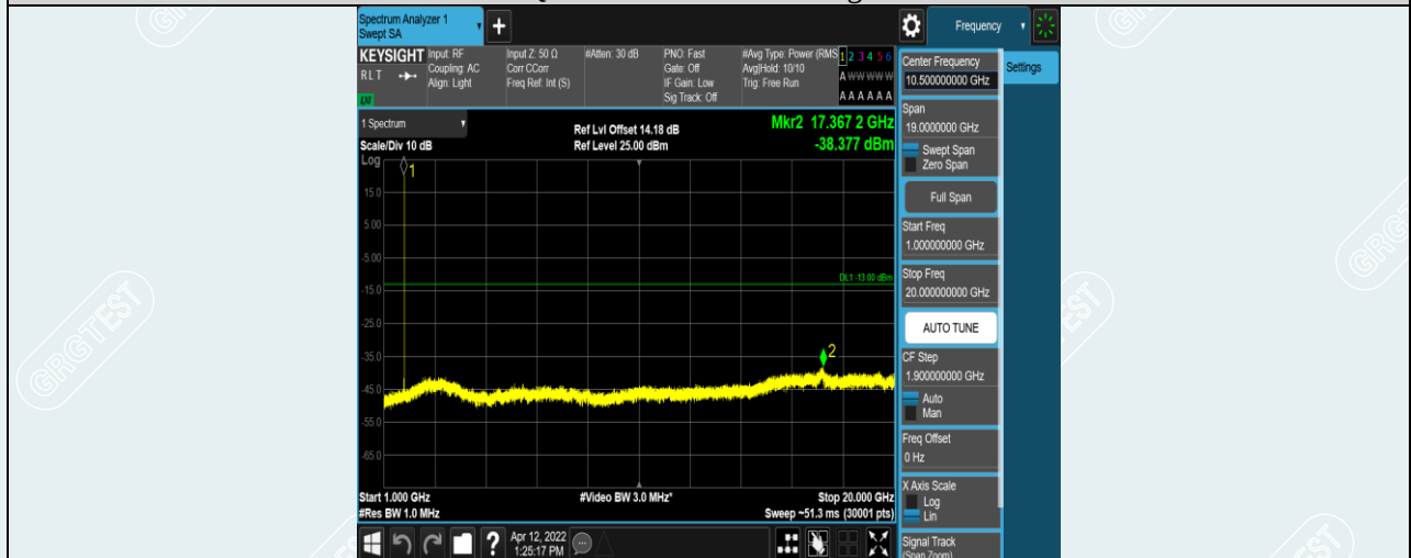
Band4-5MHz-QPSK-20375-1RB#0-Range2:1000~20000MHz
