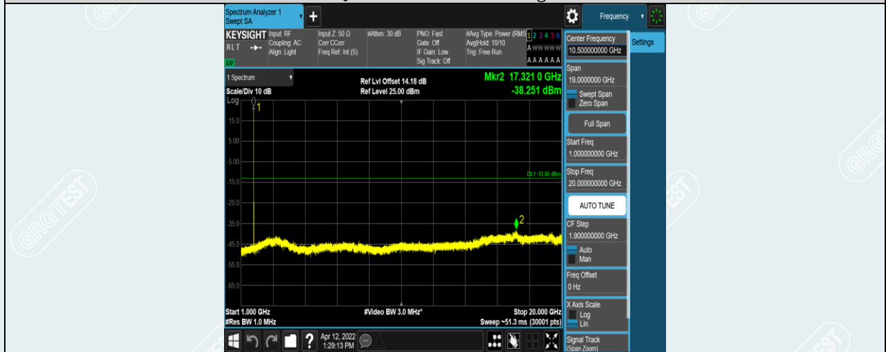
Band4-10MHz-QPSK-20350-1RB#0-Range2:1000~20000MHz
