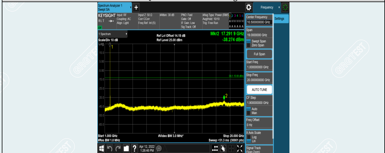
Band4-10MHz-QPSK-20000-1RB#0-Range2:1000~20000MHz
