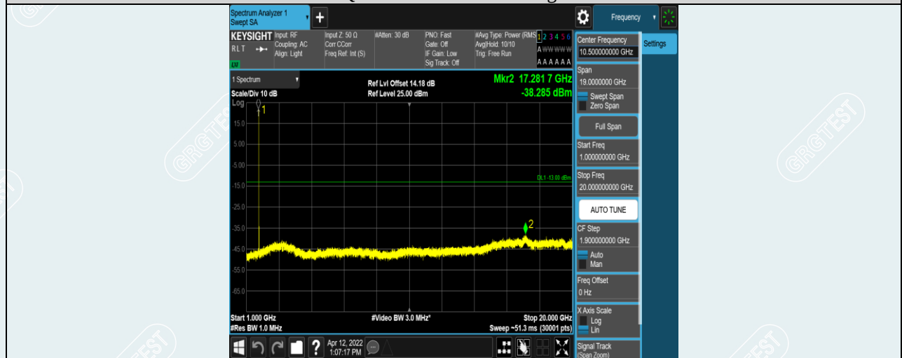
Band4-15MHz-QPSK-20025-1RB#0-Range2:1000~20000MHz
