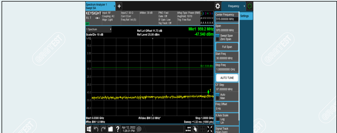
Band4-10MHz-QPSK-20000-1RB#0-Range1:30~1000MHz
