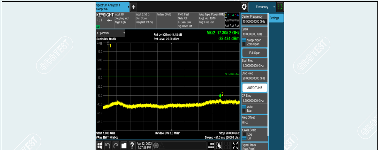
Band4-10MHz-QPSK-20175-1RB#0-Range2:1000~20000MHz
