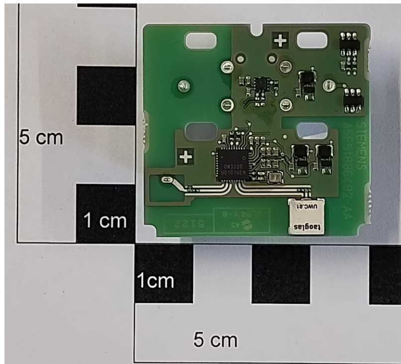
PCB bottom
