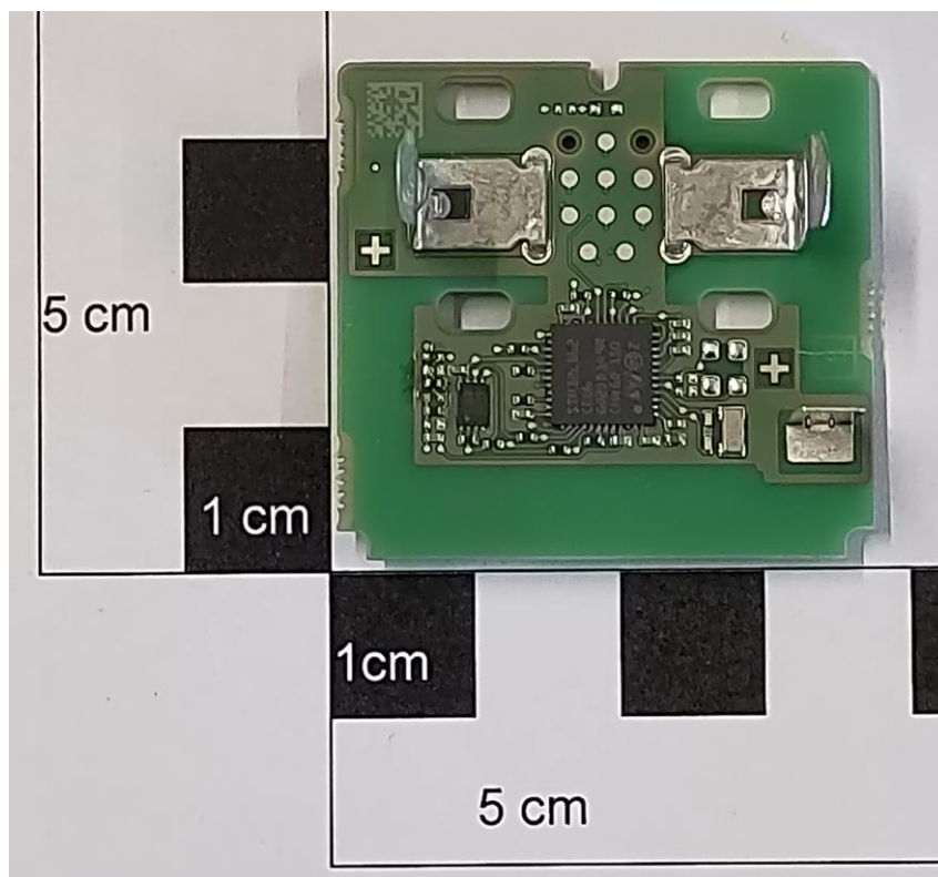
PCB top
