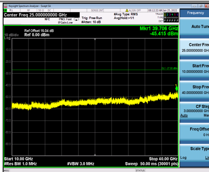
11N20MIMO_Ant1_6995_10000~40000
