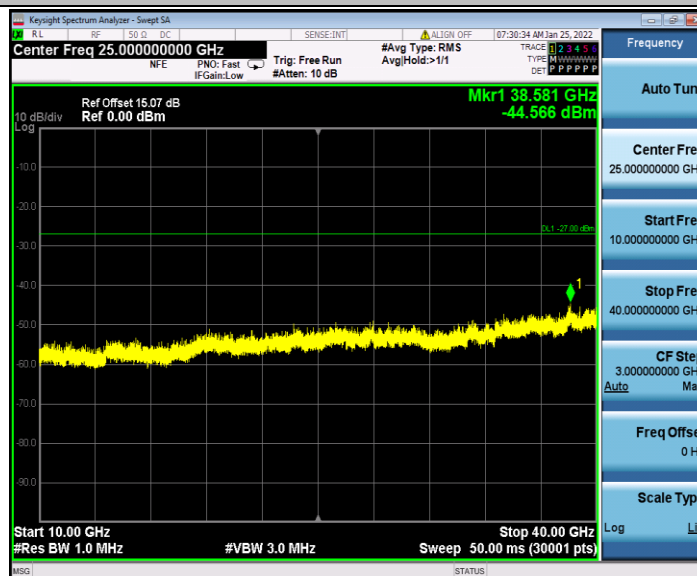
11N20MIMO_Ant2_6695_10000~40000
