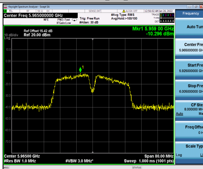
11N40MIMO_Ant2_5965
