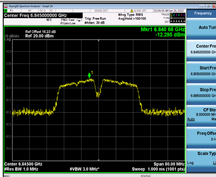
11N40MIMO_Ant1_6845
