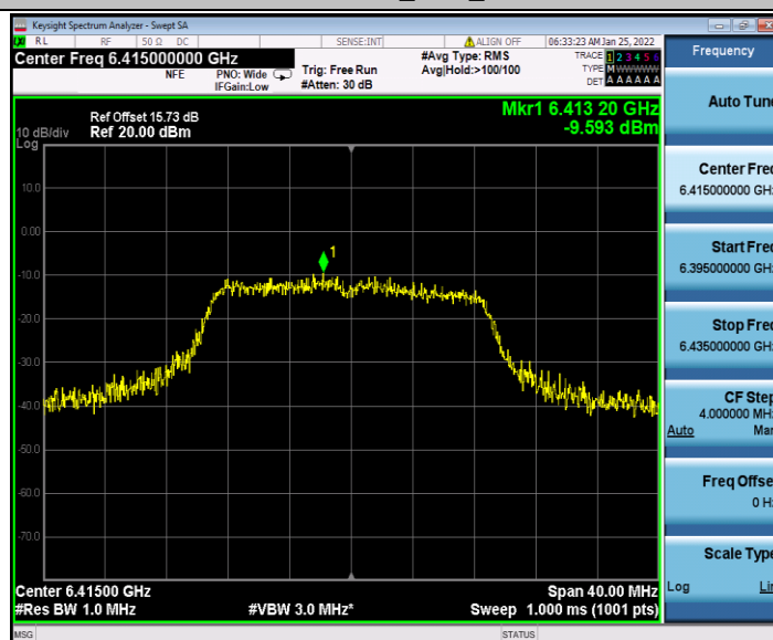
11N20MIMO_Ant2_6415
