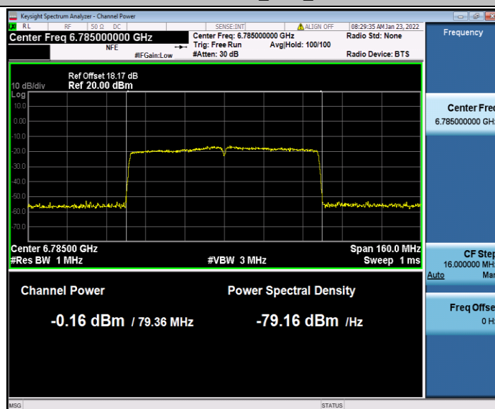
11AC80SISO_Ant1_6785
