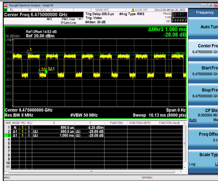
11AC20MIMO_Ant2_6475
