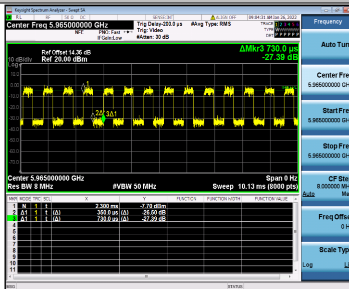
11AC40MIMO_Ant2_5965
