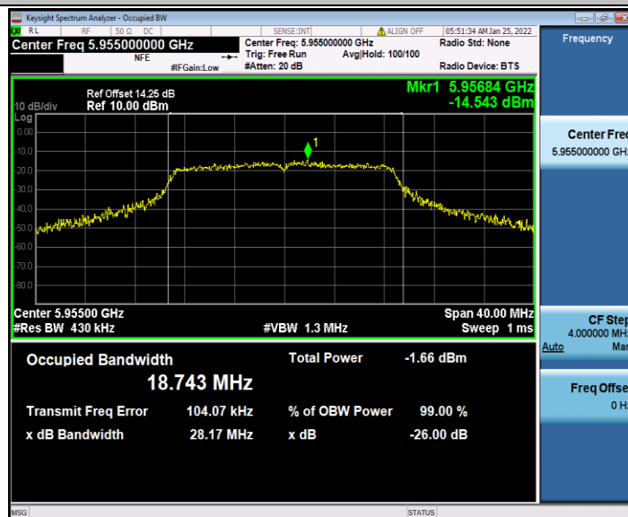
11N20MIMO_Ant1_5955
