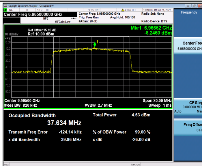
11AX40SISO_Ant2_6965
