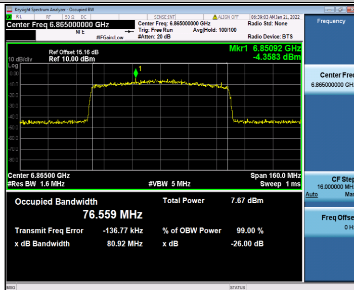
11AX80ISO_Ant2_6865
