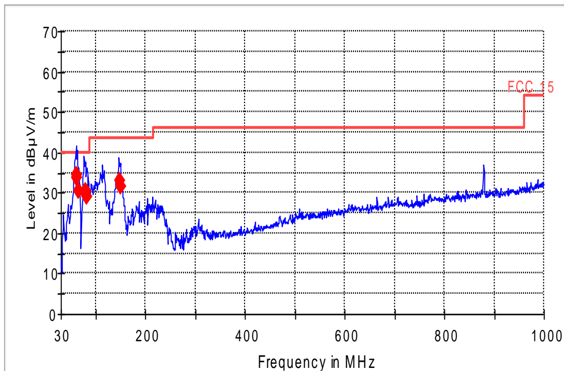
FCC 15 30-1000MHz
