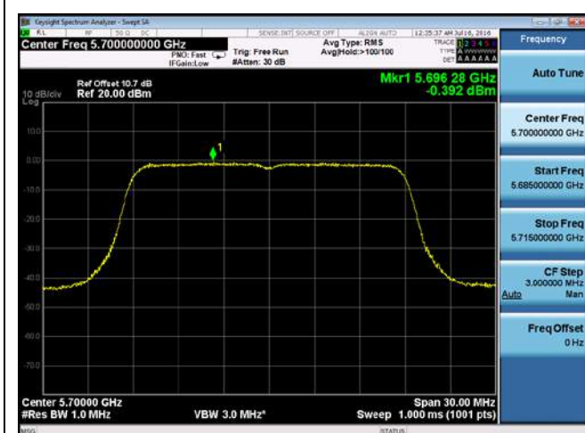
PSD-802.11n-20M-5700M-chain3
