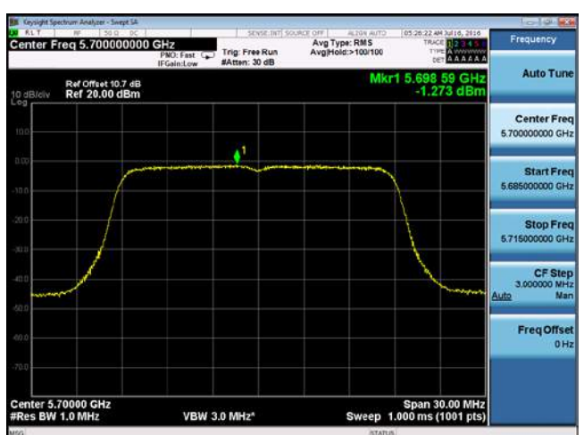
PSD-802.11n-20M-5700M-chain4
