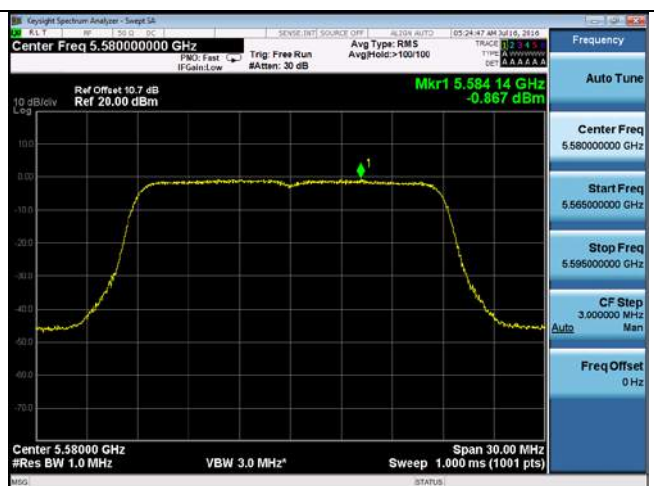
PSD-802.11n-20M-5580M-chain4
