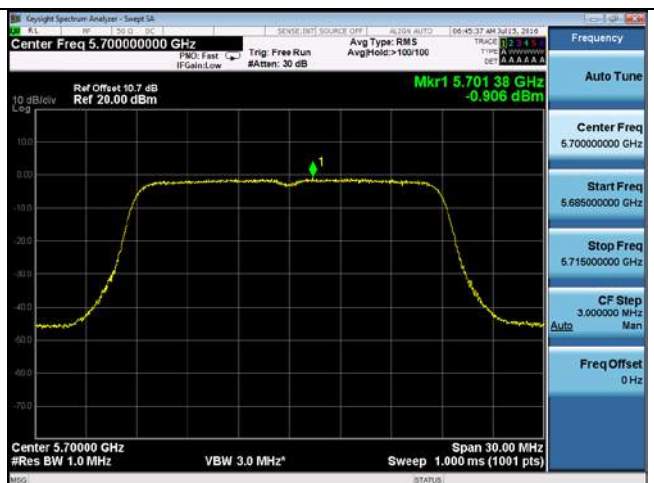
PSD-802.11n-20M-5700M-chain2
