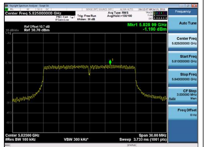
PSD-802.11n-20M-5825M-chain4
