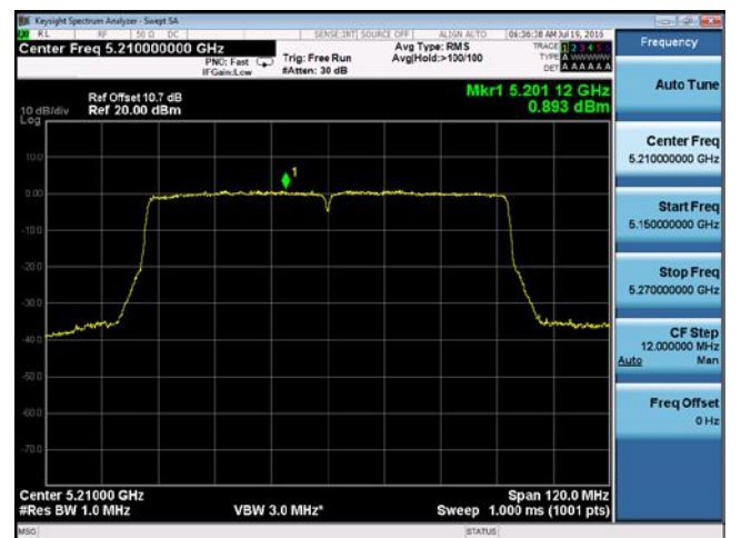
PSD-802.11ac-80M-5210M-chain4
