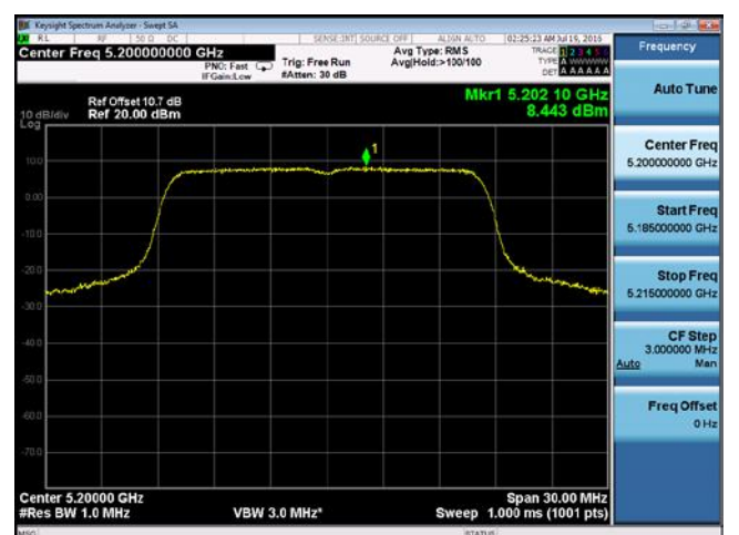
PSD-802.11a-5200M-chain2
