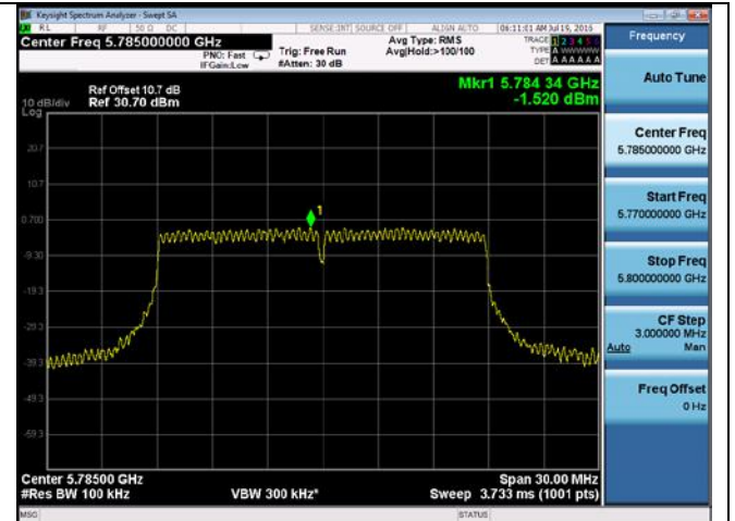
PSD-802.11n-20M-5785M-chain4
