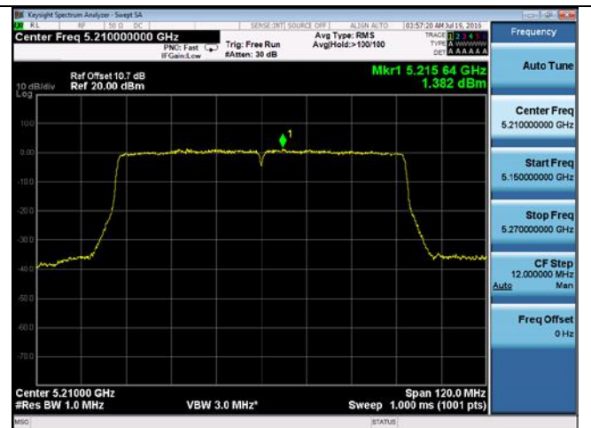
PSD-802.11ac-80M-5210M-chain2
