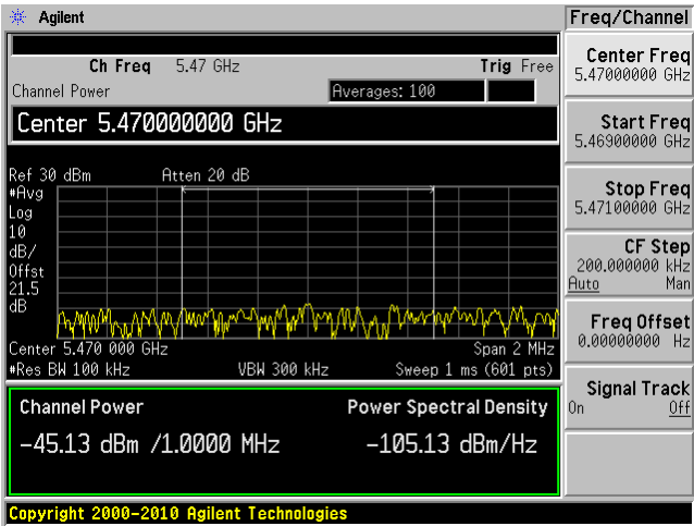
802.11 n 40, Chain 2 Low Band Edge
