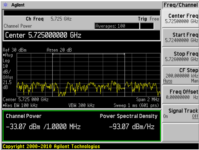
802.11 n 40, Chain 2 High Band Edge
