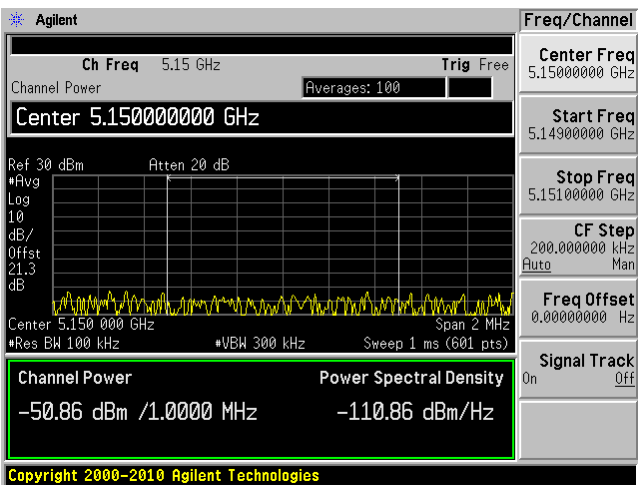
802.11 n 40, Chain 1 Low Band Edge
