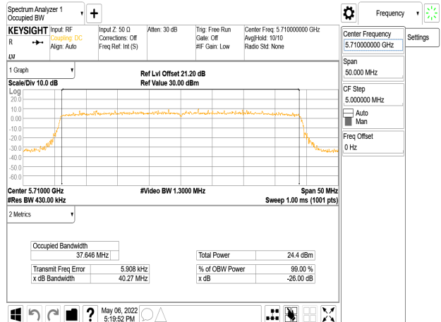
802.11ax_40MHz_Chain2_5710MHz
