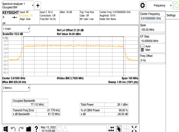
802.11ax_80MHz_Chain3_5610MHz
