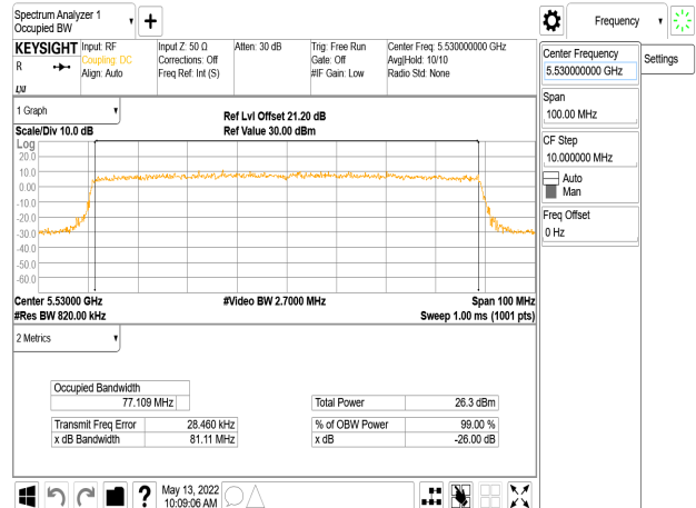
802.11ax_80MHz_Chain1_5530MHz
