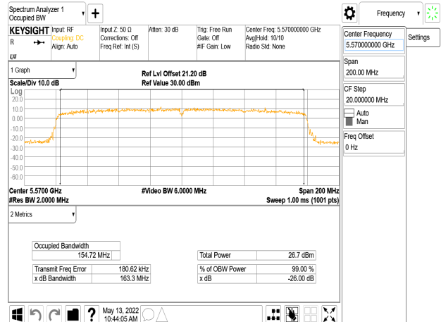
802.11ax_160MHz_Chain3_5570MHz
