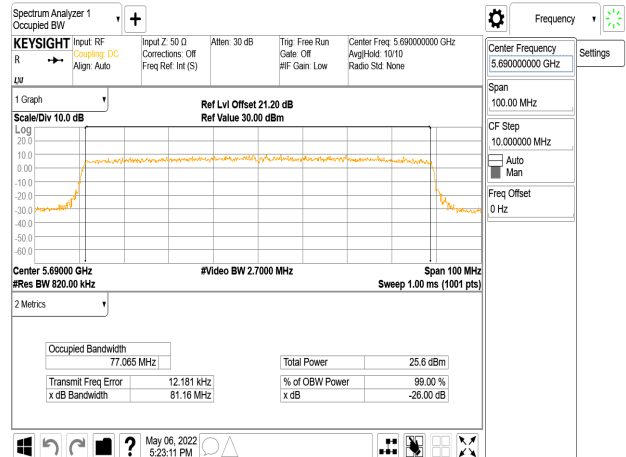
802.11ax_80MHz_Chain2_5690MHz
