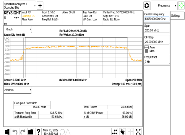
802.11ax_160MHz_Chain0_5570MHz
