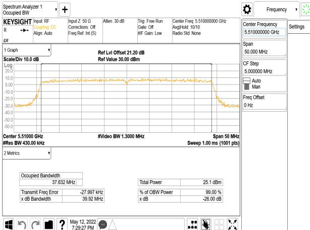
802.11ax_40MHz_Chain3_5510MHz
