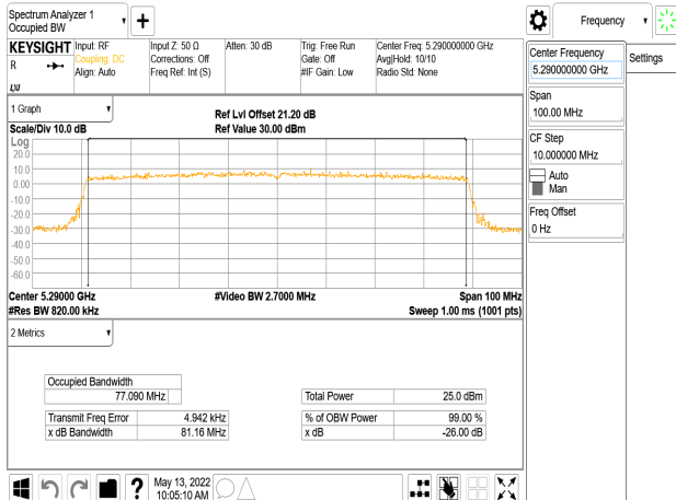
802.11ax_80MHz_Chain2_5290MHz
