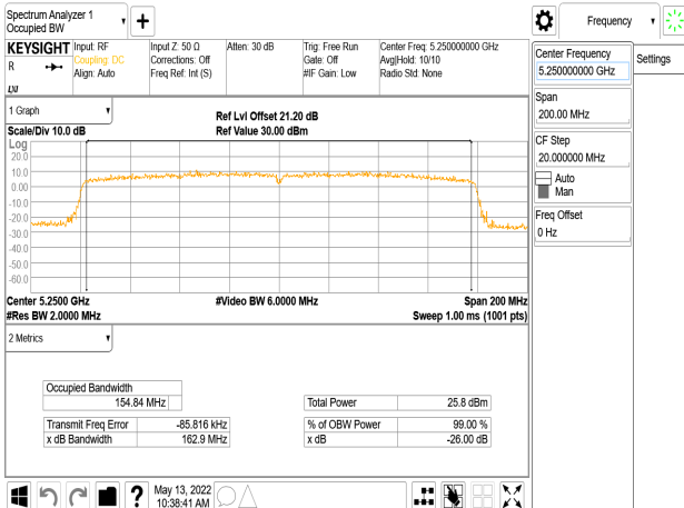
802.11ax_160MHz_Chain2_5250MHz
