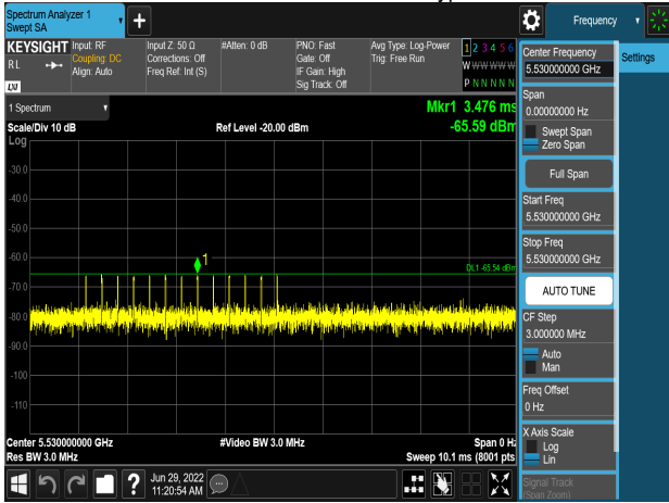
HE80_5530MHz_Radar_Type 4
