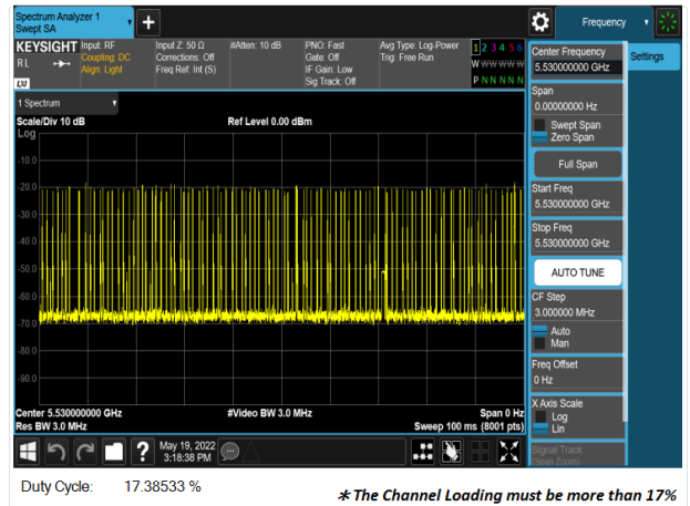
HE80_5530MHz
