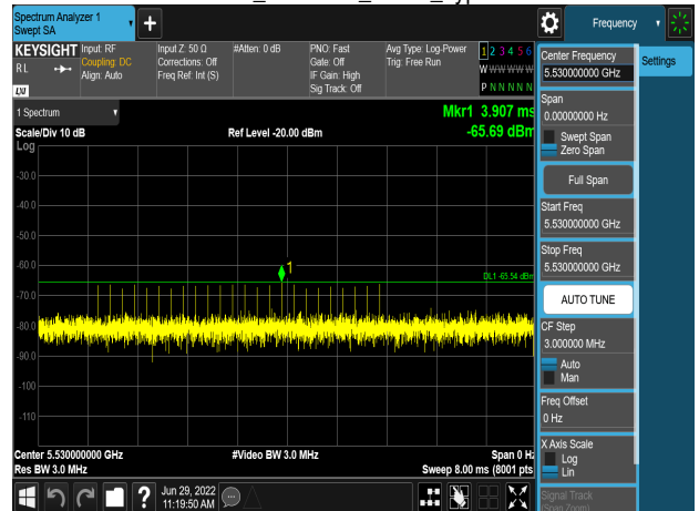
HE80_5530MHz_Radar_Type 2
