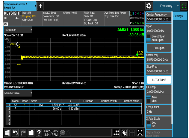
HE160_5570MHz
