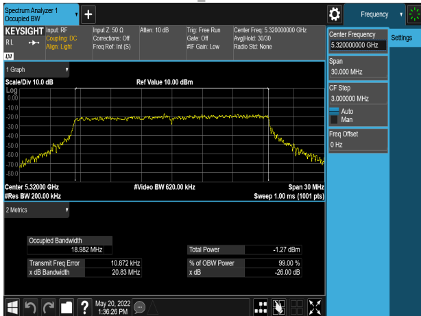
HE20_5320MHz
