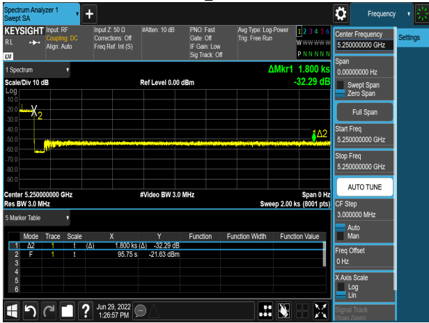
HE160_5250MHz
