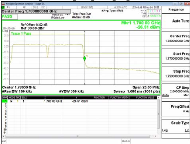
Band66B_10MHz+10MHz_QPSK_RB1-0_1-0_CH132022-132121
