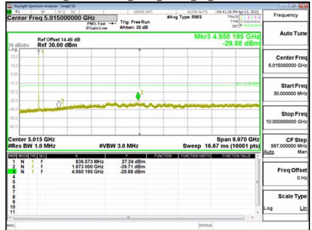
Band5_10MHz+10MHz_QPSK_RB1-49_1-0_CH20501-20600
