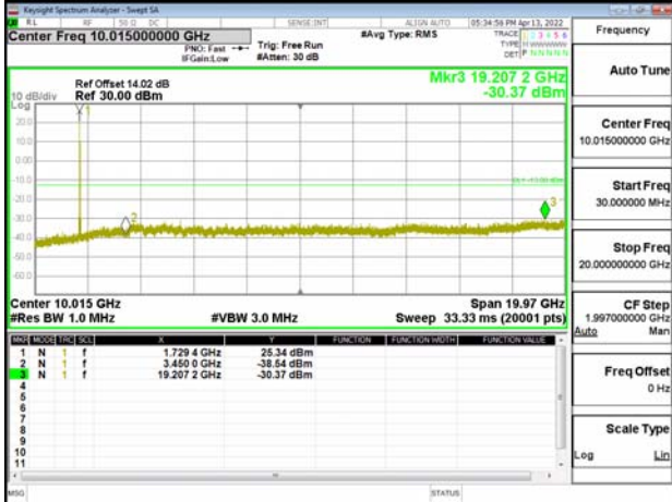
Band66_20MHz+10MHz_QPSK_RB1-99_1-0_CH132373-132517
