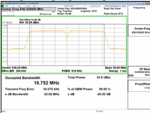
Band5_10MHz+10MHz_64QAM_RB50-0+RB50-0_CH20476+CH20575
