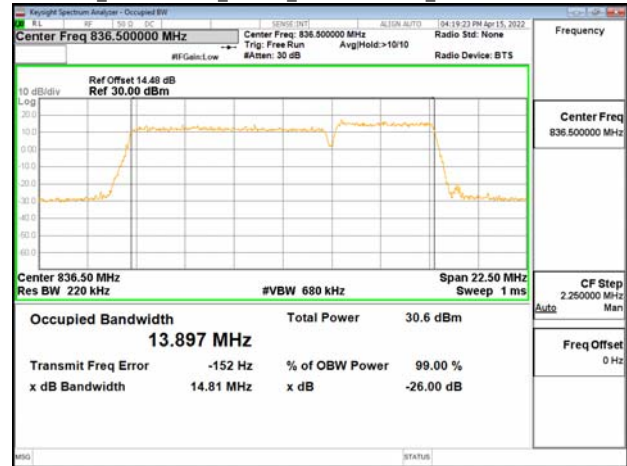
Band5_10MHz+5MHz_64QAM_RB50-0+RB25-0_CH20500+CH20572
