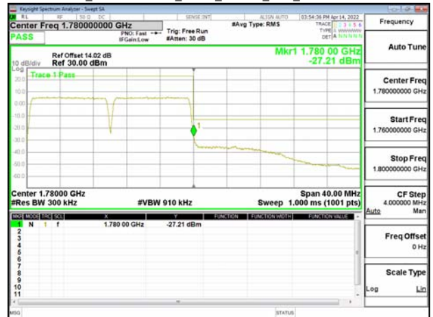
Band66B_10MHz+10MHz_QPSK_RB50-0_50-0_CH132523-132622
