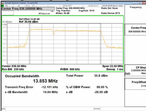
Band5_5MHz+10MHz_64QAM_RB25-0+RB50-0_CH20478+CH20550
