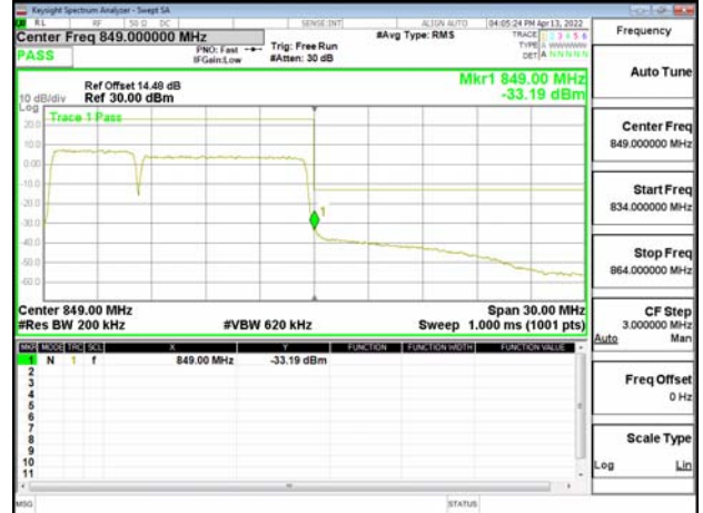
Band5_10MHz+10MHz_QPSK_RB1-0_1-0_CH20450-20549
