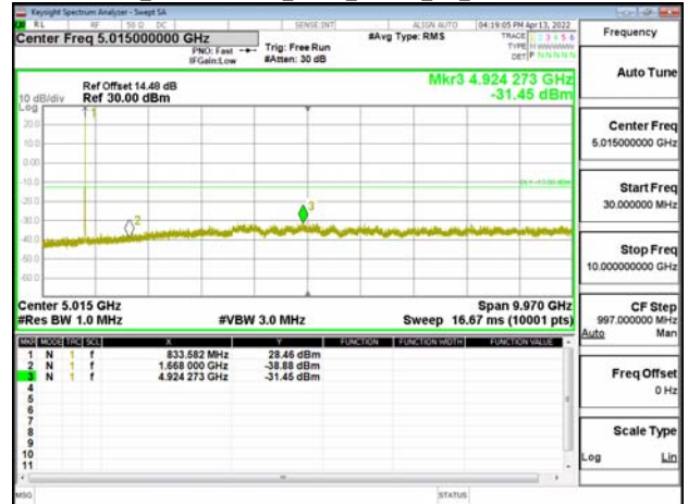
Band5_10MHz+10MHz_QPSK_RB1-49_1-0_CH20476-20575
