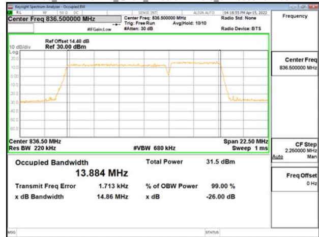
Band5_10MHz+5MHz_16QAM_RB50-0+RB25-0_CH20500+CH20572
