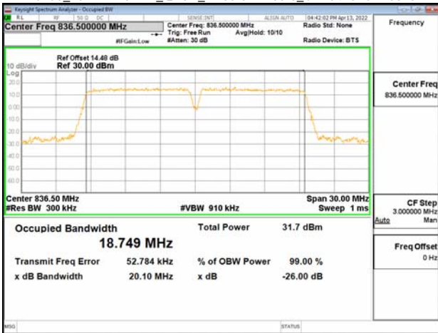
Band5_10MHz+10MHz_16QAM_RB50-0+RB50-0_CH20476+CH20575
