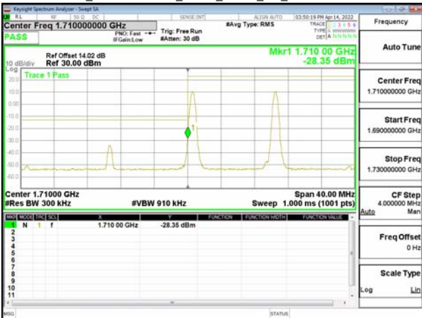
Band66B_10MHz+10MHz_QPSK_RB1-0_1-0_CH132022-132121
