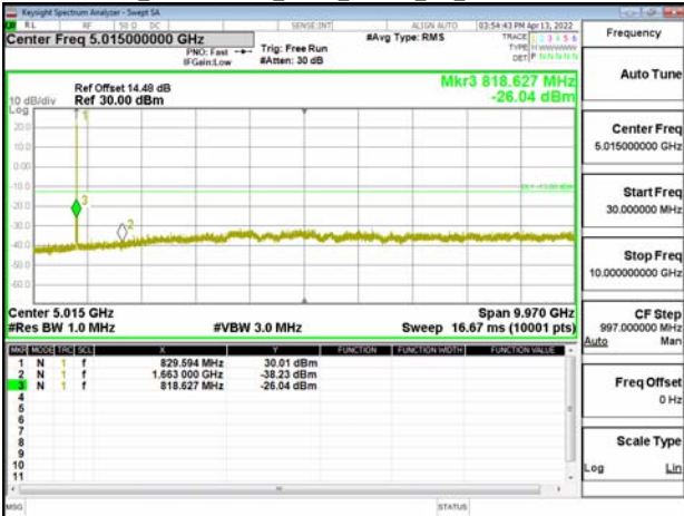
Band5_5MHz+10MHz_QPSK_RB1-24_1-0_CH20478-20550
