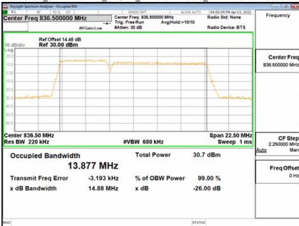
Band5_5MHz+10MHz_64QAM_RB25-0+RB50-0_CH20478+CH20550
