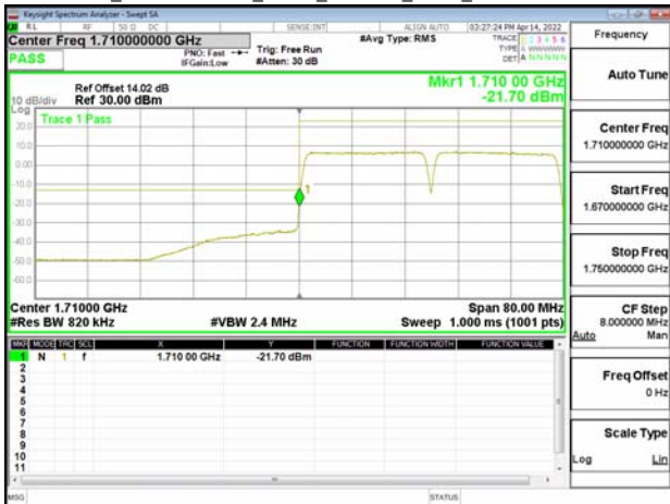
Band66_20MHz+20MHz_QPSK_RB100-0_100-0_CH132072-132270
