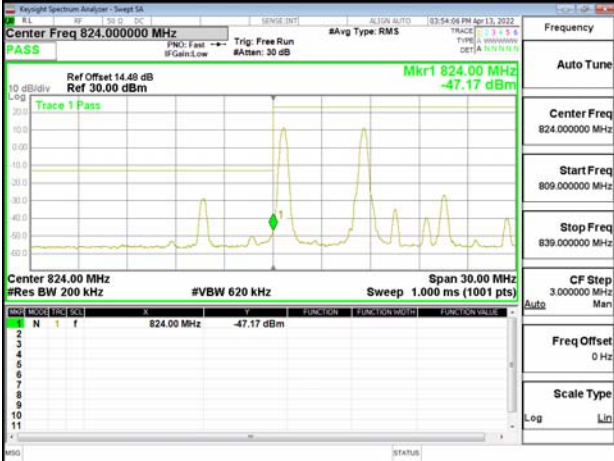
Band5_5MHz+10MHz_QPSK_RB1-24_1-49_CH20528-20600
