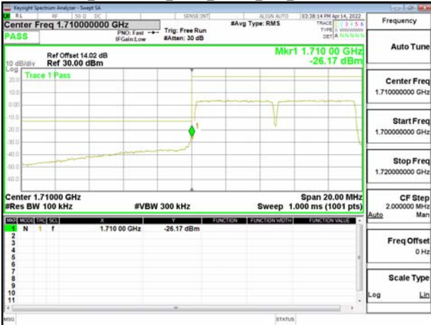
Band66B_5MHz+5MHz_QPSK_RB25-0_25-0_CH132599-132647
