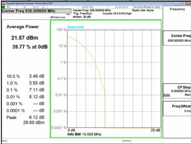
Band5_10MHz+10MHz_64QAM_RB50-0+RB50-0_CH20476+CH20575
