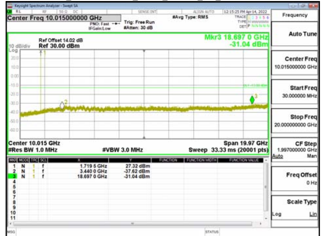
Band66B_10MHz+10MHz_OPSK_RB1-49_1-0_CH132373-132472
