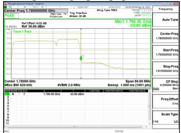
Band66_20MHz+10MHz_QPSK_RB100-0_50-0_CH132473-132617
