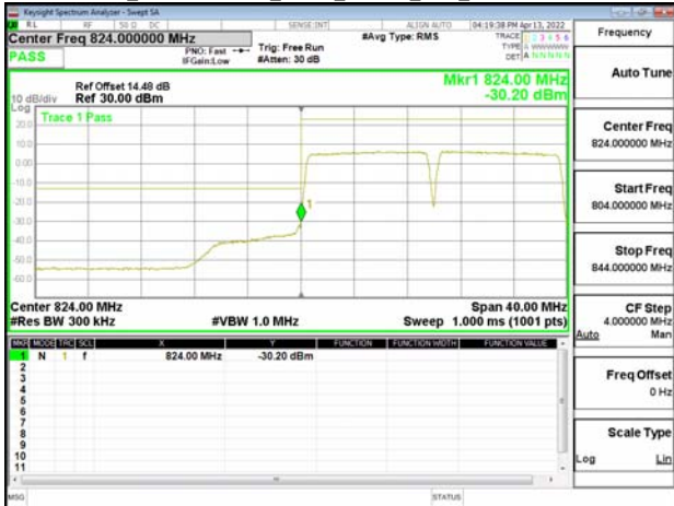
Band5_10MHz+10MHz_QPSK_RB50-0_50-0_CH20501-20600
