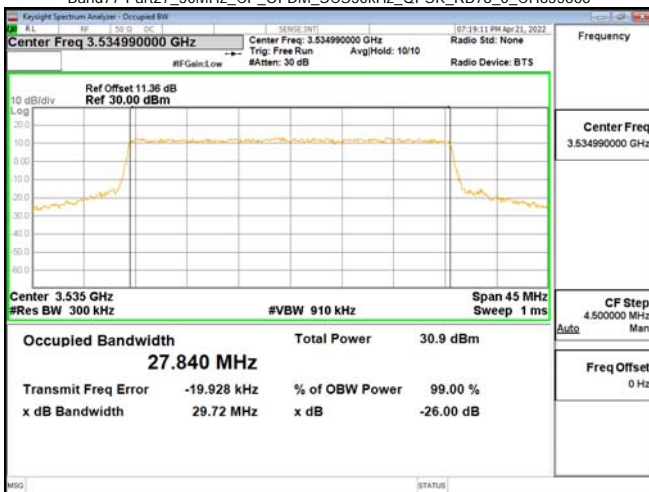
Band77-Part27_30MHz_CP_OFDM_SCS30kHz_QPSK_RB78_0_CH635666
