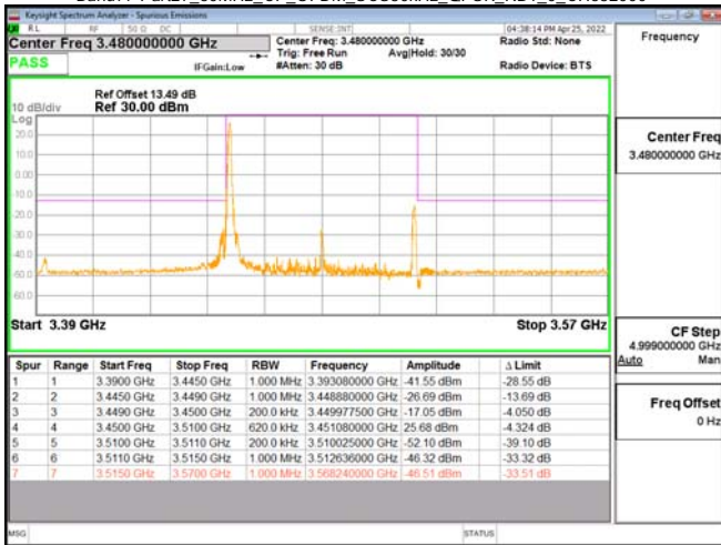
Band77-Part27_60MHz_CP_OFDM_SCS30kHz_OPSK_RB1_0_CH633334
