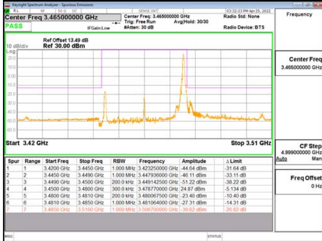
Band77-Part27_30MHz_CP_OFDM_SCS30kHz_QPSK_RB1_77_CH633334
