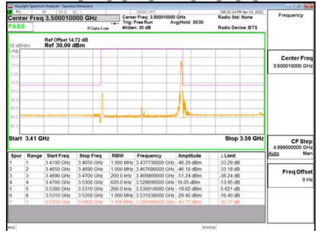
Band77-Part27_60MHz_CP_OFDM_SCS30kHz_OPSK_RB1_161_CH633334
