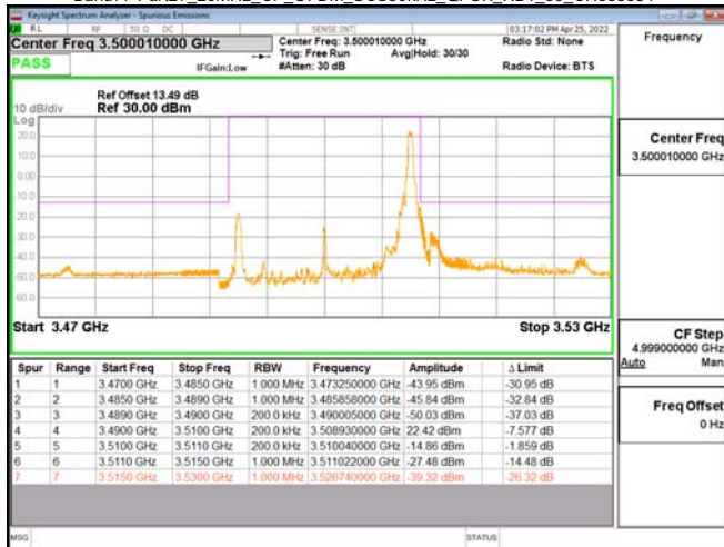
Band77-Part27_20MHz_CP_OFDM_SCS30kHz_OPSK_RB1_50_CH636000
