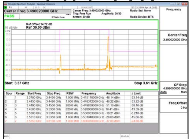
Band77-Part27_80MHz_CP_OFDM_SCS30kHz_OPSK_RB1_216_CH633334
