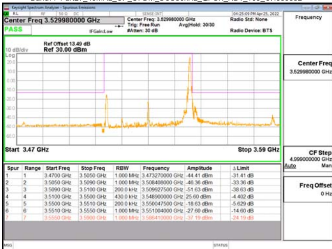
Band77-Part27_40MHz_CP_OFDM_SCS30kHz_OPK RB1_105_CH635332
