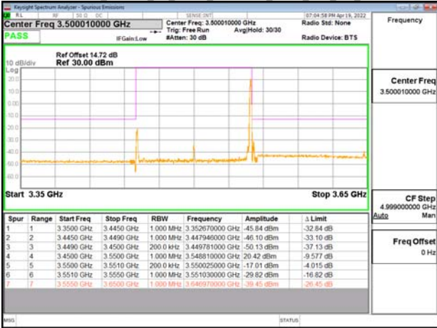
Band77-Part27_100MHz_CP_OFDM_SCS30kHz_OPK_RB1_272_CH633334
