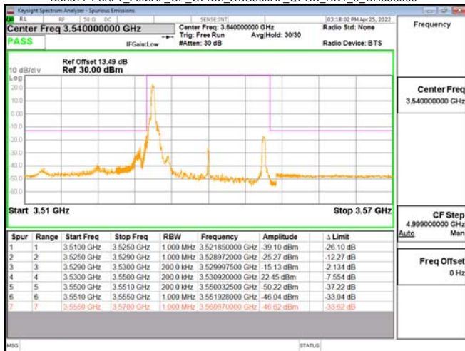
Band77-Part27_20MHz_CP_OFDM_SCS30kHz_QPSK_RB1_0_CH636000
