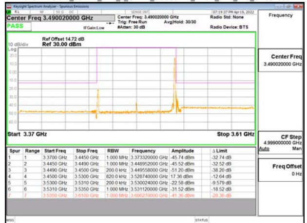
Band77-Part27_80MHz_DFT_s_OFDM_SCS30kHz_BPSK_RB1_216_CH633334
