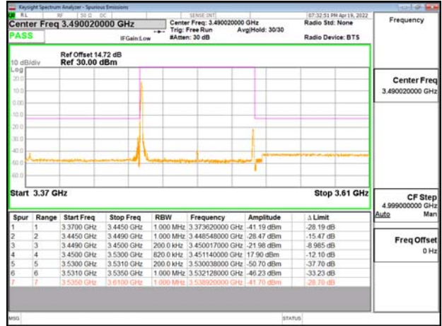
Band77-Part27_80MHz_CP_OFDM_SCS30kHz_QPSK_RB1_0_CH633334
