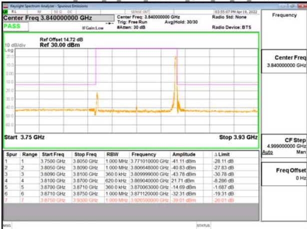
Band77-Part27_60MHz_CP_OFDM_SCS30kHz_OPSK_RB1_161_CH656000
