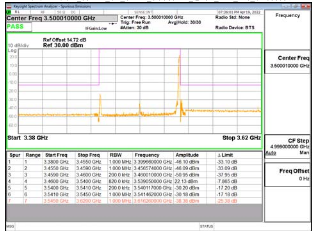
Band77-Part27_80MHz_CP_OFDM_SCS30kHz_OPSK_RB1_216_CH633334
