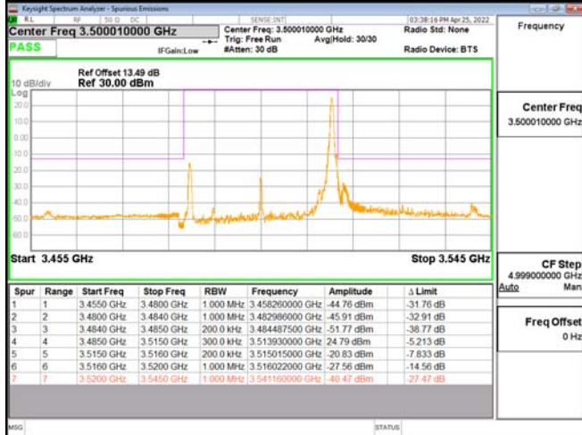
Band77-Part27_30MHz_CP_OFDM_SCS30kHz_QPSK_RB1_77_CH635666
