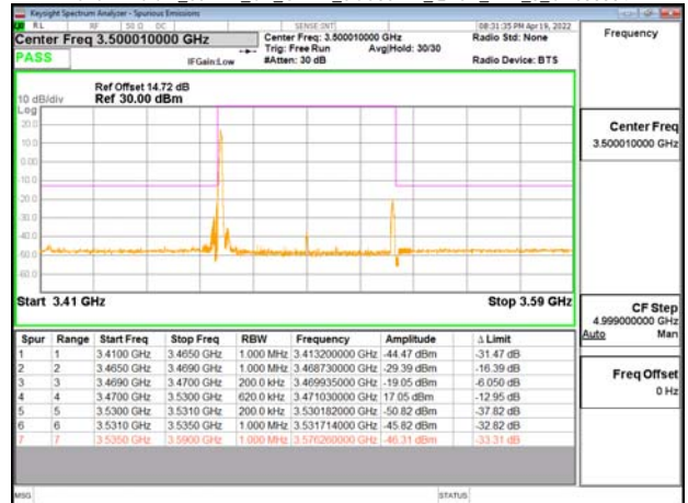
Band77-Part27_60MHz_CP_OFDM_SCS30kHz_OPSK_RB1_0_CH633334
