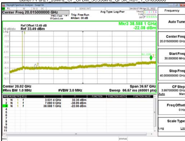
Band77-Part27_20MHz_CP_OFDM_SCS30kHz_QPSK_RB1_1_CH636000
