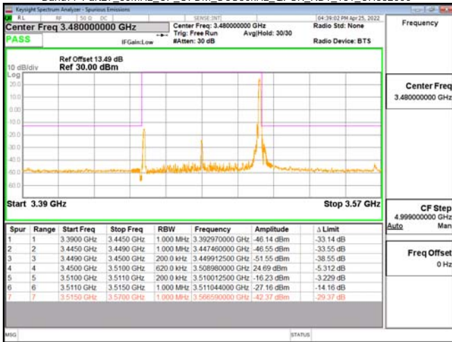
Band77-Part27_60MHz_CP_OFDM_SCS30kHz_OPK RB1_161_CH633334
