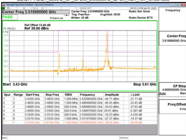
Band77-Part27_60MHz_CP_OFDM_SCS30kHz_OPK RB1_161_CH634666
