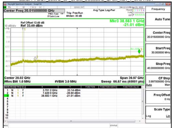
Band77-Part27_20MHz_CP_OFDM_SCS30kHz_QPSK_RB1_1_CH656000
