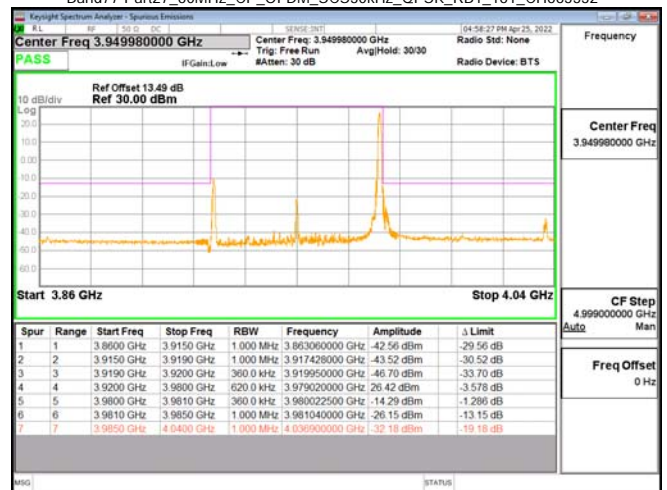
Band77-Part27_60MHz_CP_OFDM_SCS30kHz_OPK RB1_161_CH663332
