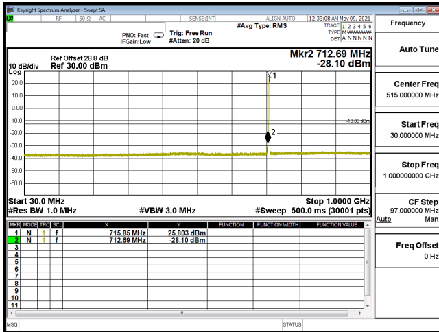
CSE-B12_3M-CH23165-QPSK(1,14)-30M-1G
