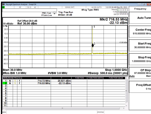
CSE-B12_3M-CH23165-16QAM(1,7)-30M-1G
