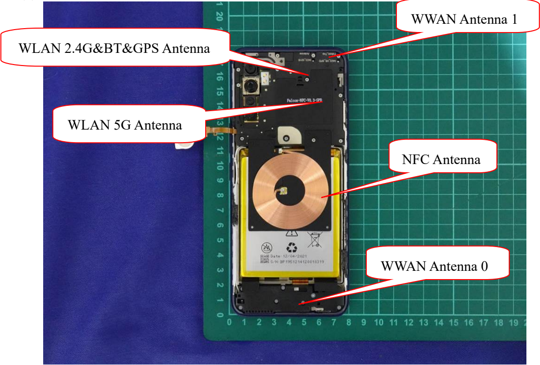
(2) EUT Photo
