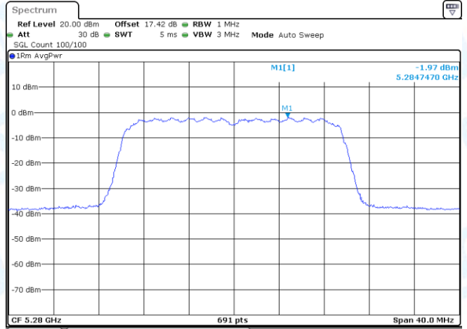
11AX20MIMO-Ant1-5280-PASS
