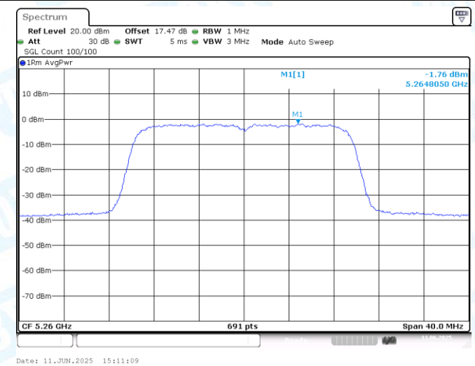
11AX20MIMO-Ant1-5260-PASS
