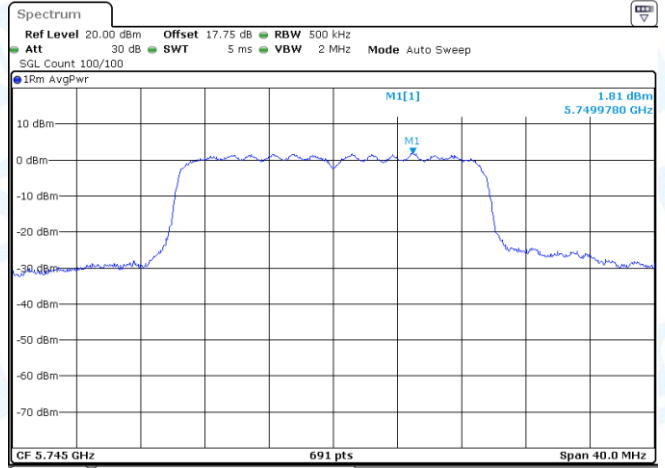
11AX20MIMO-Ant1-5745-PASS
