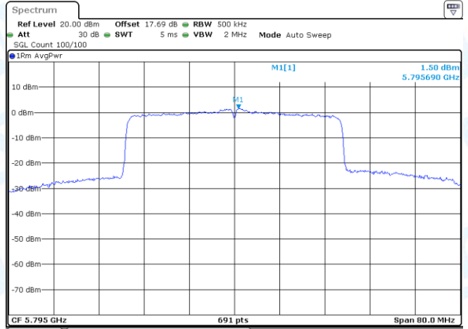
11AX40MIMO-Ant1-5795-PASS
