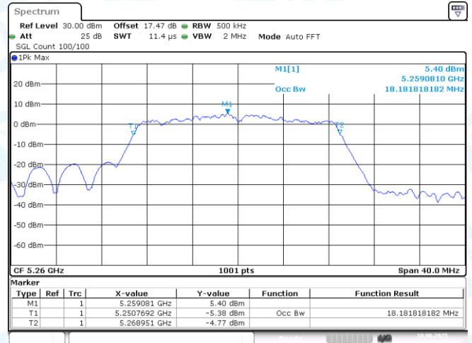
11N20MIMO-Ant1-5260
