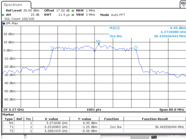
11N40MIMO-Ant2-5270
