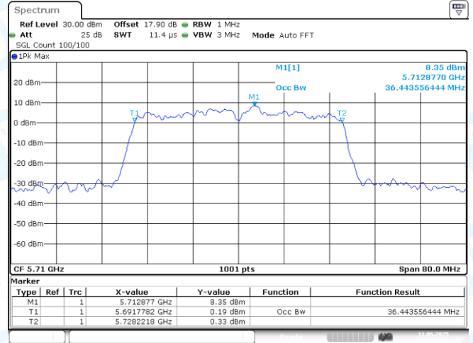
11N40MIMO-Ant1-5710
