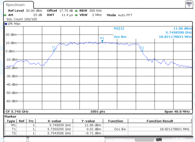
11N20MIMO-Ant1-5745
