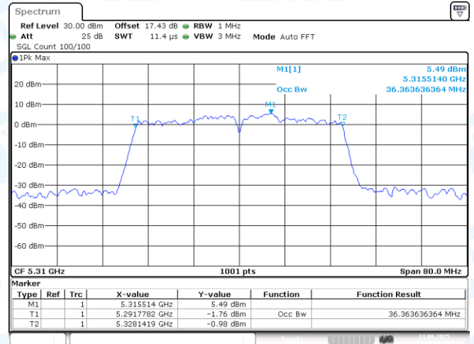
11N40MIMO-Ant1-5310
