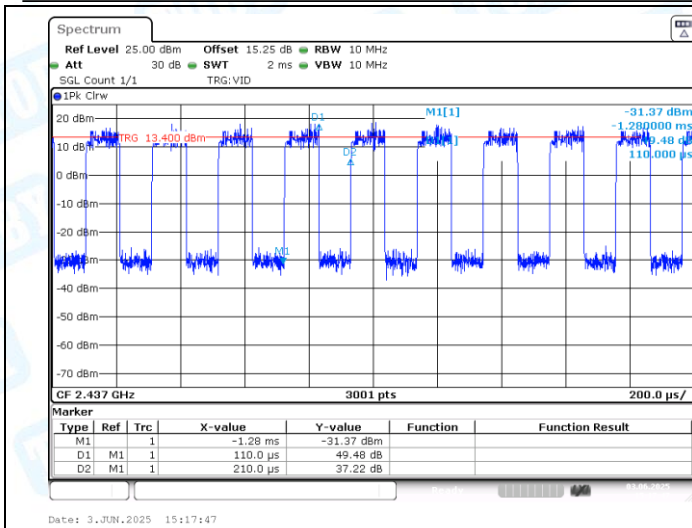
NTNV-11AX20MIMO-Ant2-2437
