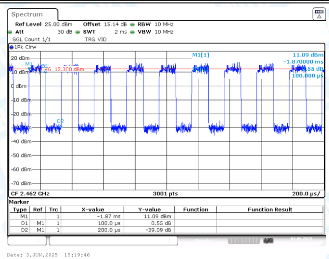
NTNV-11AX20MIMO-Ant1-2462
