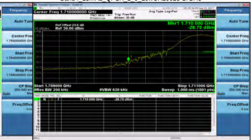
Band4 15MHz QPSK 1 0 LowCH20025-1717.5
