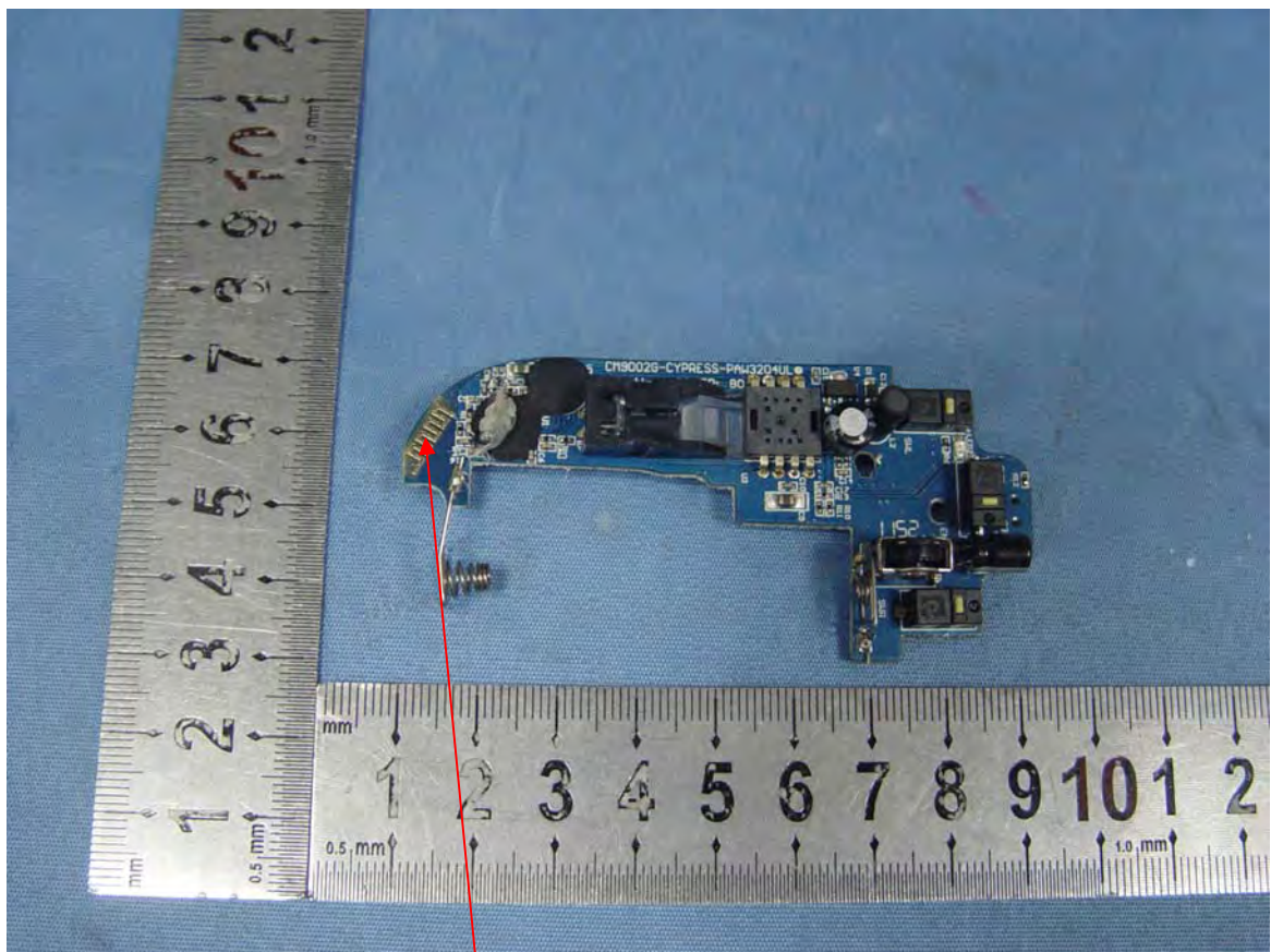
Antenna
