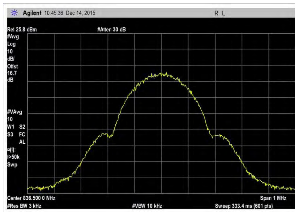
7.10_OBW_UL_824-849MHz_GSM
