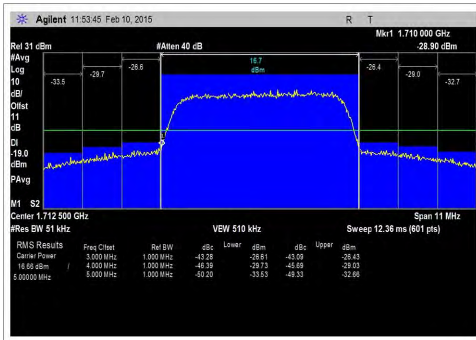
7.5_OBE_UL_1710-1755MHz_LTE_L_-26dBm
