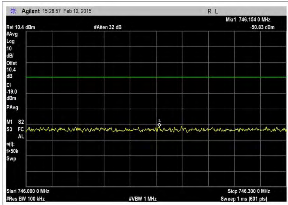
7.5_OBE_DL_728-746MHz_CDMA_H_-56dBm
