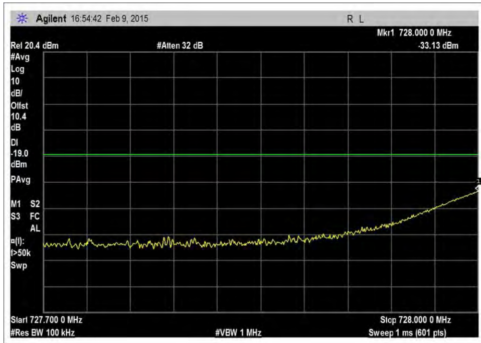
7.5_OBE_DL_728-746MHz_GSM_L_-46dBm
