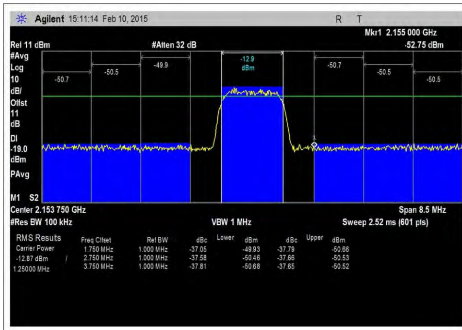
7.5_OBE_DL_2110-2155MHz_CDMA_H_-48dBm
