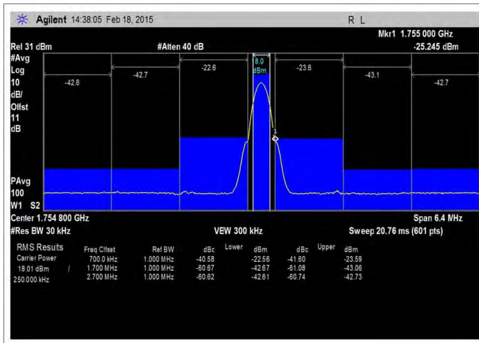
7.5_OBE_UL_1710-1755MHz_GSM_H_-21dBm
