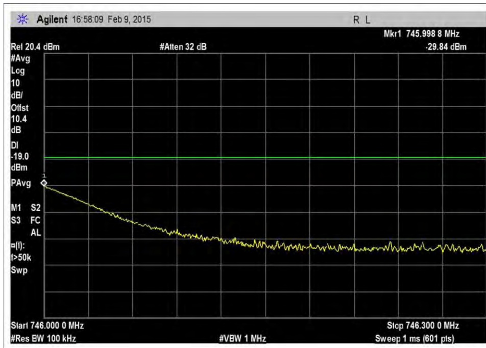
7.5_OBE_DL_728-746MHz_GSM_H_-48dBm
