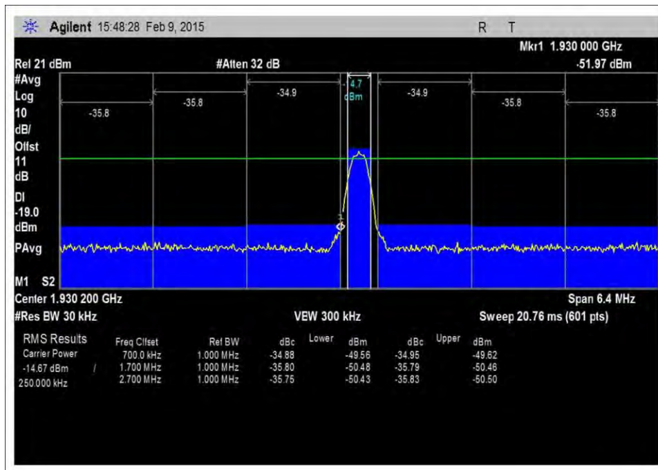
7.5_OBE_DL_1930-1995MHz_GSM_L_-47dBm
