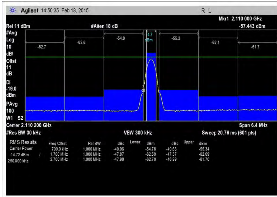
7.5_OBE_DL_2110-2155MHz_GSM_L_-52dBm
