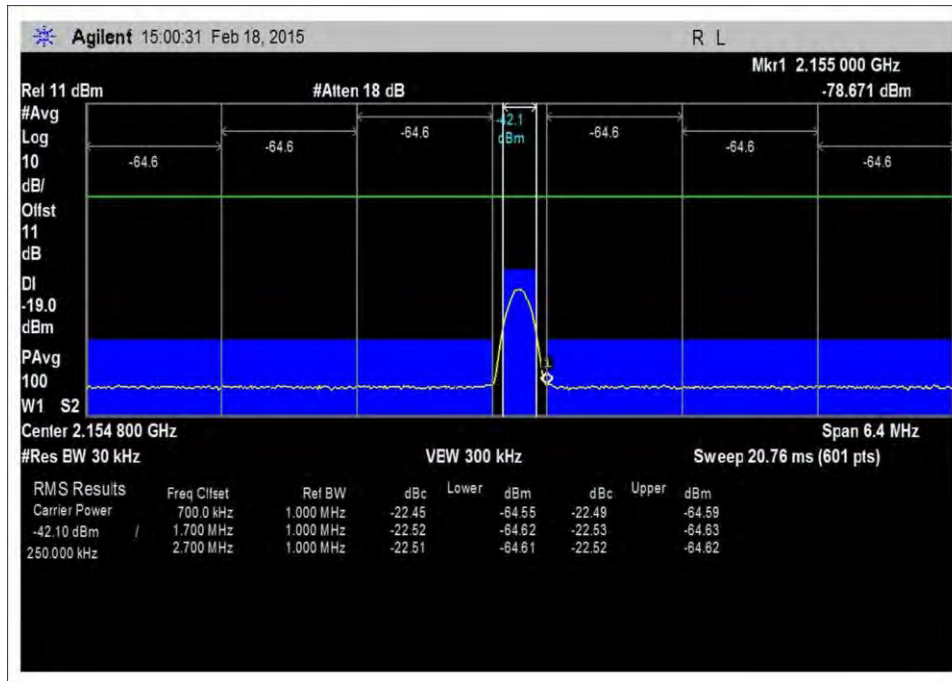
7.5_OBE_DL_2110-2155MHz_GSM_H_-20dBm
