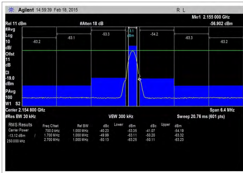
7.5_OBE_DL_2110-2155MHz_GSM_H_-48dBm
