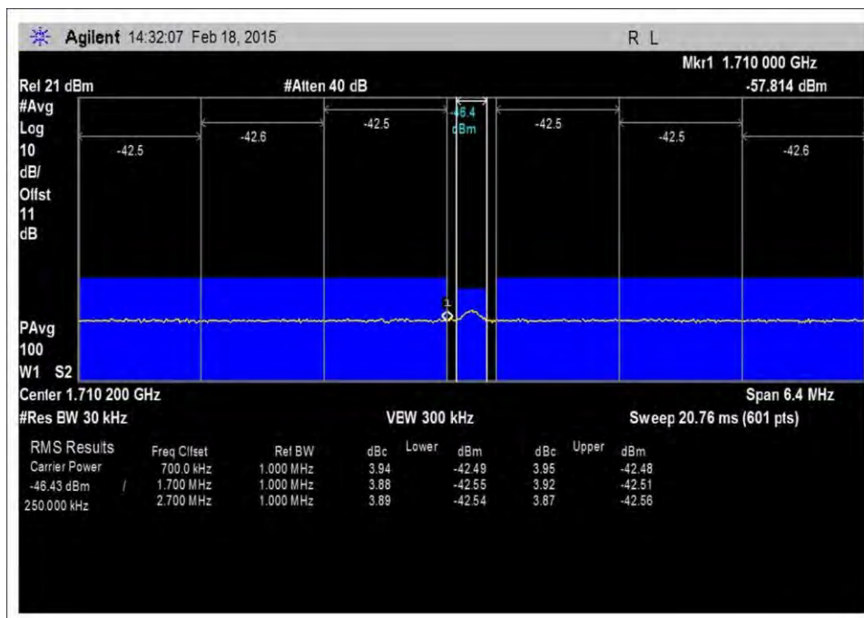
7.5_OBE_UL_1710-1755MHz_GSM_L_+10dBm
