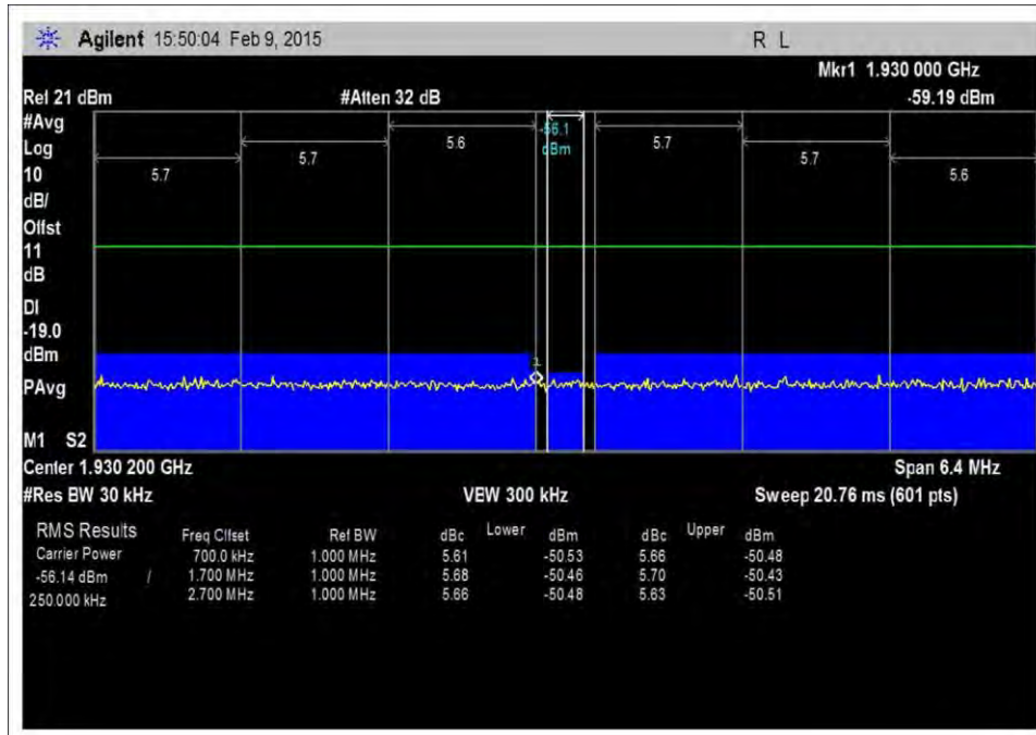
7.5_OBE_DL_1930-1995MHz_GSM_L_-20dBm
