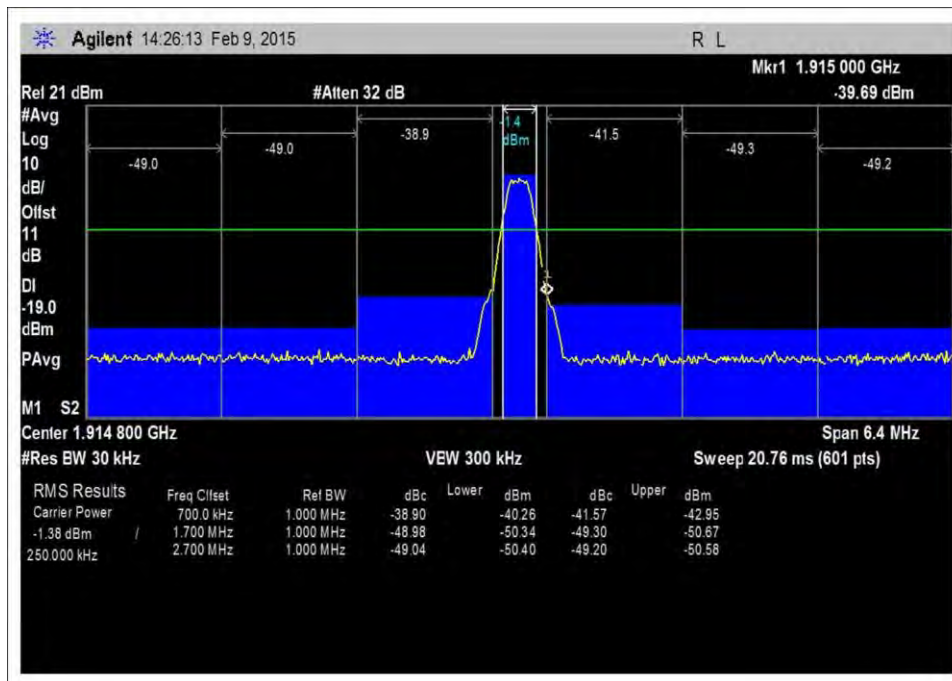
7.5_OBE_UL_1850-1915MHz_GSM_H_26
