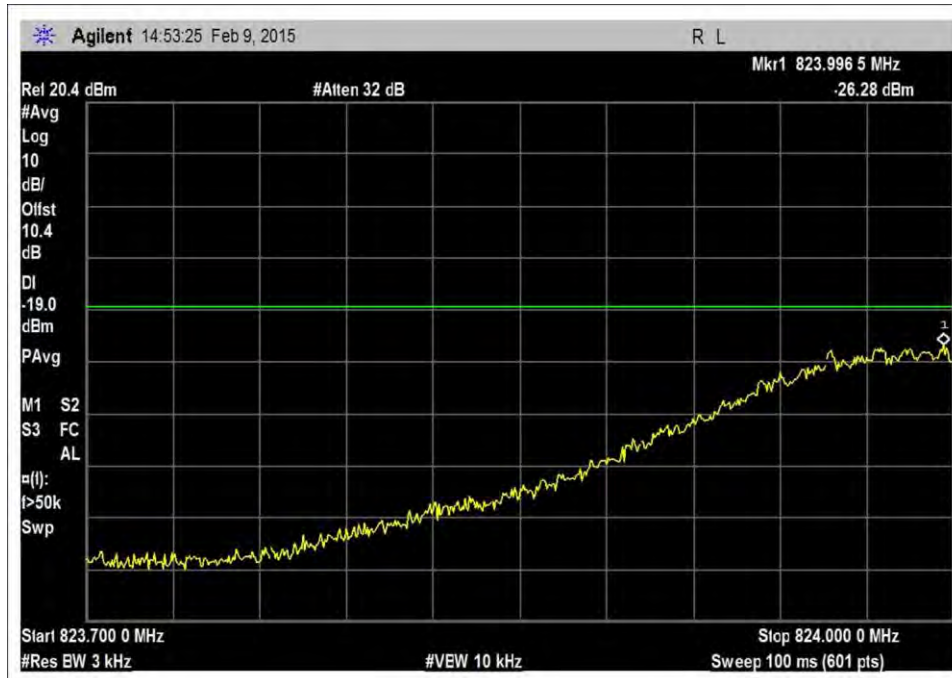
7.5_OBE_UL_824-849MHz_GSM_L_-26dBm
