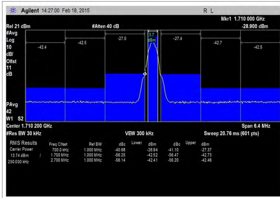
7.5_OBE_UL_1710-1755MHz_GSM_L_-27dBm
