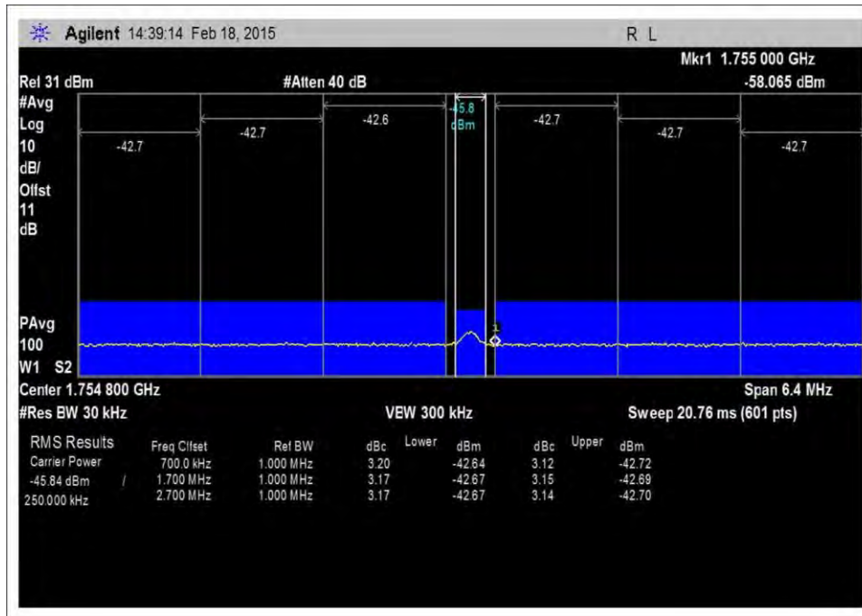
7.5_OBE_UL_1710-1755MHz_GSM_H_+10dBm
