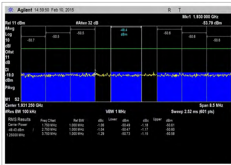
7.5_OBE_DL_1930-1995MHz_CDMA_L_-20dBm
