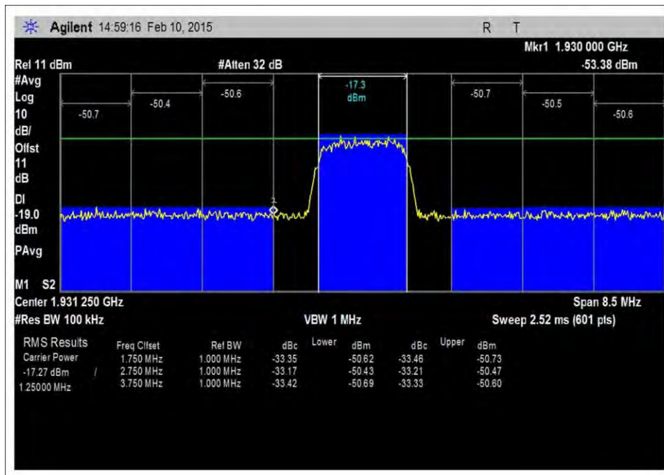
7.5_OBE_DL_1930-1995MHz_CDMA_L_-47dBm
