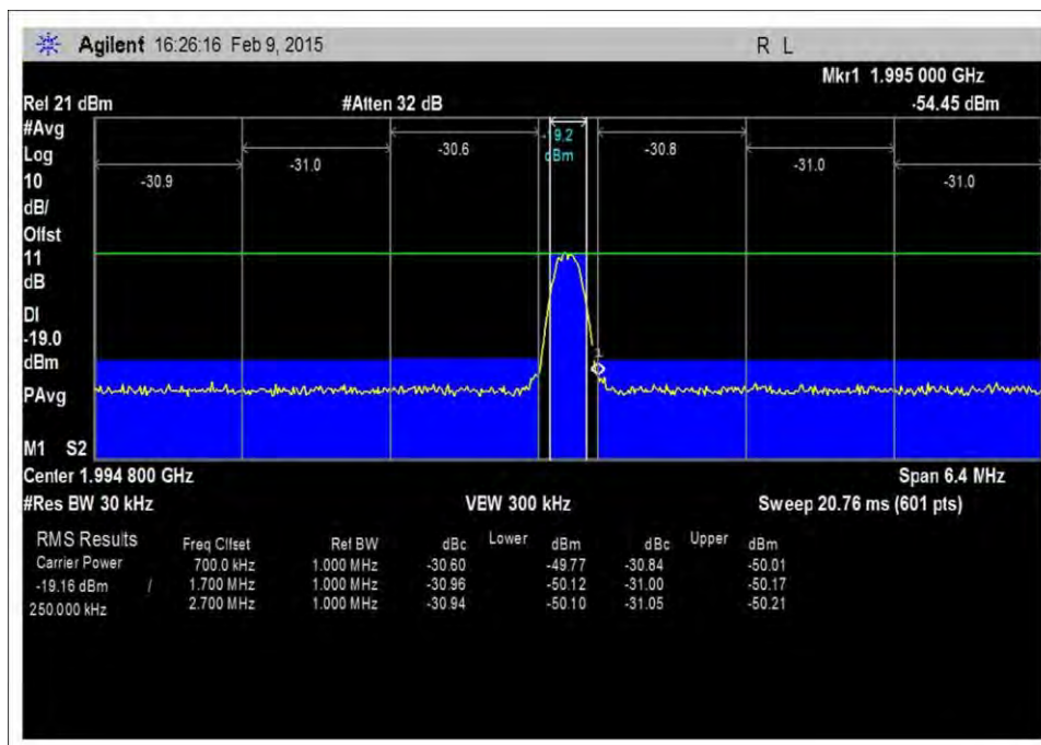
7.5_OBE_DL_1930-1995MHz_GSM_H_-46dBm
