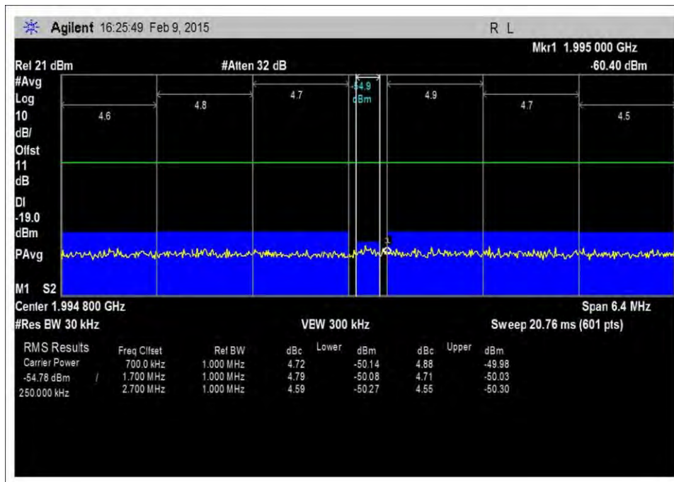
7.5_OBE_DL_1930-1995MHz_GSM_H_-20dBm
