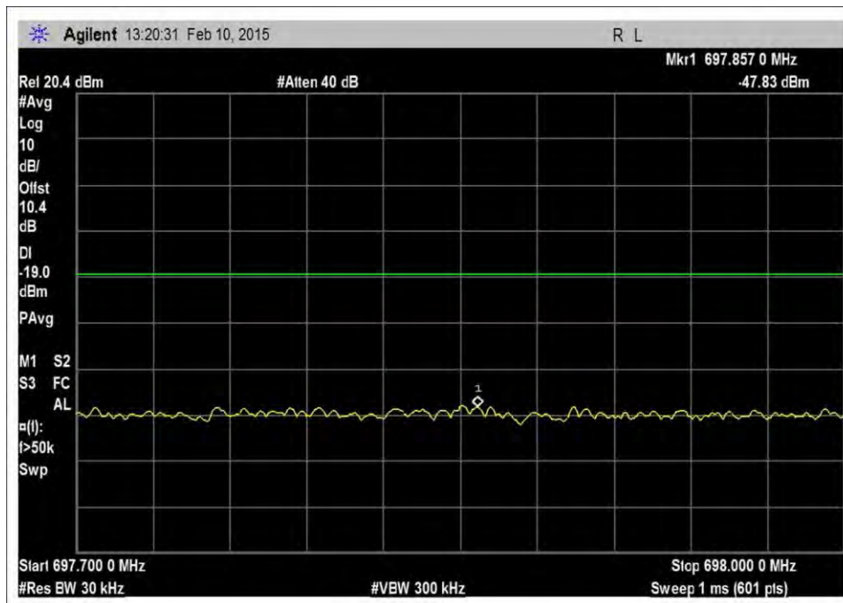
7.5_OBE_UL_698-716MHz_LTE_L_+10dBm
