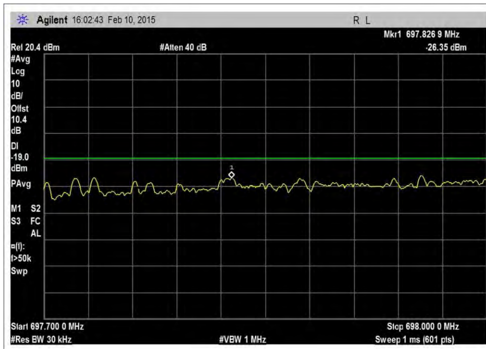
7.5_OBE_UL_698-716MHz_CDMA_L_-21dBm
