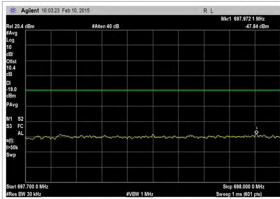
7.5_OBE_UL_698-716MHz_CDMA_L_+10dBm
