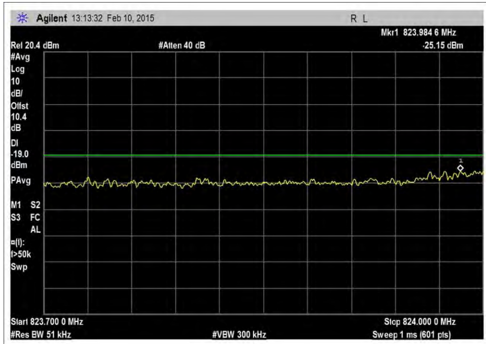
7.5_OBE_UL_824-849MHz_LTE_L_-26dBm
