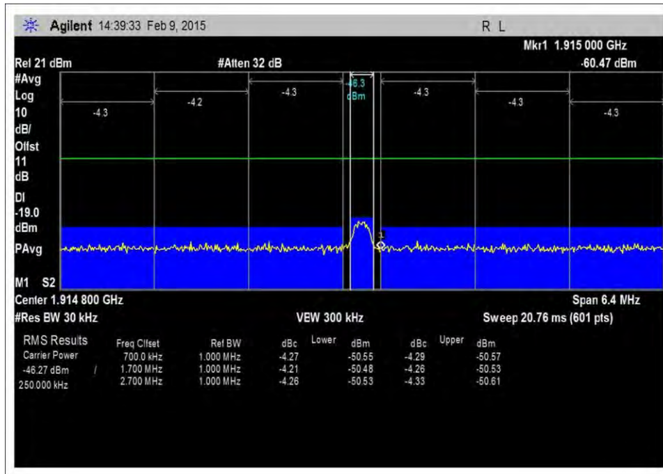
7.5_OBE_UL_1850-1915MHz_GSM_H_+10dBm
