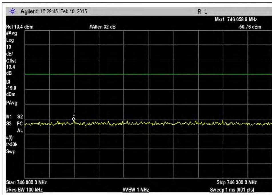
7.5_OBE_DL_728-746MHz_CDMA_H_-48dBm
