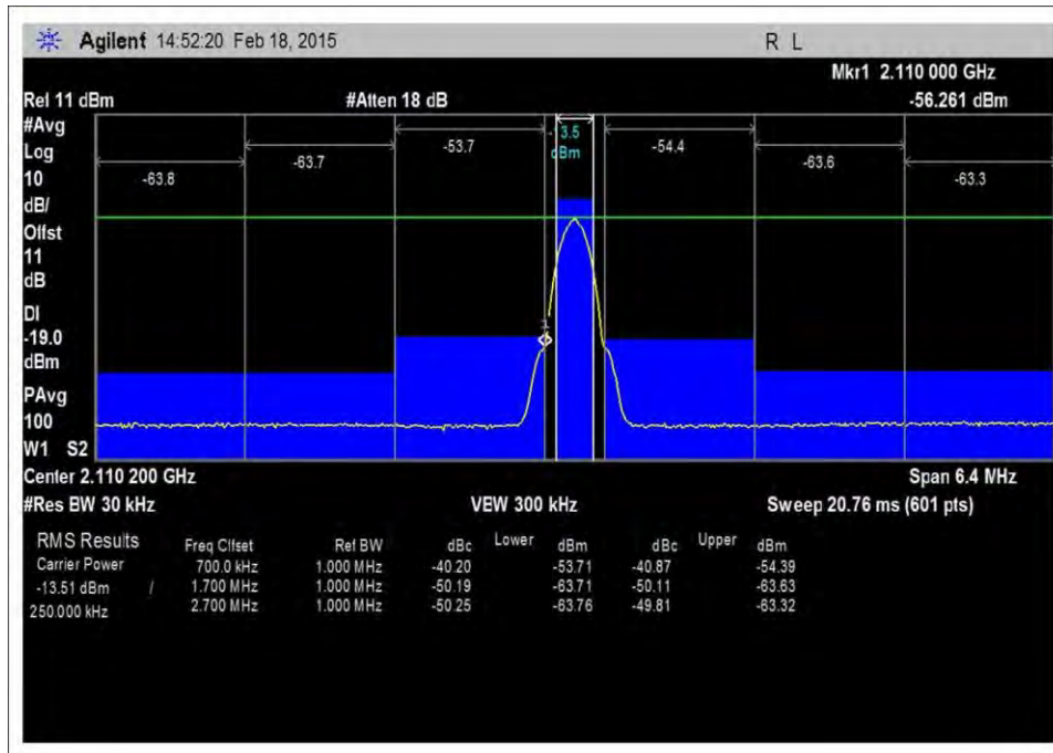
7.5_OBE_DL_2110-2155MHz_GSM_L_-46dBm
