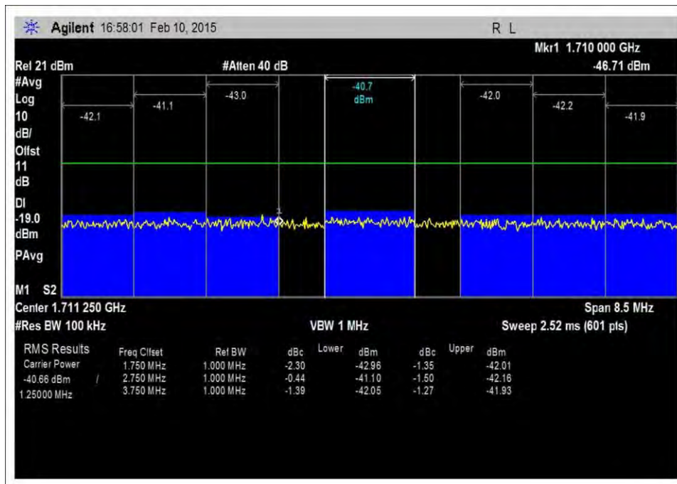
7.5_OBE_UL_1710-1755MHz_CDMA_L_+10dBm
