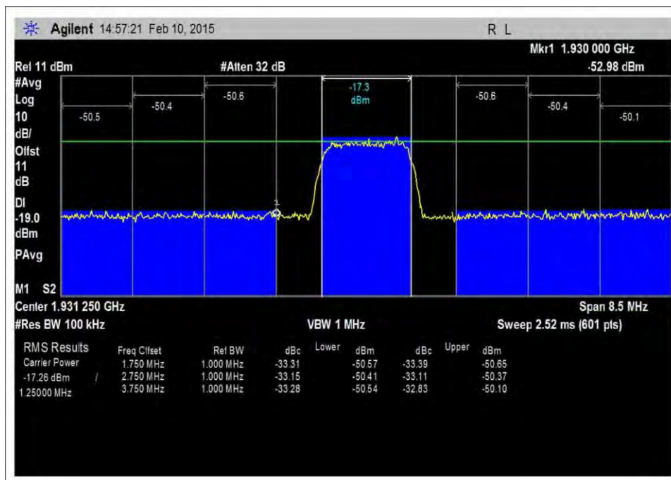
7.5_OBE_DL_1930-1995MHz_CDMA_L_-52dBm
