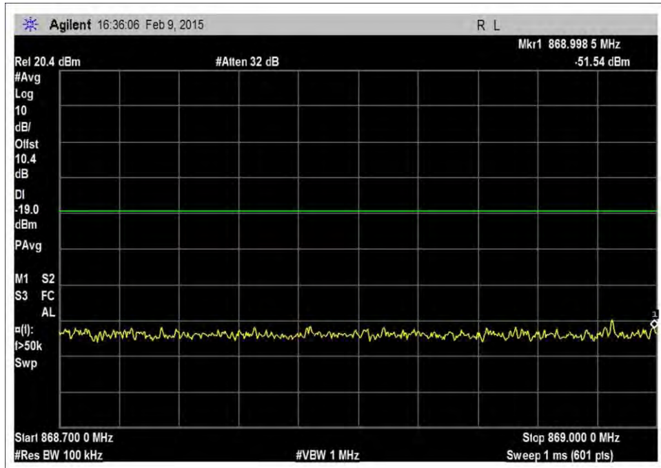
7.5_OBE_DL_869-894MHz_GSM_L_-20dBm
