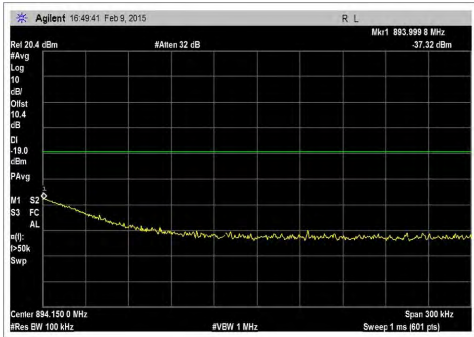
7.5_OBE_DL_869-894MHz_GSM_H_-56dBm
