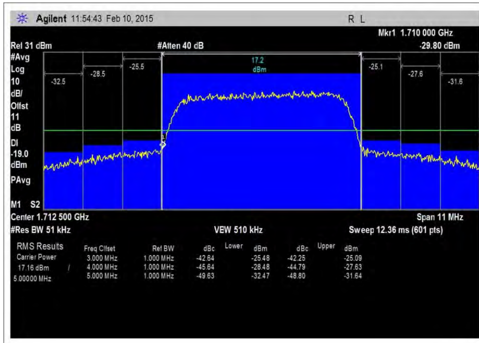
7.5_OBE_UL_1710-1755MHz_LTE_L_-20dBm
