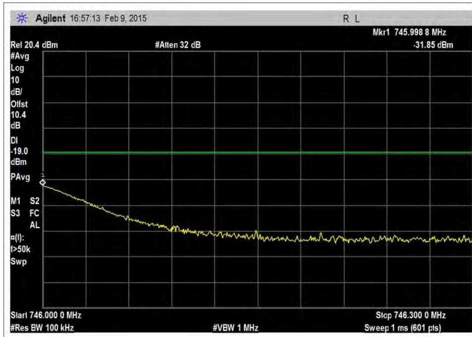
7.5_OBE_DL_728-746MHz_GSM_H_-54dBm
