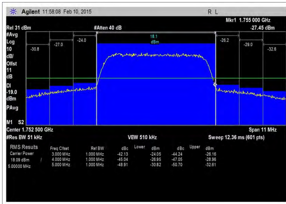
7.5_OBE_UL_1710-1755MHz_LTE_H_-24dBm
