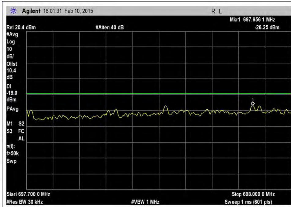
7.5_OBE_UL_698-716MHz_CDMA_L_-26dBm
