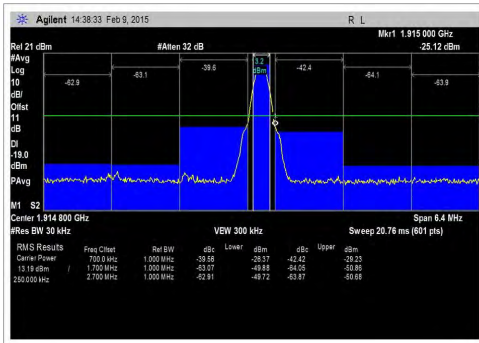
7.5_OBE_UL_1850-1915MHz_GSM_H_-5dBm
