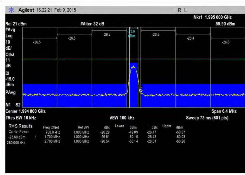
7.5_OBE_DL_1930-1995MHz_GSM_H_-55dBm
