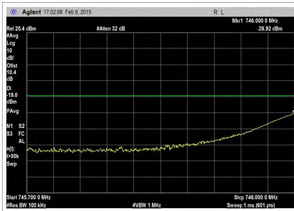
7.5_OBE_DL_746-757MHz_GSM_L_-48dBm
