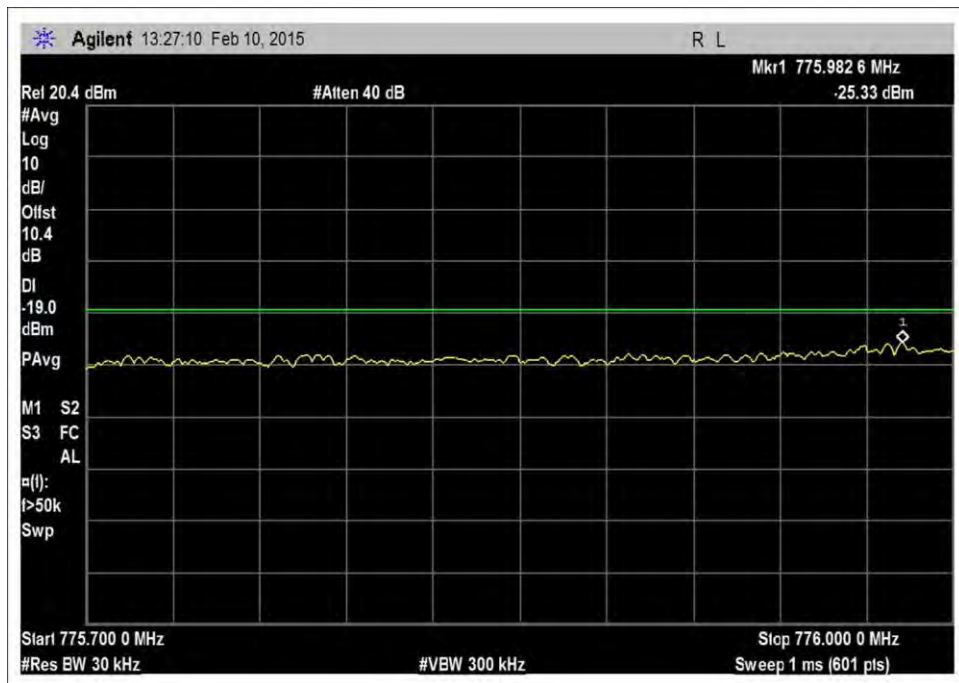
7.5_OBE_UL_776-787MHz_LTE_L_-26dBm
