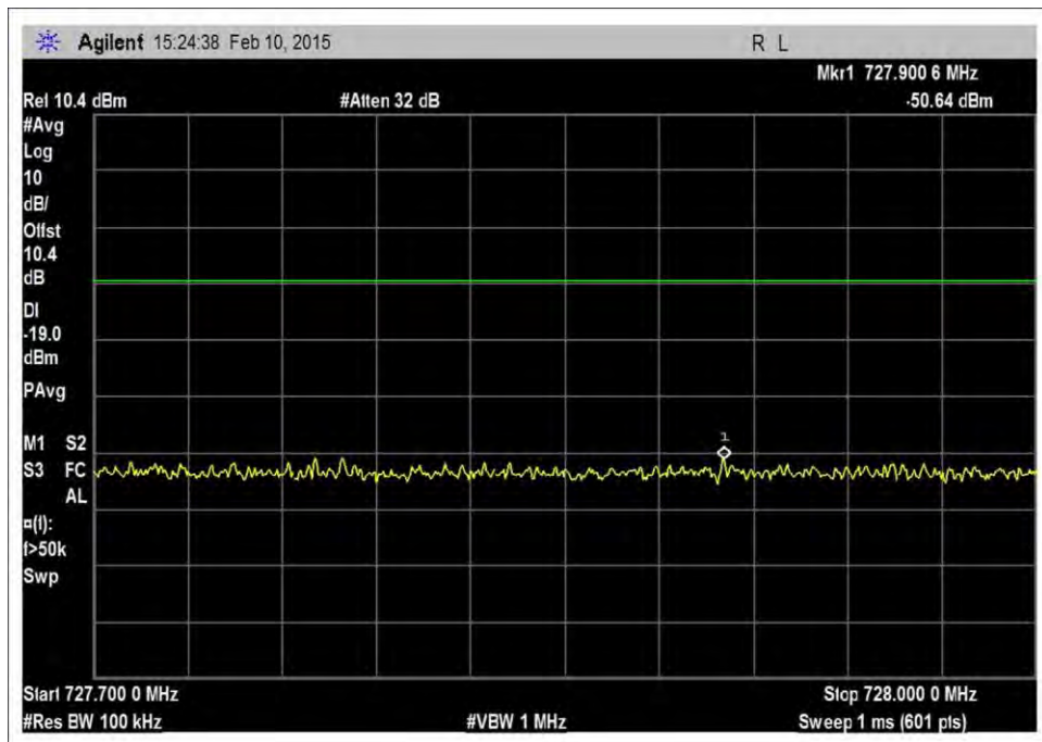
7.5_OBE_DL_728-746MHz_CDMA_L_-56dBm
