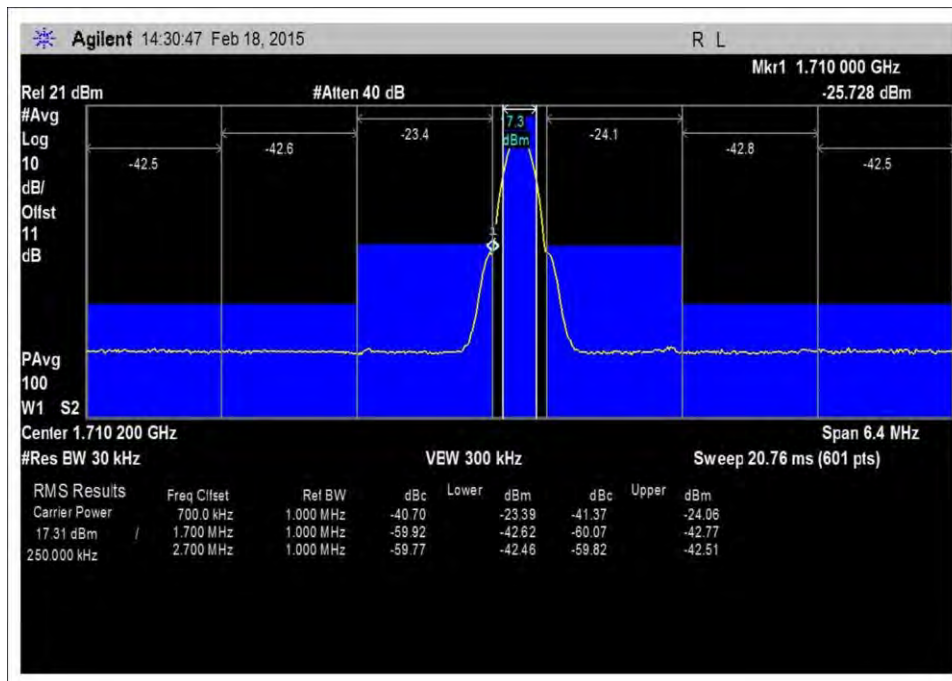
7.5_OBE_UL_1710-1755MHz_GSM_L_-18dBm
