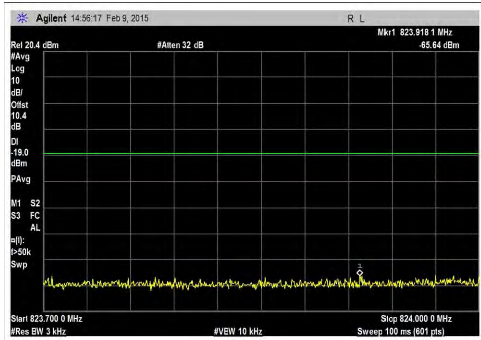
7.5_OBE_UL_824-849MHz_GSM_L_+10dBm
