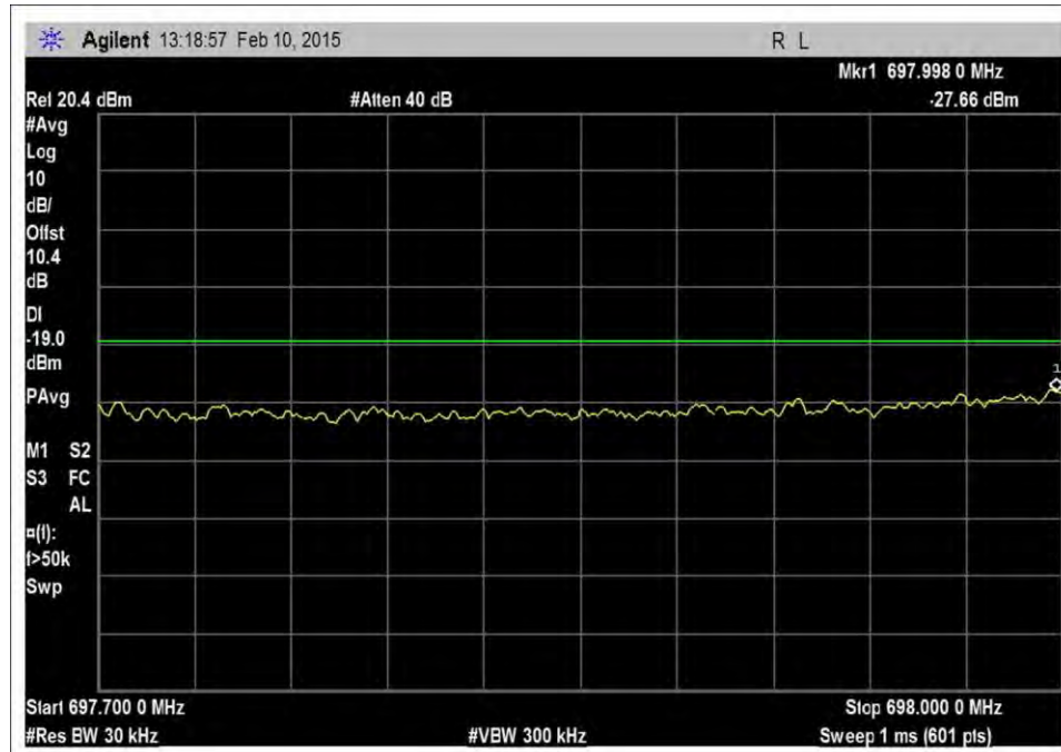
7.5_OBE_UL_698-716MHz_LTE_L_-27dBm
