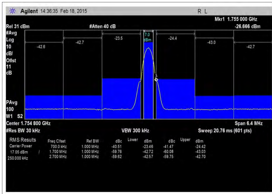
7.5_OBE_UL_1710-1755MHz_GSM_H_-26dBm
