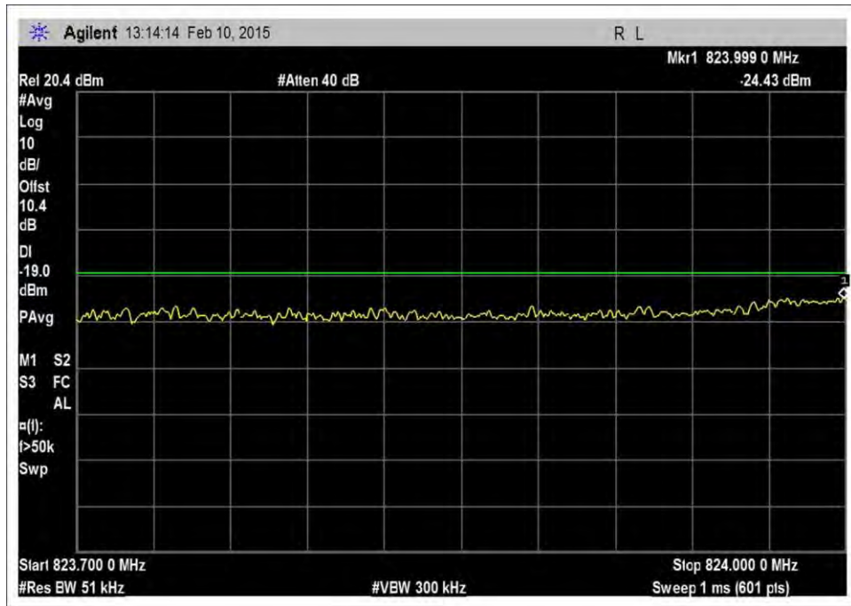
7.5_OBE_UL_824-849MHz_LTE_L_-22dBm
