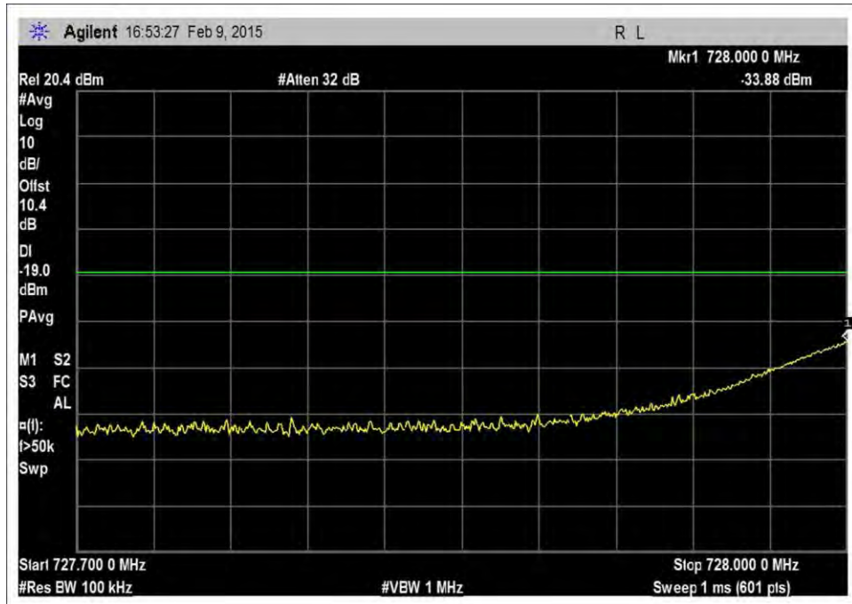
7.5_OBE_DL_728-746MHz_GSM_L_-51dBm
