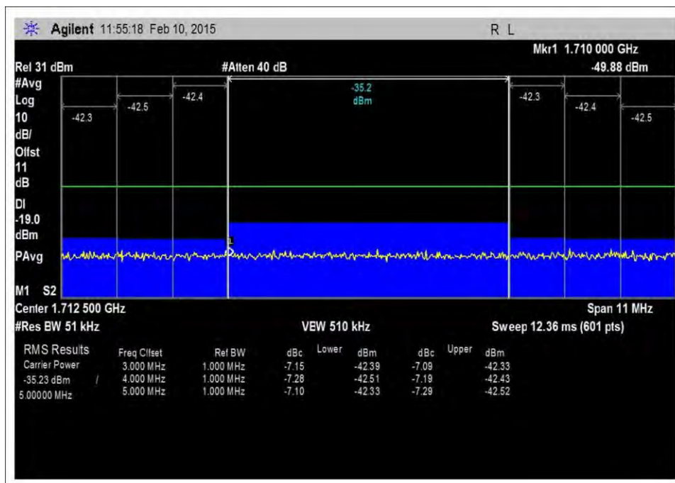
7.5_OBE_UL_1710-1755MHz_LTE_L_+10dBm
