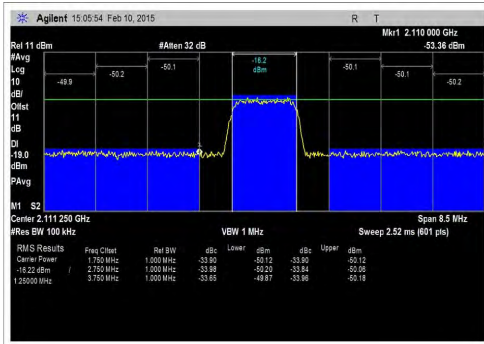
7.5_OBE_DL_2110-2155MHz_CDMA_L_-54dBm
