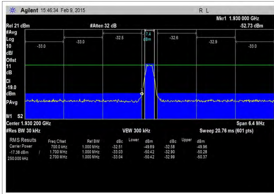
7.5_OBE_DL_1930-1995MHz_GSM_L_-54dBm
