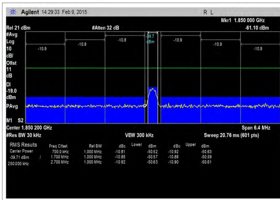
7.5_OBE_UL_1850-1915MHz_GSM_L_+10dBm
