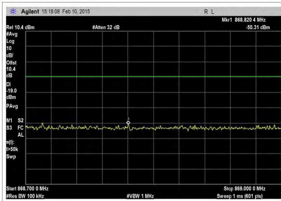
7.5_OBE_DL_869-880MHz_CDMA_L_-46dBm
