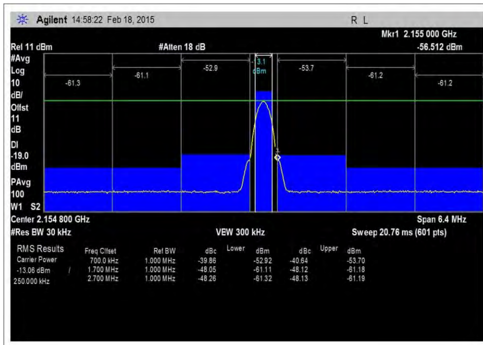
7.5_OBE_DL_2110-2155MHz_GSM_H_-53dBm
