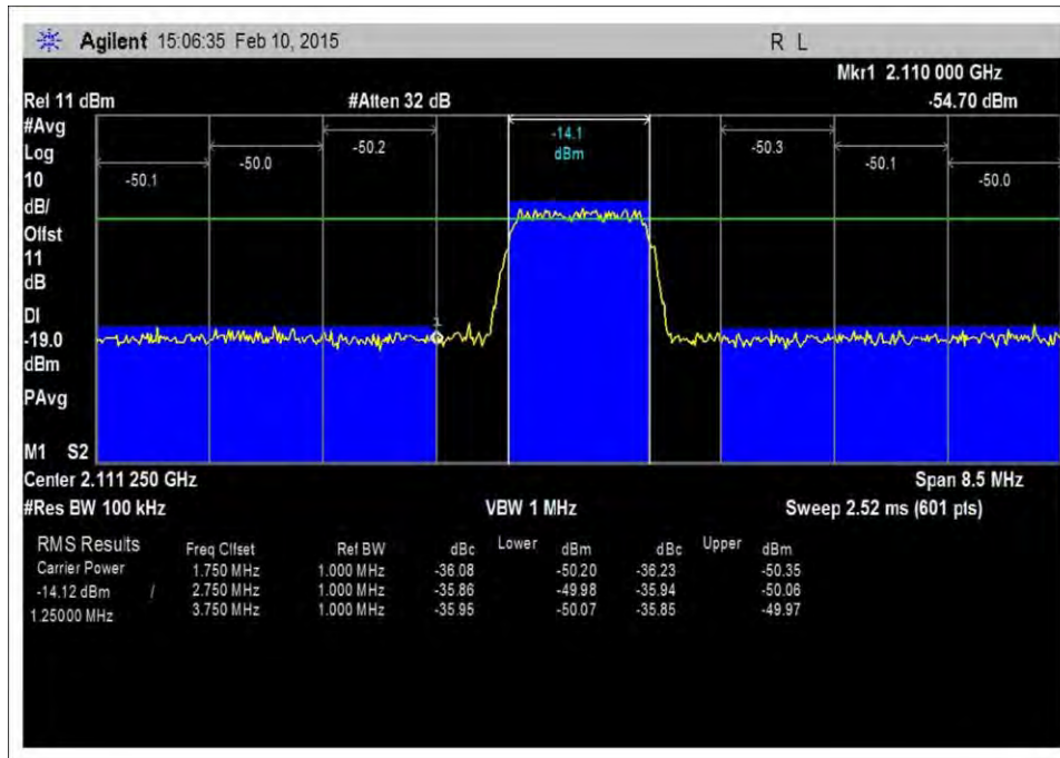
7.5_OBE_DL_2110-2155MHz_CDMA_L_-47dBm
