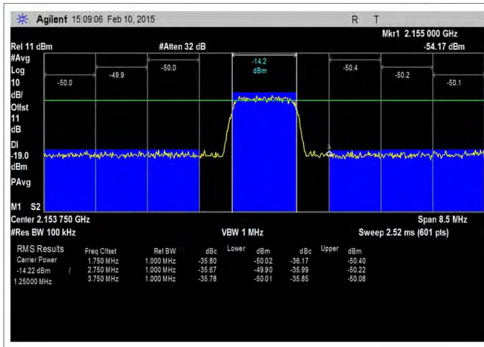
7.5_OBE_DL_2110-2155MHz_CDMA_H_-54dBm
