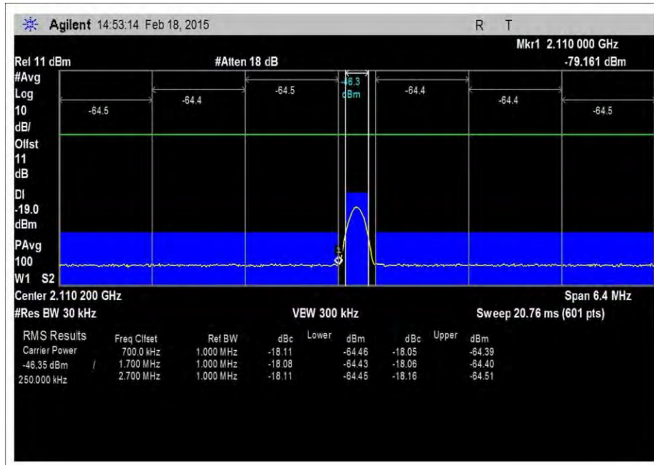
7.5_OBE_DL_2110-2155MHz_GSM_L_-20dBm
