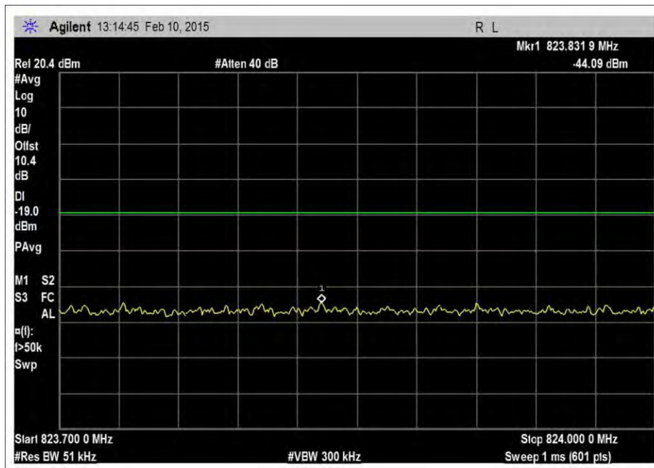
7.5_OBE_UL_824-849MHz_LTE_L_+10dBm
