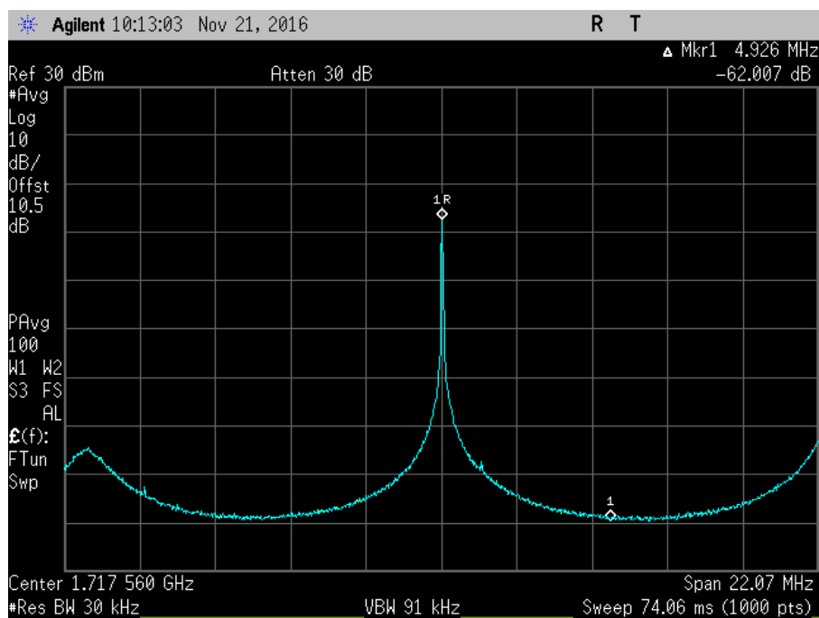
7.11.3_Osc_UL_1710-1755MHz-2_AWGNR
