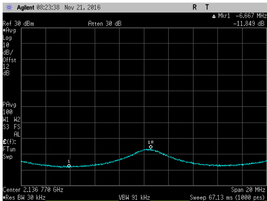
7.11.3_Osc_DL_2110-2155MHz+3_AWGNL
