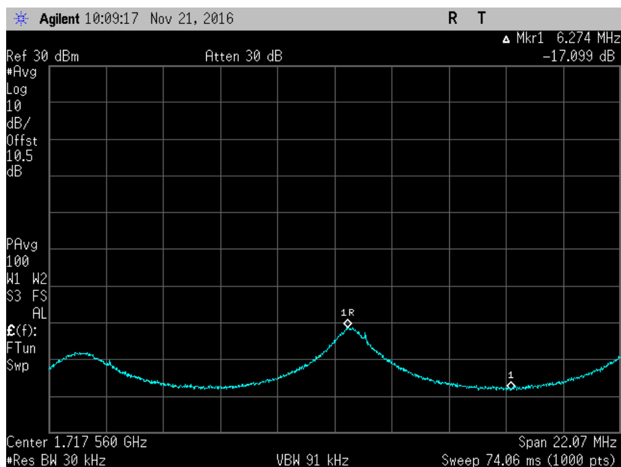
7.11.3_Osc_UL_1710-1755MHz+1_AWGNR
