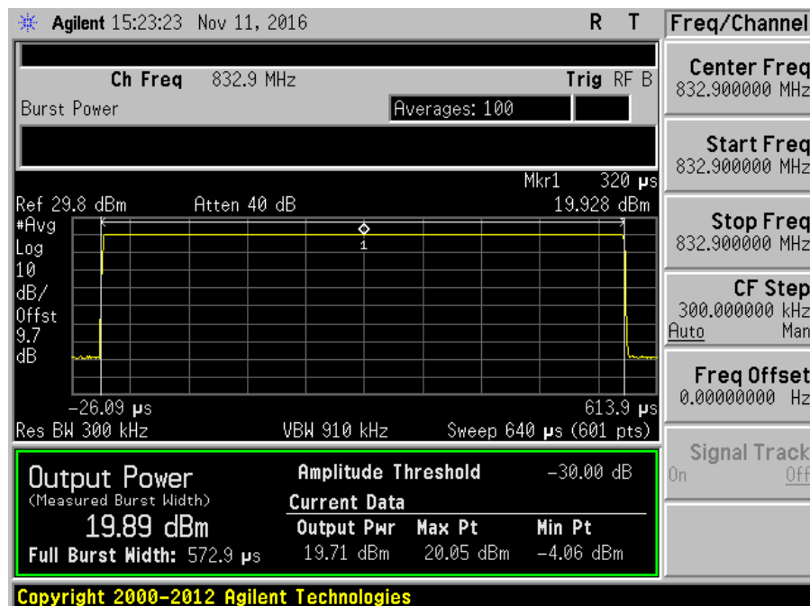
7.2_Power_UL_824-849MHz_GSM_Max
