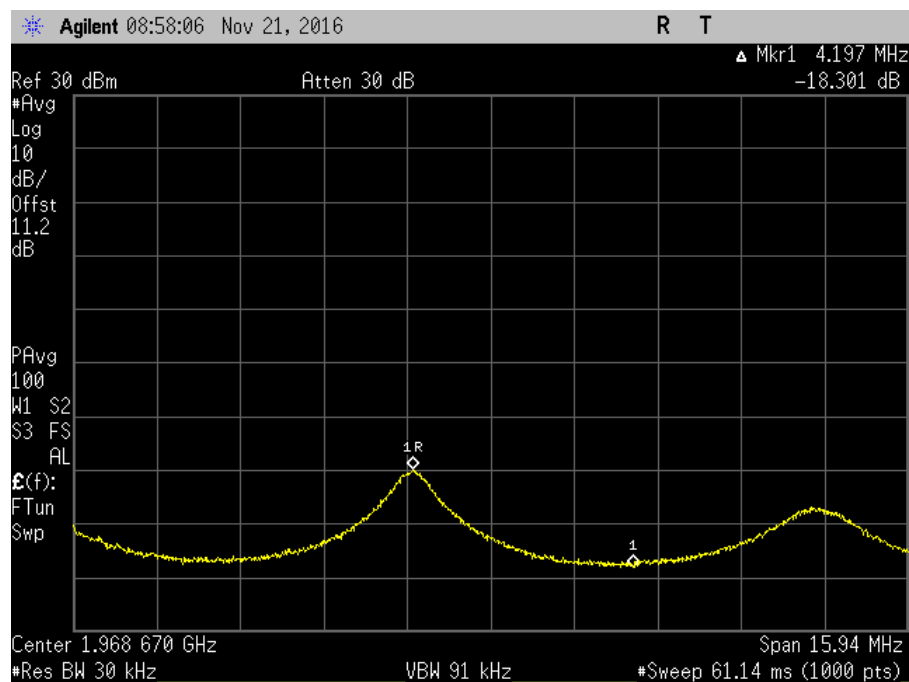
7.11.3_Osc_DL_1930-1995MHz+0_AWGNL
