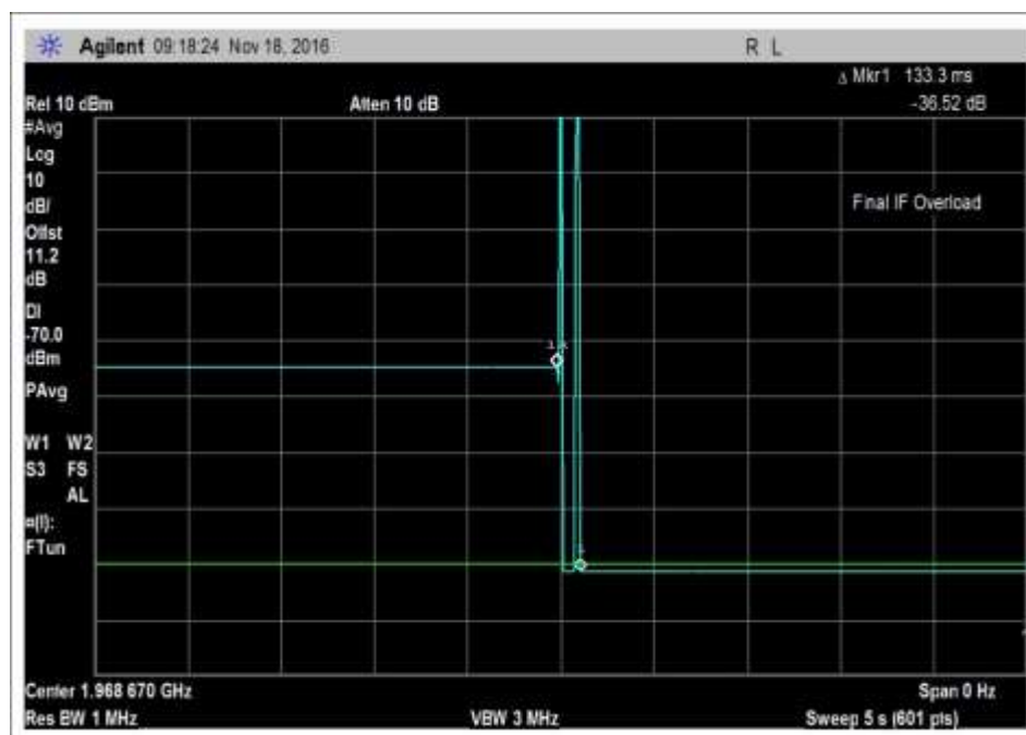
7.11_osc_DL-1930-1995MHz
