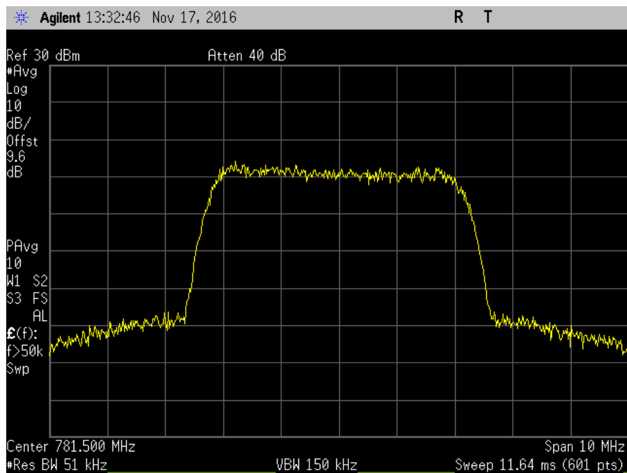
7.10_OBW_UL_776-787MHz_WCDMA_Out
