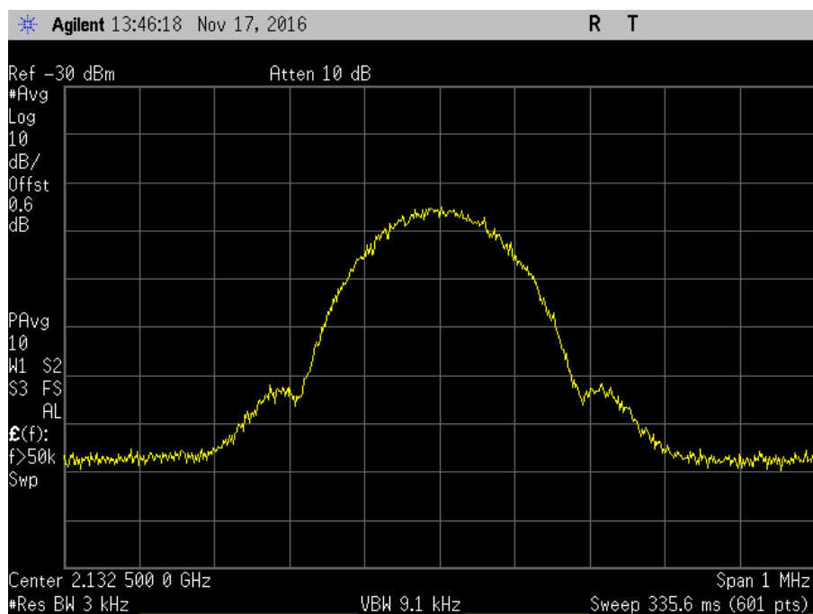
7.10_OBW_DL_2110-2155MHz_GSM_In
