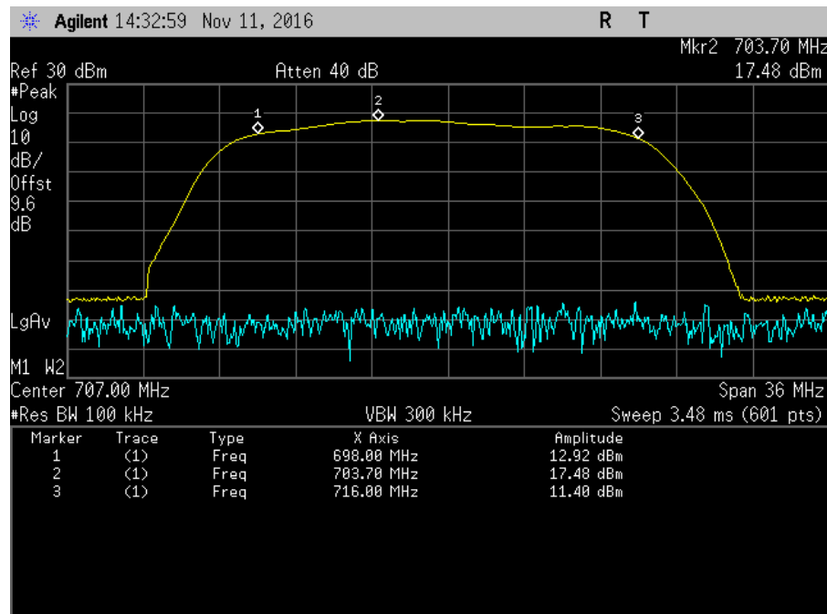
7.1_Band Verify_UL_698-716MHz
