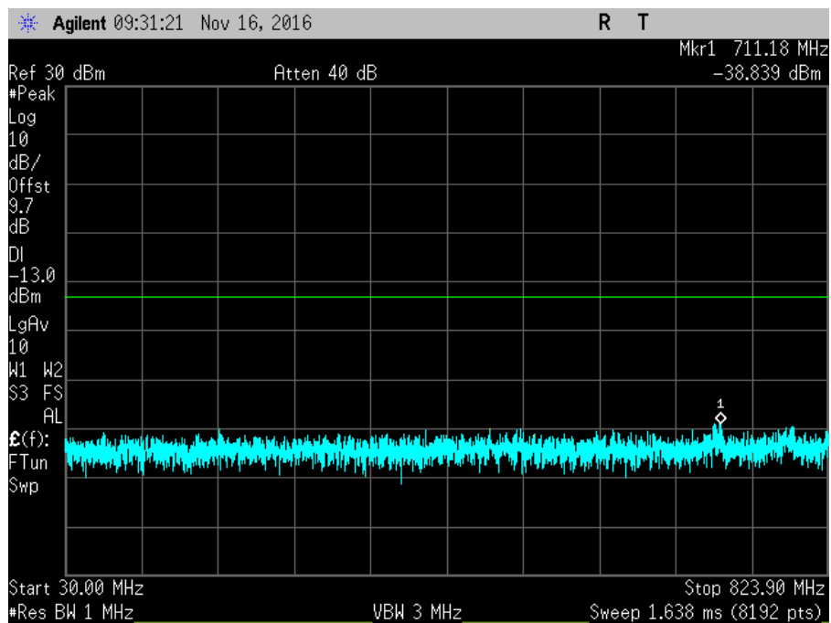
7.6_CSE_UL_824-849MHz_L
