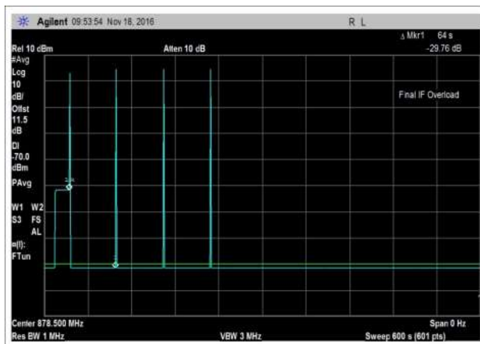
7.11_osc_DL-869-894MHz-600
