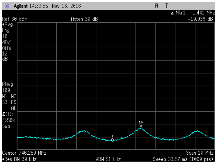
7.11.3_Osc_DL_746-757MHz+3_AWGNR
