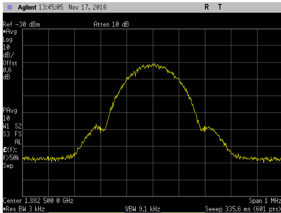
7.10_OBW_UL_1850-1915MHz_GSM_In
