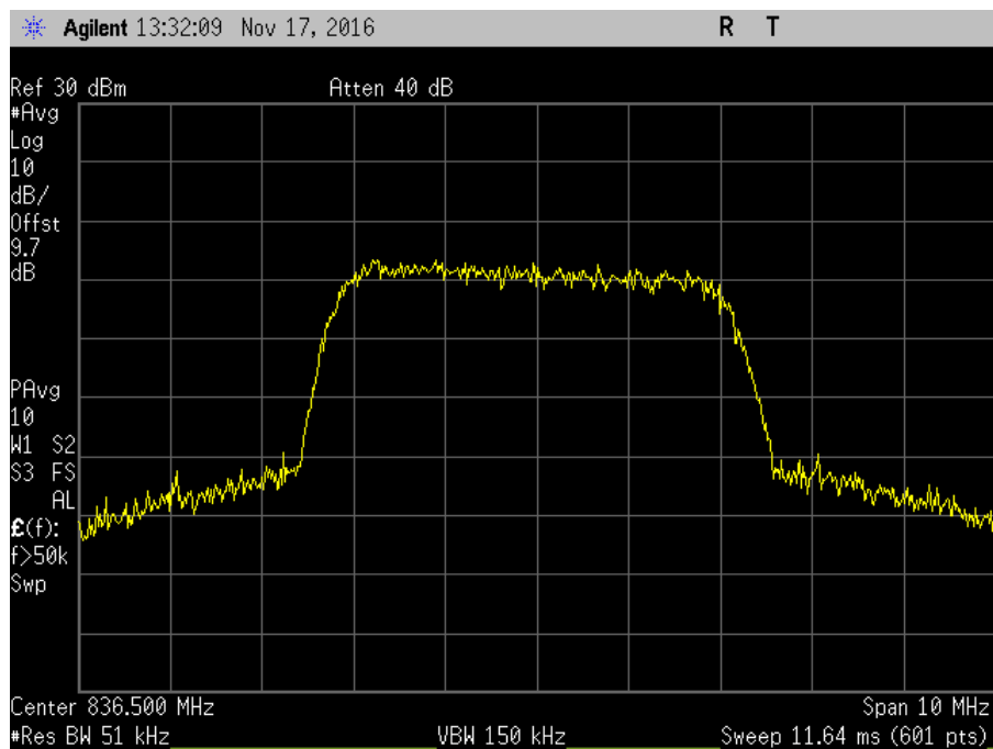
7.10_OBW_UL_824-849MHz_WCDMA_Out
