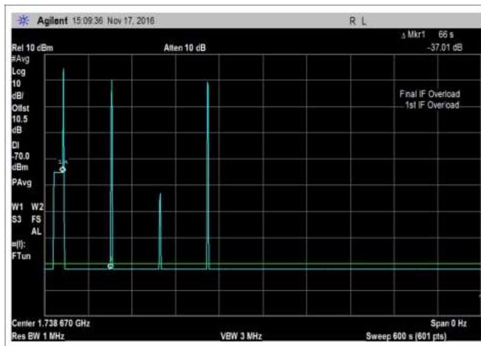
7.11_osc_UL-1710-1755MHz-600sec
