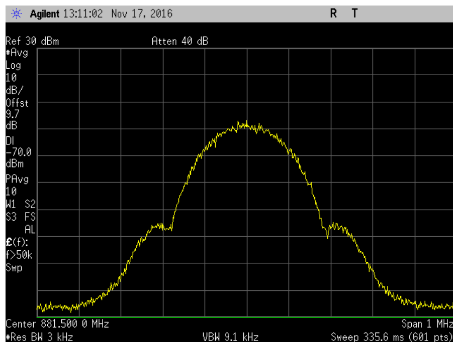
7.10_OBW_DL_869-894MHz_GSM_Out
