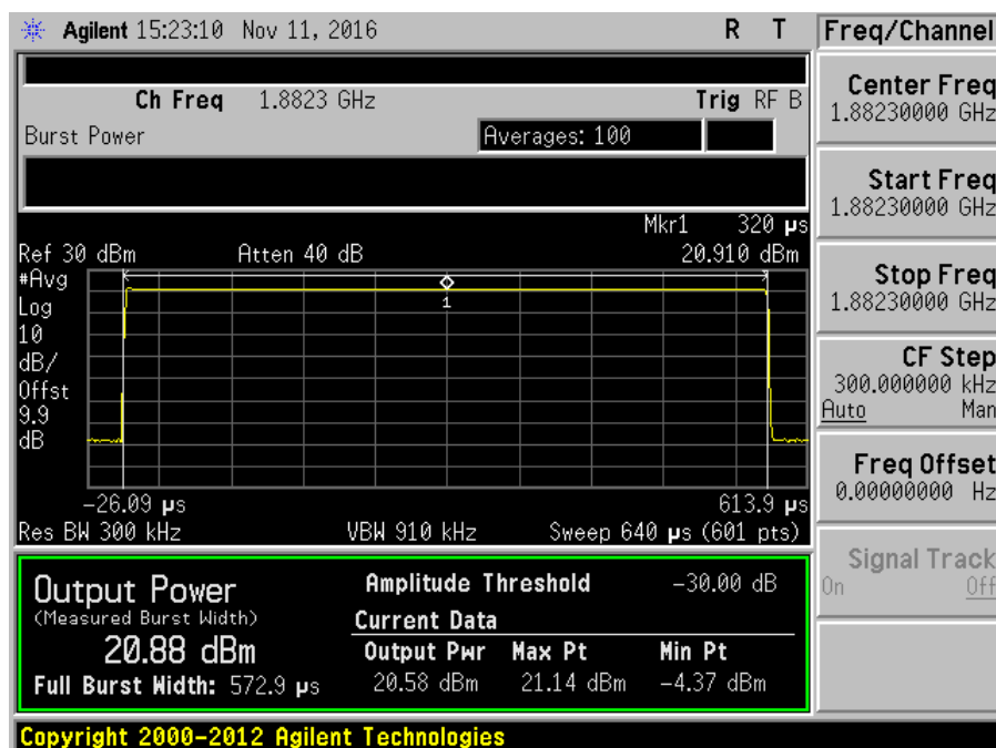
7.2_Power_UL_1850-1915MHz_GSM_Max
