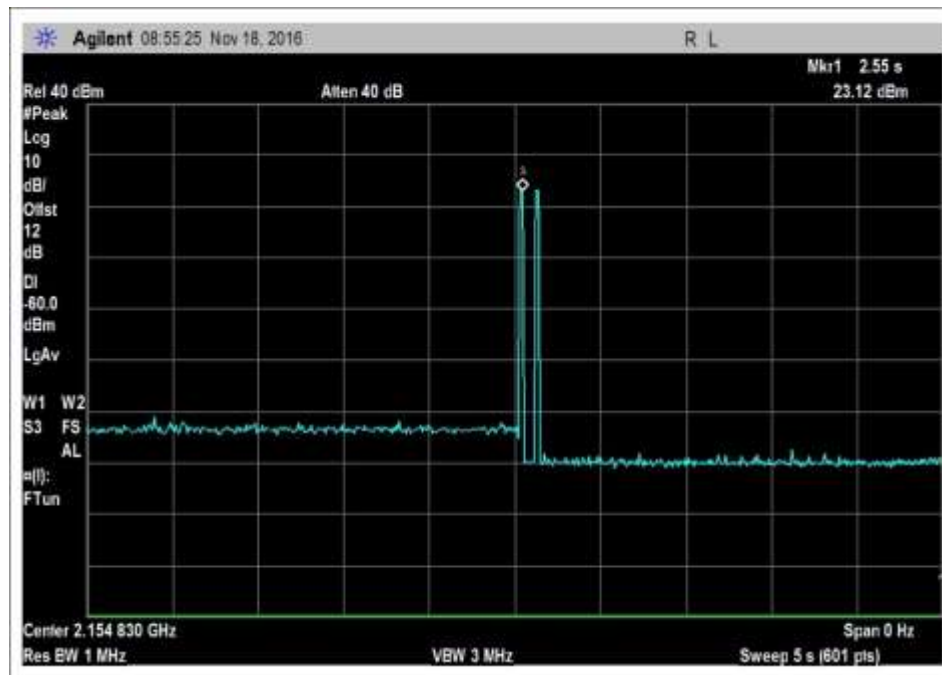
7.11_osc_DL-2110-2155MHz-Pk
