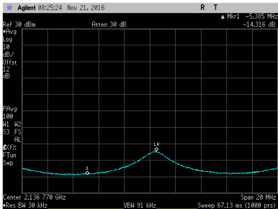
7.11.3_Osc_DL_2110-2155MHz+1_AWGNL
