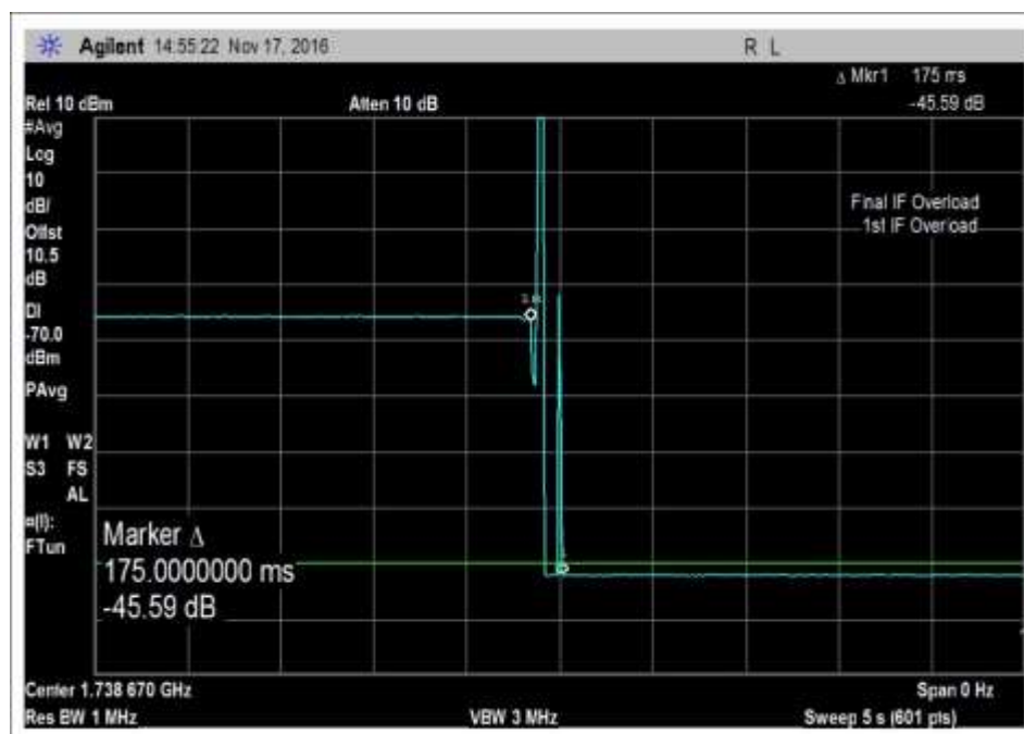
7.11_osc_UL-1710-1755MHz
