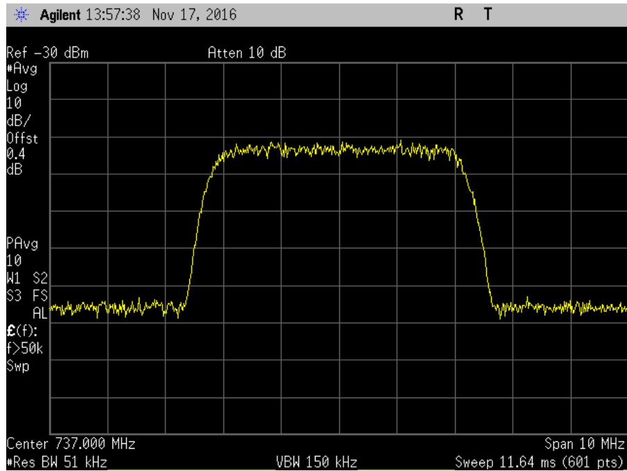
7.10_OBW_DL_728-746MHz_WCDMA_In
