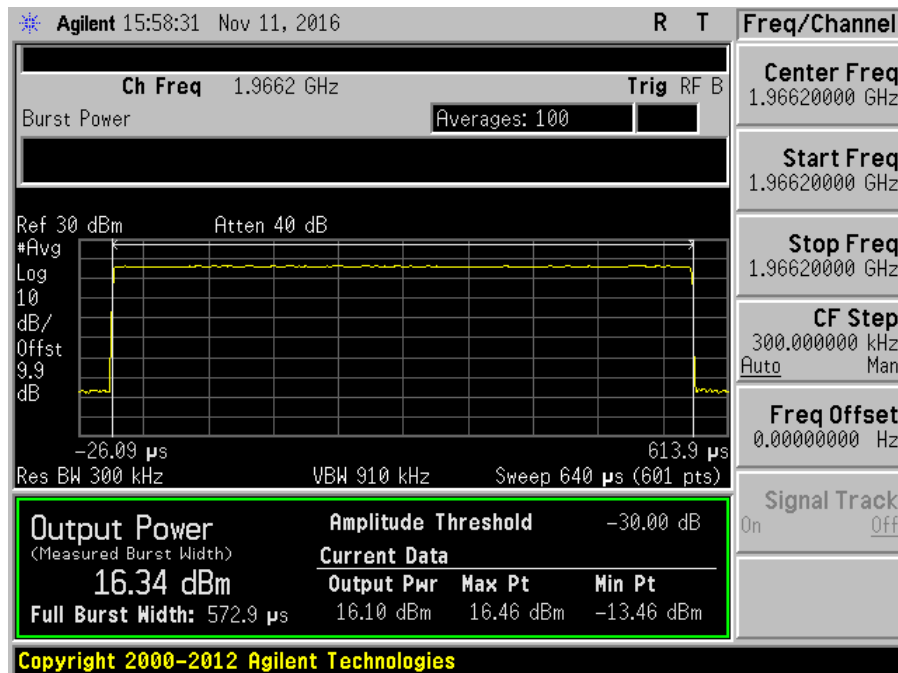
7.2_Power_DL_1930-1995MHz_GSM_Max
