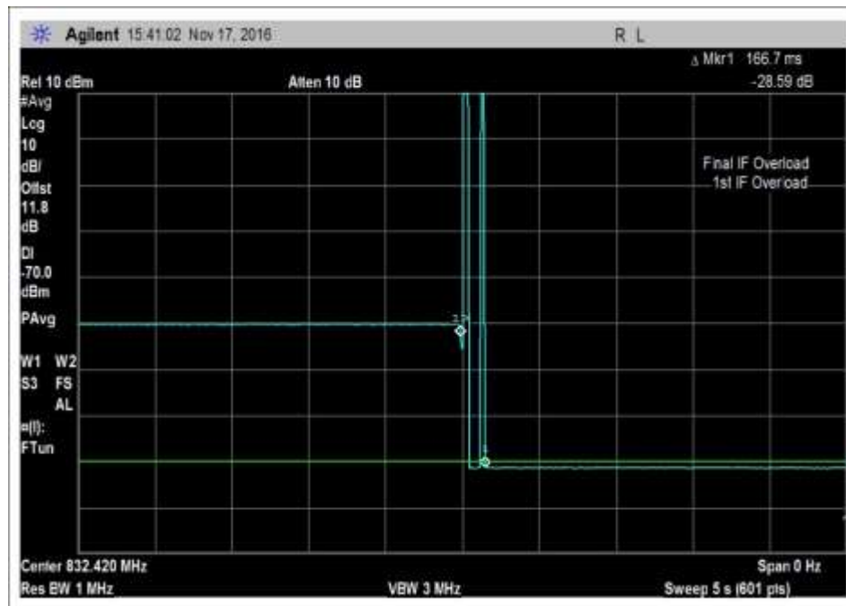
7.11_osc_UL-824-849MHz
