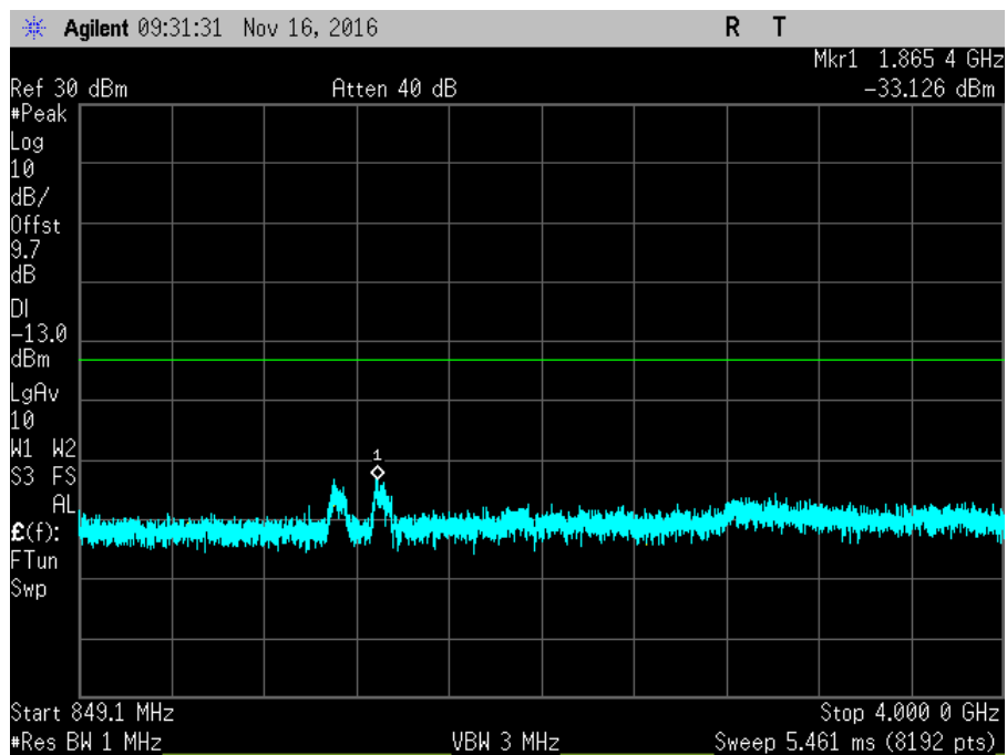
7.6_CSE_UL_824-849MHz_R1
