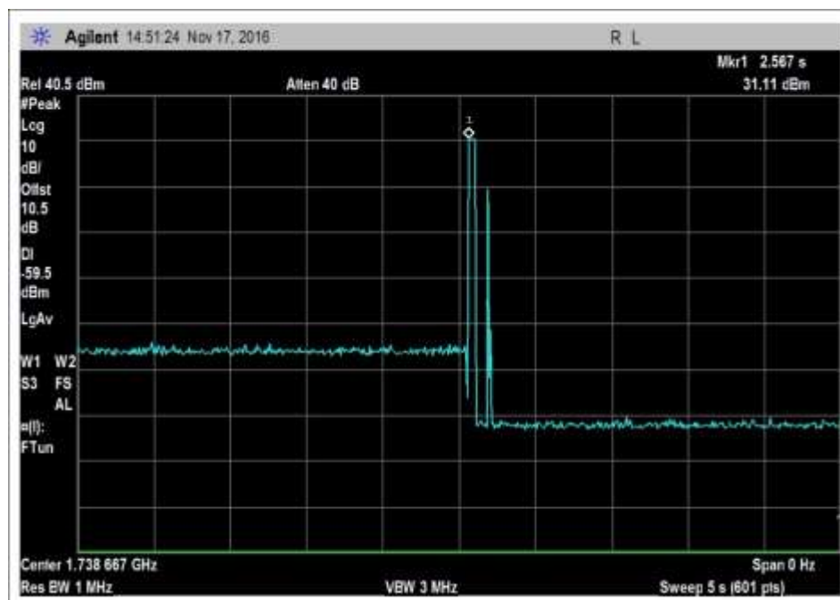
7.11_osc_UL-1710-1755MHz-Pk
