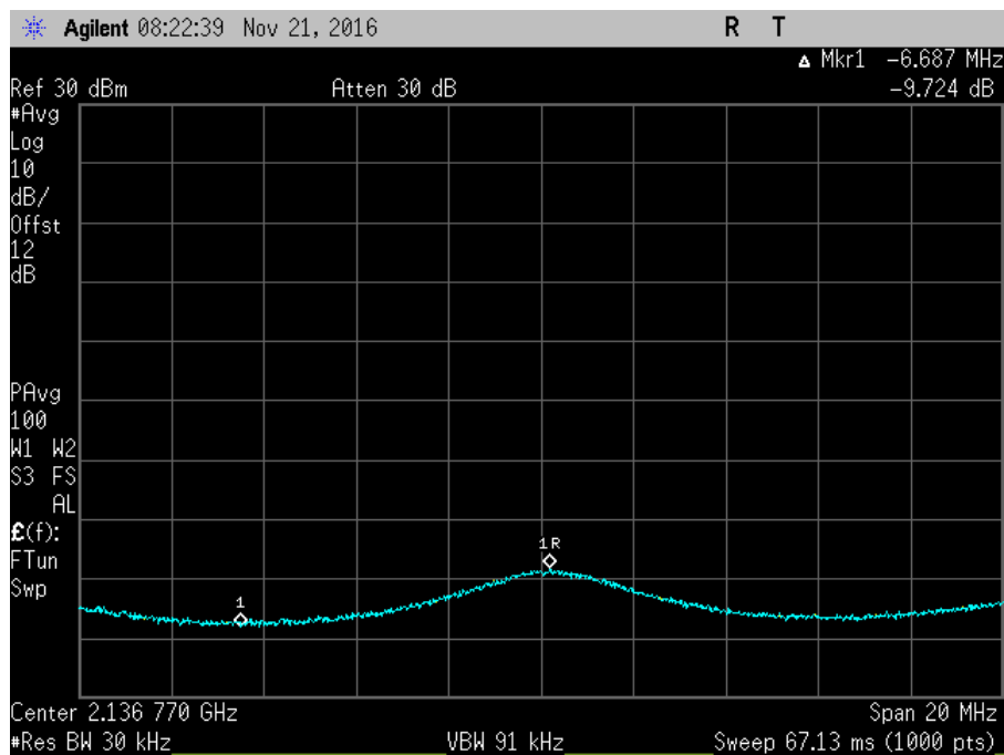
7.11.3_Osc_DL_2110-2155MHz+5_AWGNL
