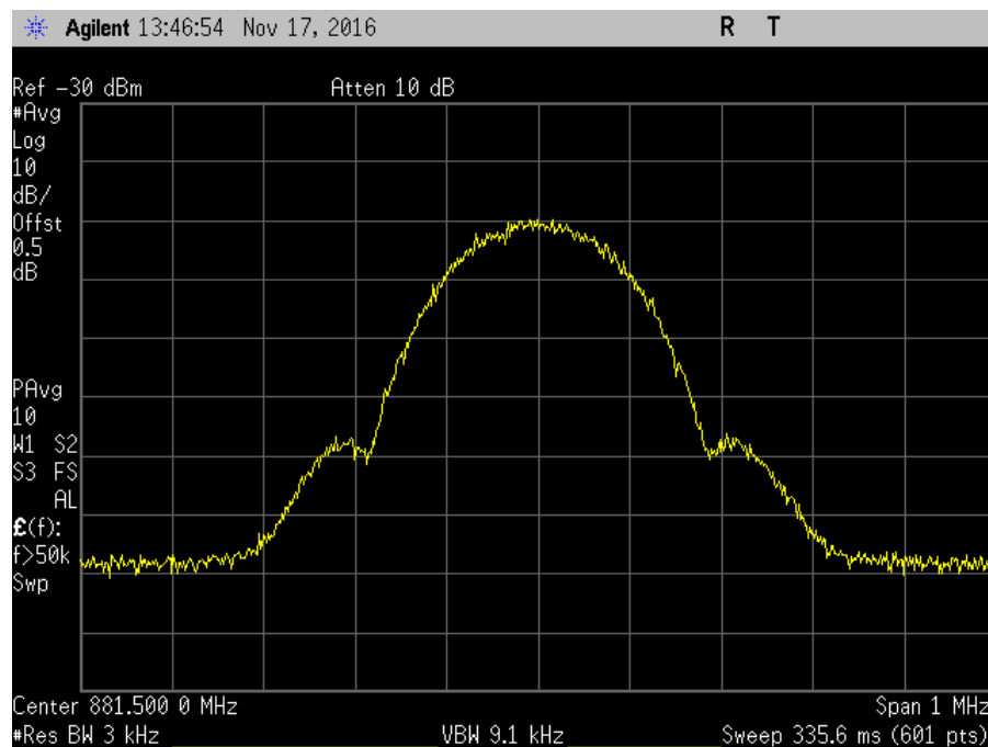
7.10_OBW_DL_869-894MHz_GSM_In
