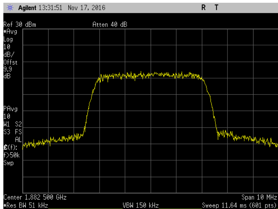
7.10_OBW_UL_1850-1915MHz_WCDMA_Out
