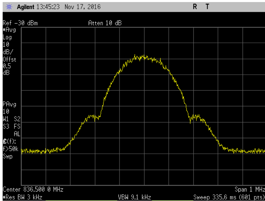
7.10_OBW_UL_824-849MHz_GSM_In
