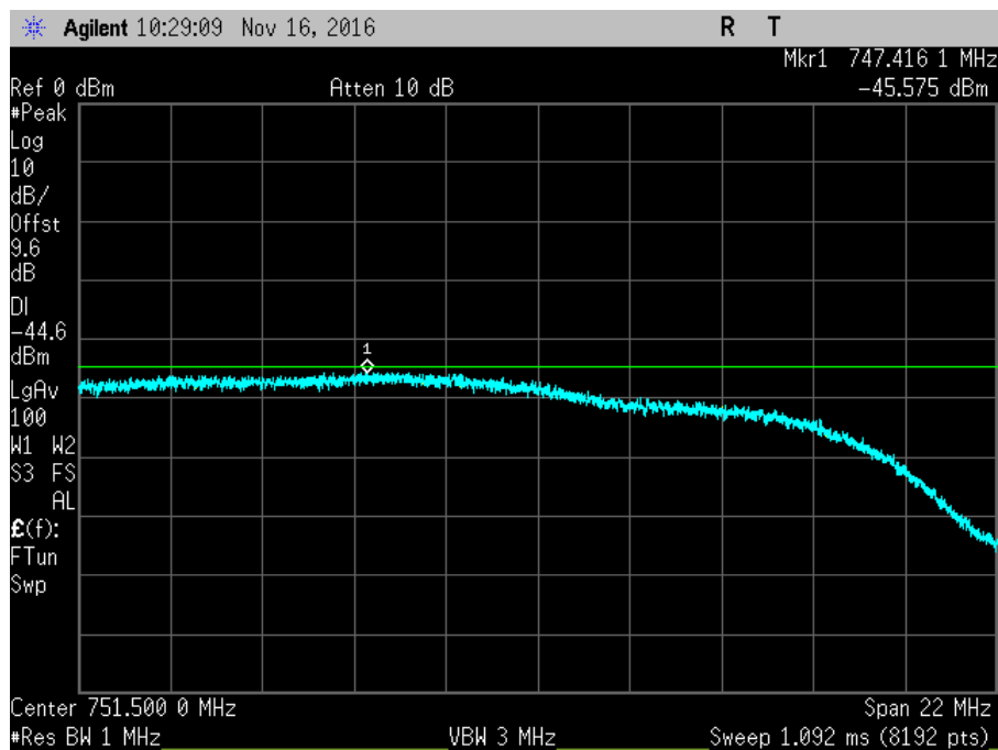
7.7.1_Noise_DL_746-757MHz
