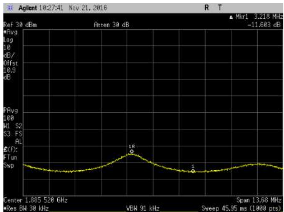
7.11.3_Osc_UL_1850-1915MHz+5_AWGNL
