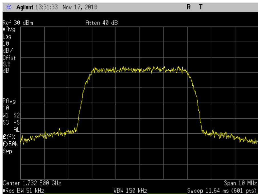
7.10_OBW_UL_1710-1755MHz_WCDMA_Out
