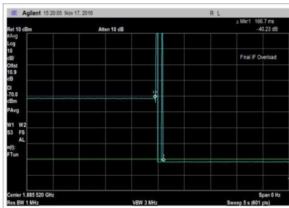
7.11_osc_UL-1850-1915MHz
