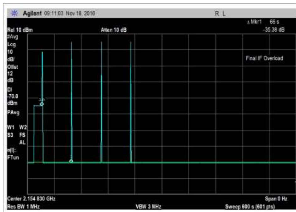
7.11_osc_DL-2110-2155MHz-600sec
