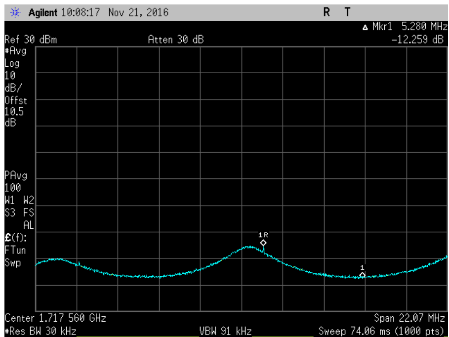
7.11.3_Osc_UL_1710-1755MHz+3_AWGNR
