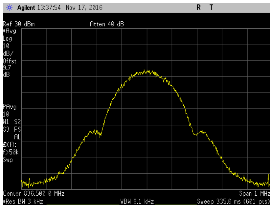
7.10_OBW_UL_824-849MHz_GSM_Out
