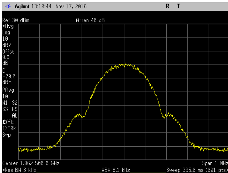
7.10_OBW_DL_1930-1995MHz_GSM_Out
