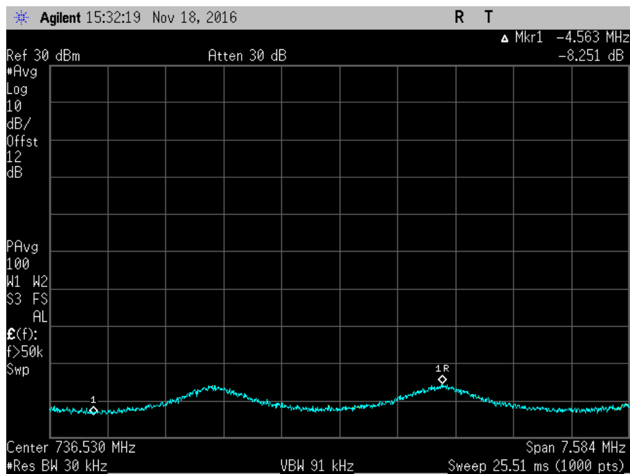
7.11.3_Osc_DL_728-746MHz+5_AWGNR
