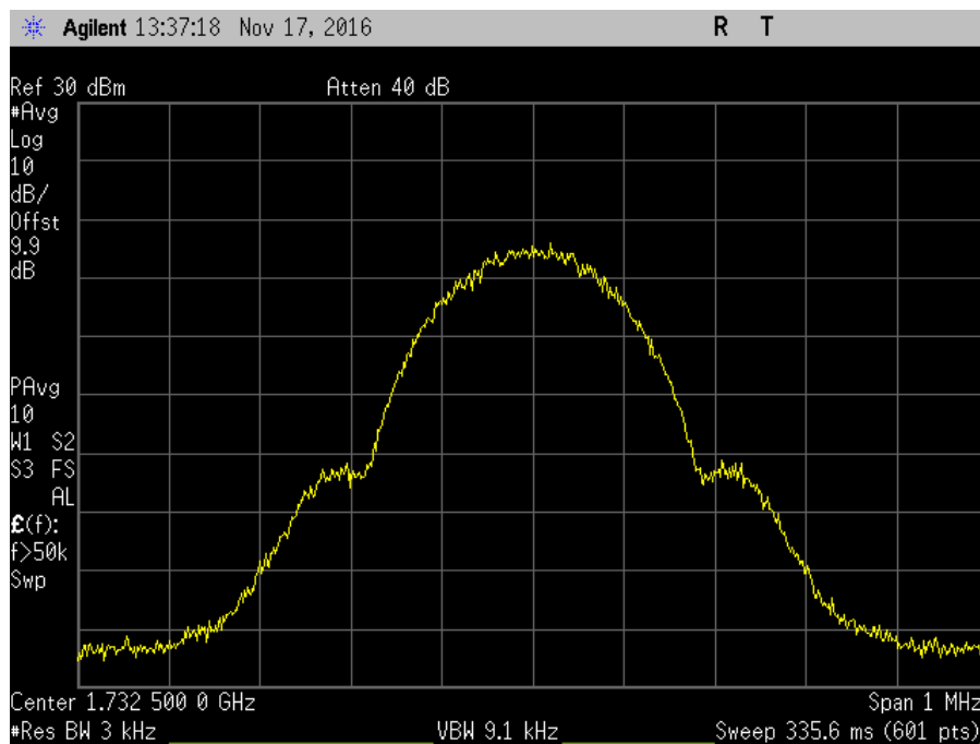
7.10_OBW_UL_1710-1755MHz_GSM_Out
