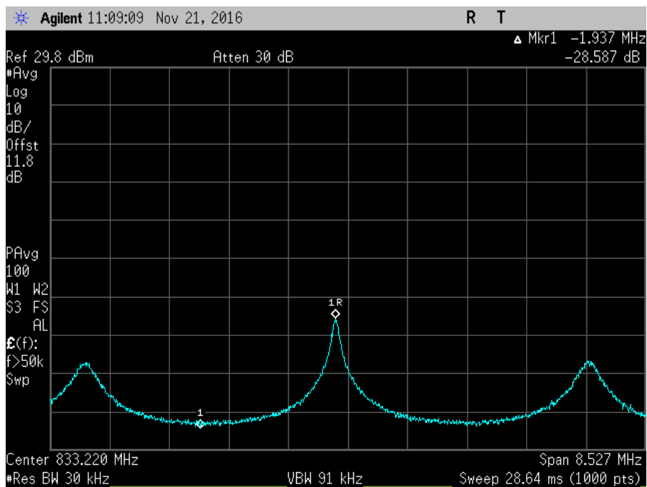
7.11.3_Osc_UL_824-849MHz-2_AWGNR
