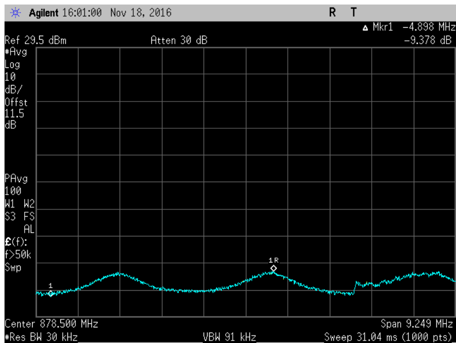
7.11.3_Osc_DL_869-894MHz+5_AWGNR
