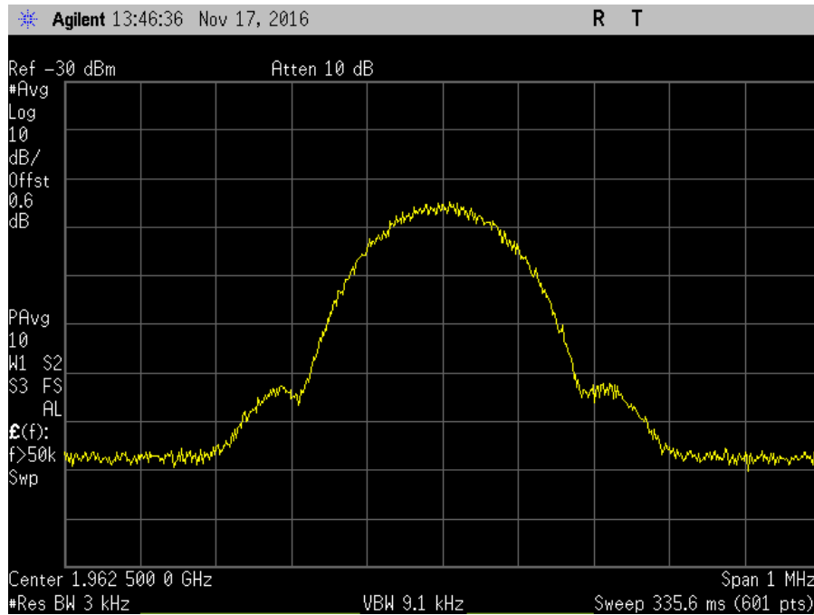
7.10_OBW_DL_1930-1995MHz_GSM_In
