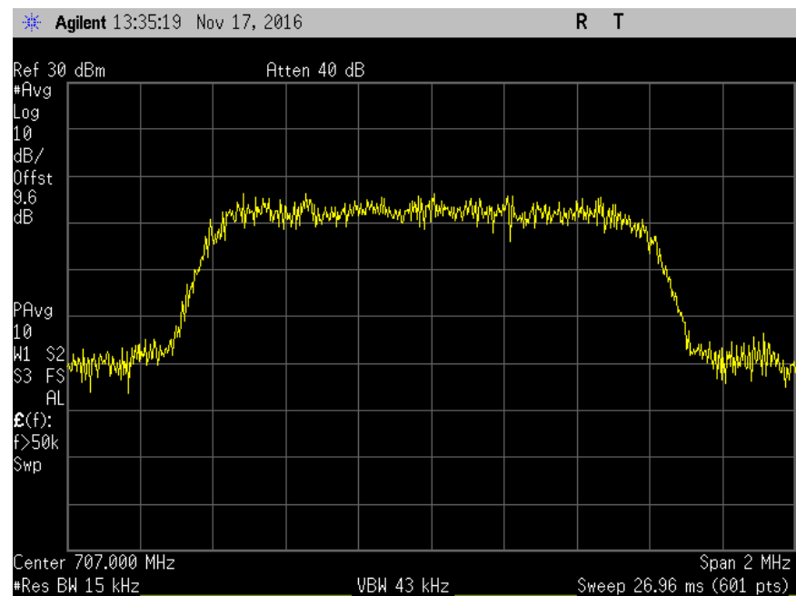
7.10_OBW_UL_698-716MHz_CDMA_Out
