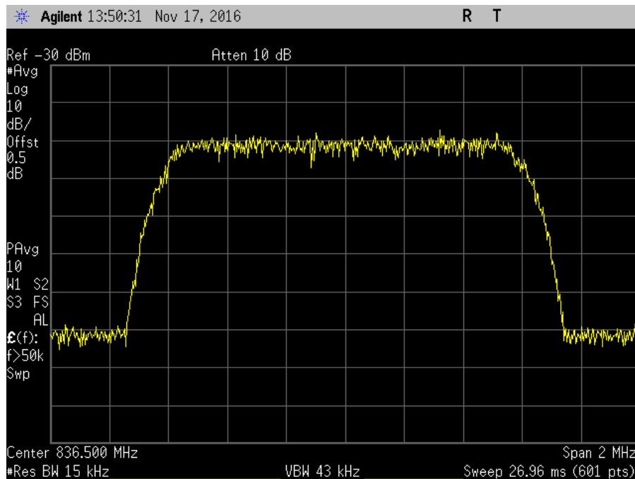
7.10_OBW_UL_824-849MHz_CDMA_In
