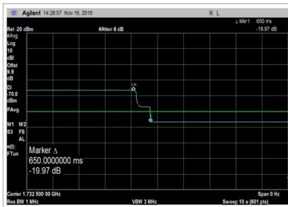
7.7_VarNoise_UL_1710-1755MHz
