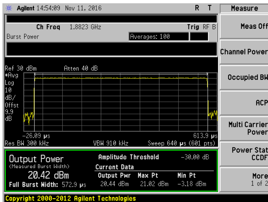
7.2_Power_UL_1850-1915MHz_GSM
