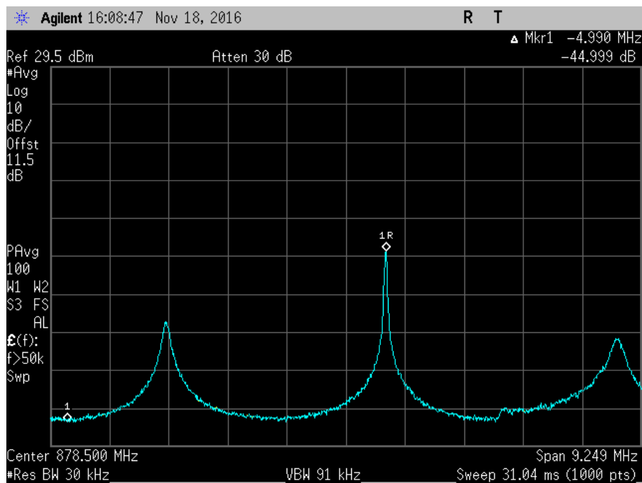
7.11.3_Osc_DL_869-894MHz-2_AWGNR
