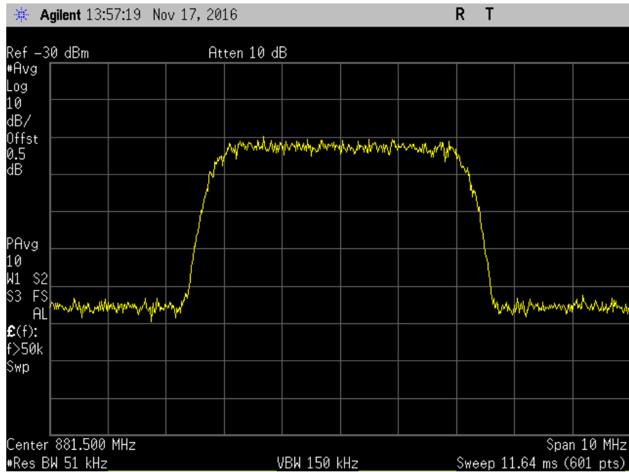
7.10_OBW_DL_869-894MHz_WCDMA_In
