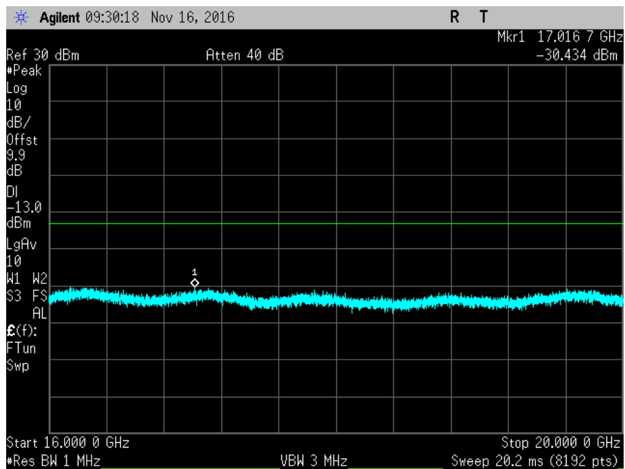
7.6_CSE_UL_1710-1755MHz_R5
