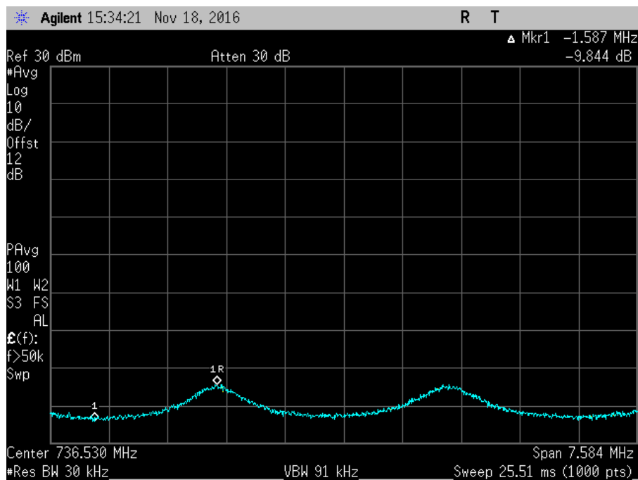
7.11.3_Osc_DL_728-746MHz+3_AWGNR
