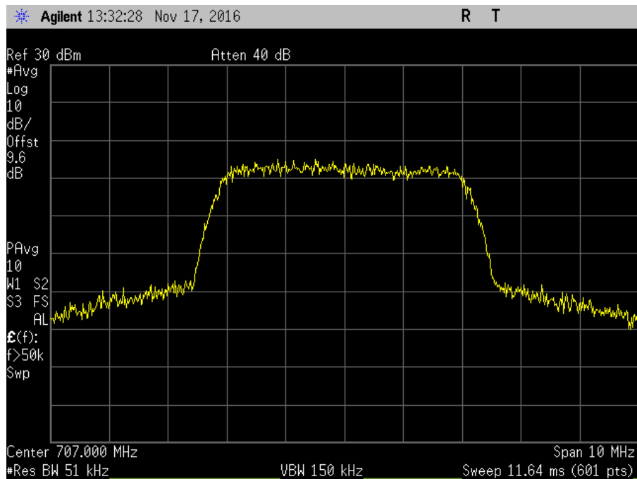
7.10_OBW_UL_698-716MHz_WCDMA_Out
