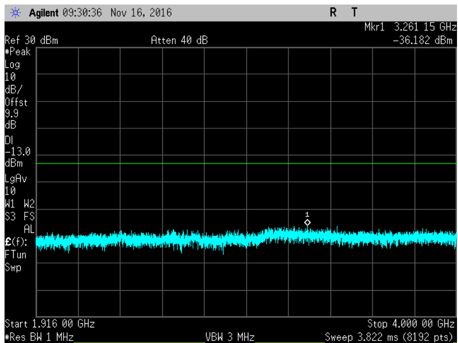
7.6_CSE_UL_1850-1915MHz_R1
