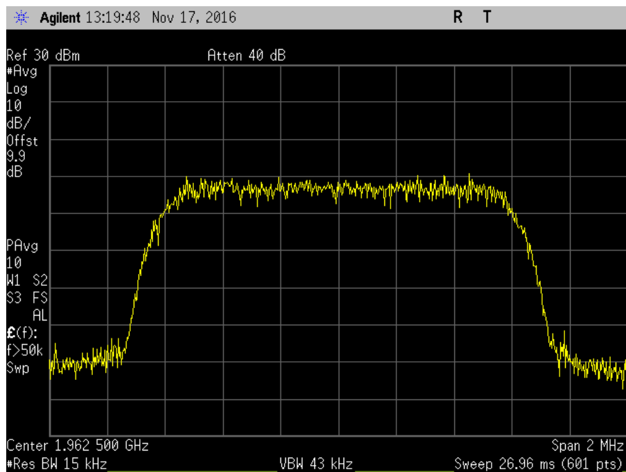
7.10_OBW_DL_1930-1995MHz_CDMA_Out
