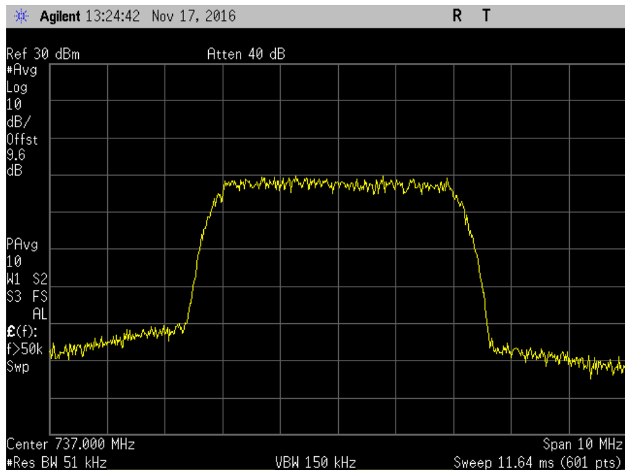
7.10_OBW_DL_728-746MHz_WCDMA_Out
