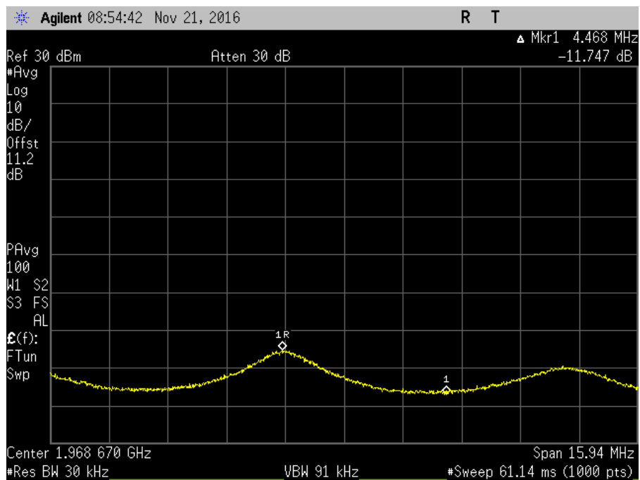
7.11.3_Osc_DL_1930-1995MHz+3_AWGNL
