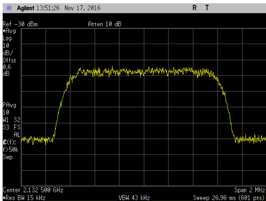
7.10_OBW_DL_2110-2155MHz_CDMA_In
