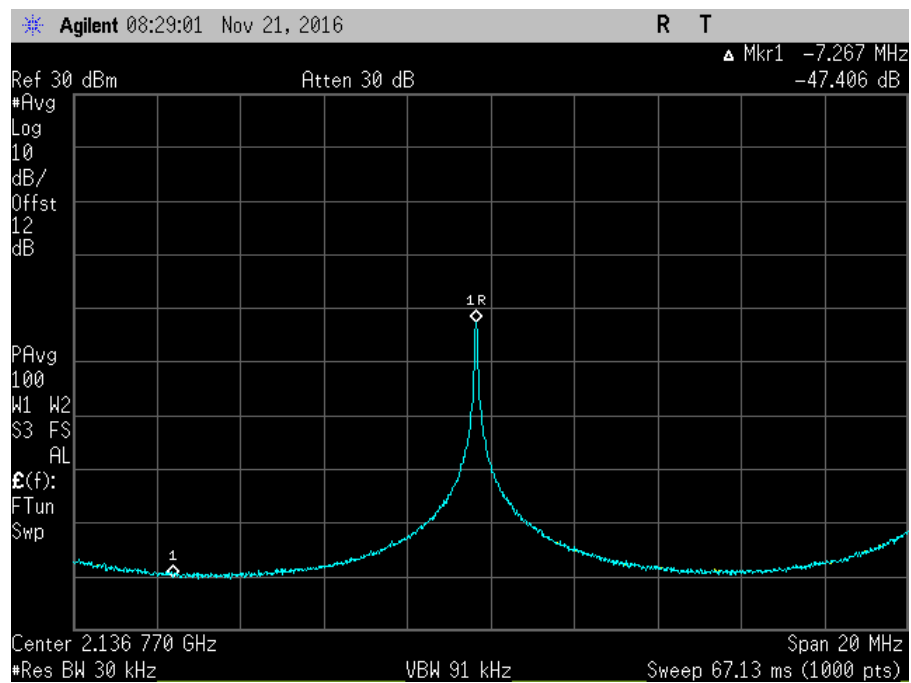
7.11.3_Osc_DL_2110-2155MHz-3_AWGNL
