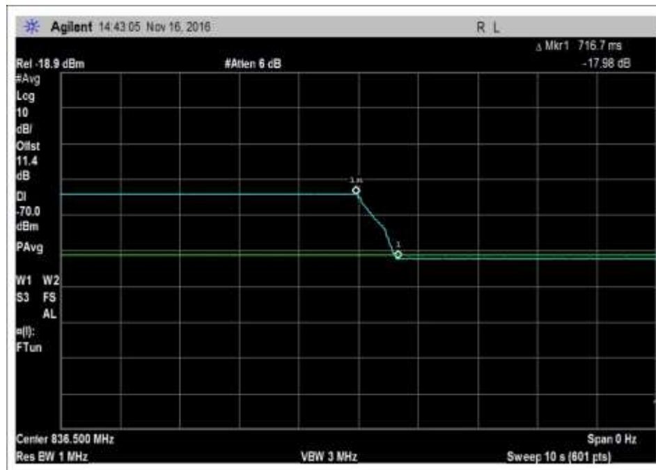
7.7_VarNoise_UL_824-849MHz
