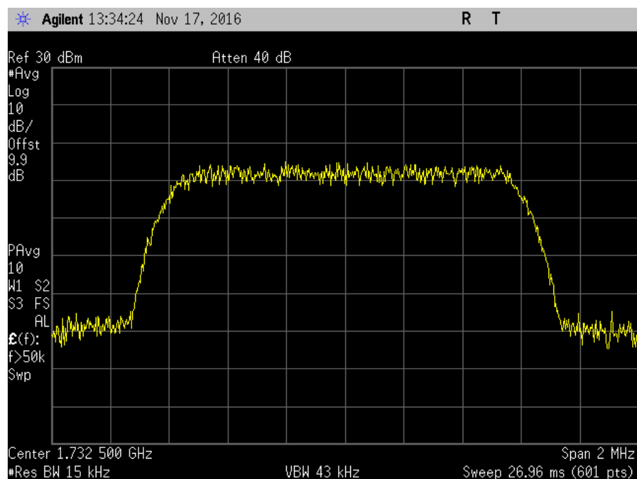
7.10_OBW_UL_1710-1755MHz_CDMA_Out
