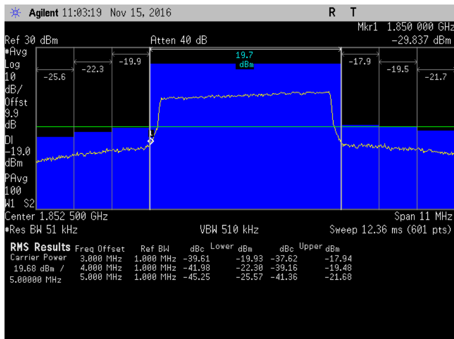
7.5_OBE_UL_1850-1915MHz_L_PreAGC_LTE
