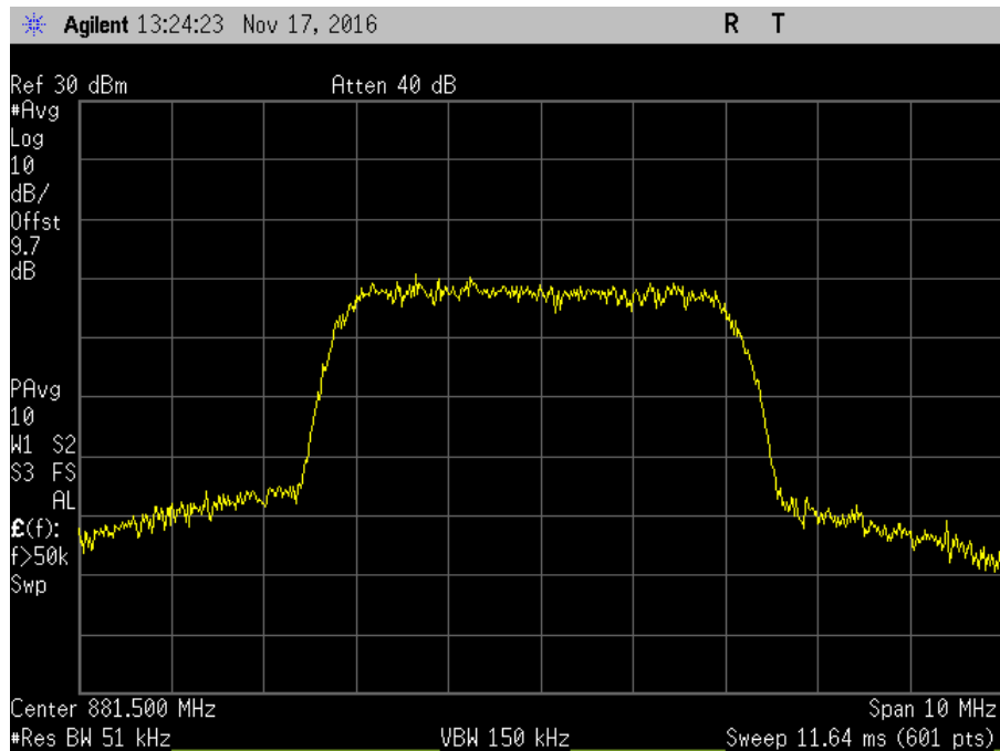
7.10_OBW_DL_869-894MHz_WCDMA_Out
