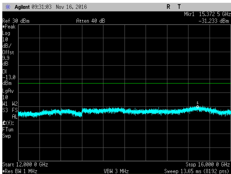
7.6_CSE_UL_1850-1915MHz_R4
