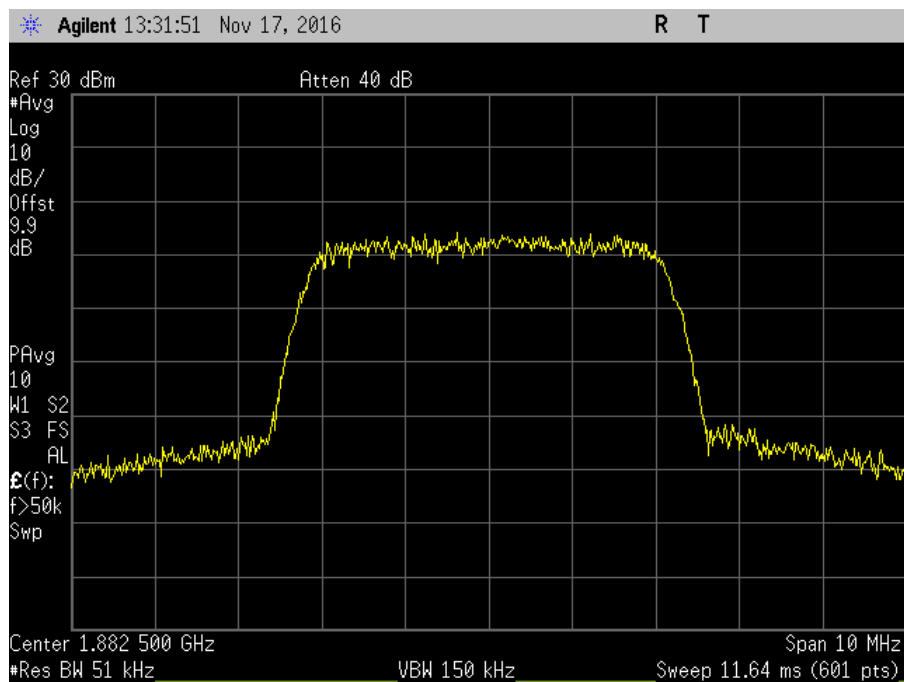
7.10_OBW_UL_1850-1915MHz_WCDMA_Out
