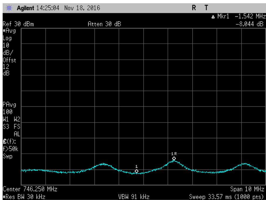
7.11.3_Osc_DL_746-757MHz+4_AWGNR
