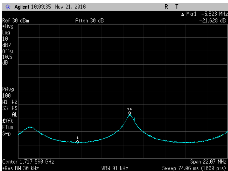
7.11.3_Osc_UL_1710-1755MHz+0_AWG NR
