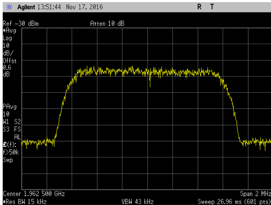
7.10_OBW_DL_1930-1995MHz_CDMA_In
