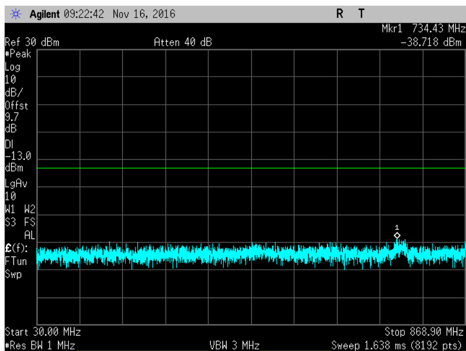
7.6_CSE_DL_869-894MHz_L
