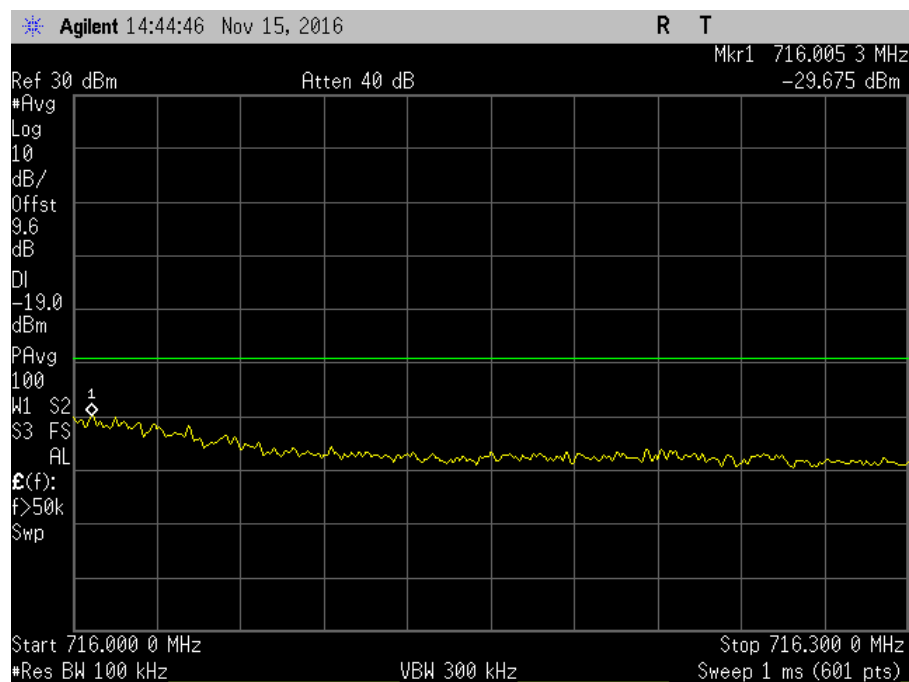
7.5_OBE_UL_698-716MHz_H_PreAGC_LTE
