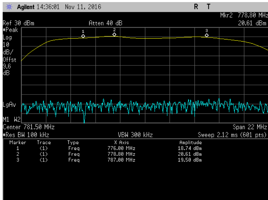
7.1_Band Verify_UL_776-787MHz
