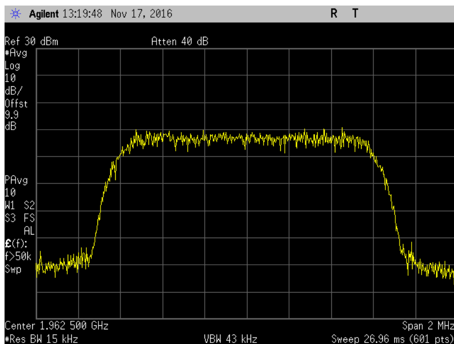
7.10_OBW_DL_1930-1995MHz_CDMA_Out
