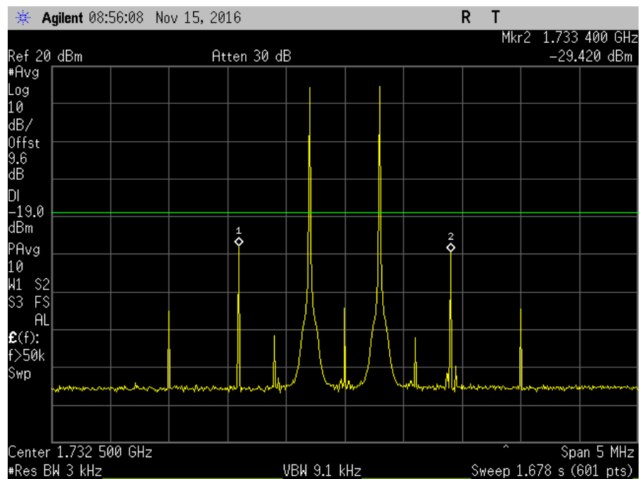
7.4_Intermod_UL_1710-1755MHz
