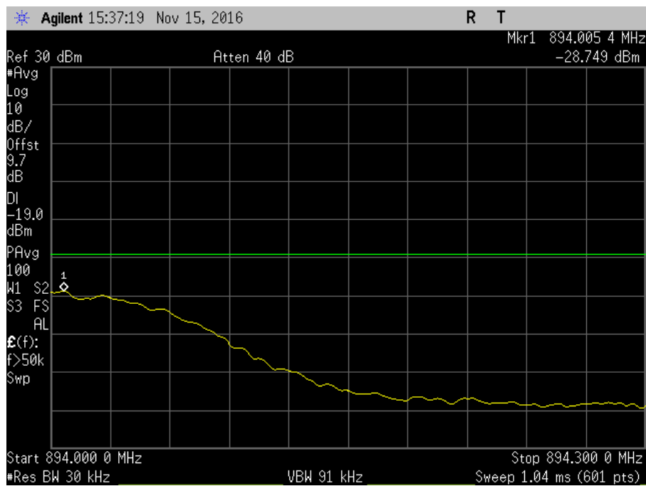
7.5_OBE_DL_869-894MHz_H_PreAGC_GSM
