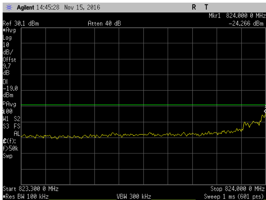
7.5_OBE_UL_824-849MHz_L_PreAGC_LTE
