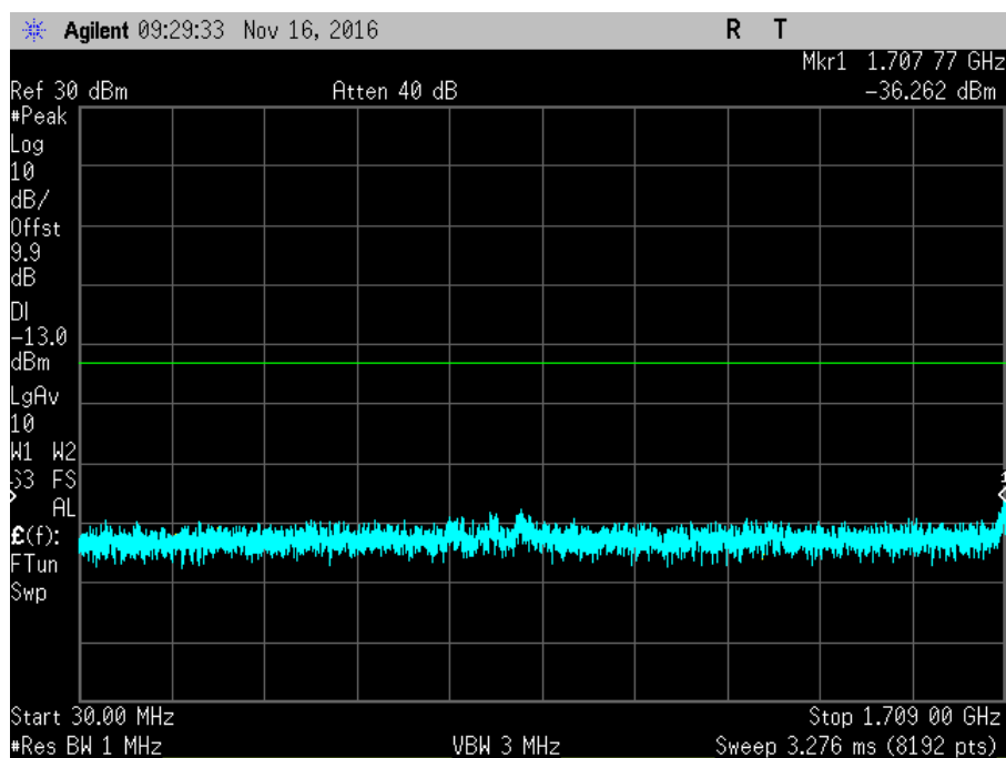
7.6_CSE_UL_1710-1755MHz_L
