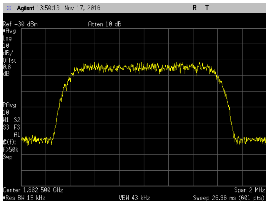
7.10_OBW_UL_1850-1915MHz_CDMA_In
