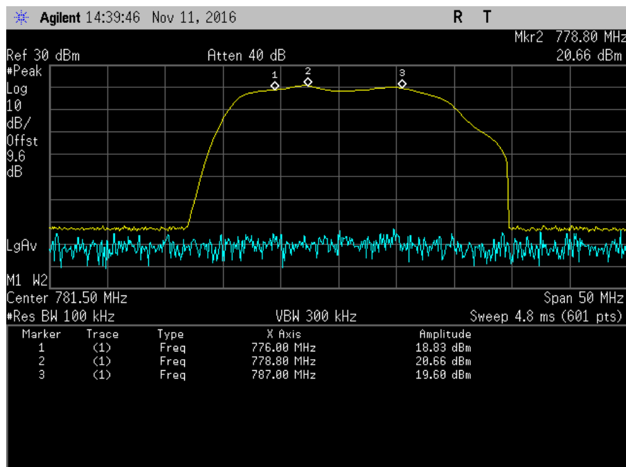
7.1_Band Verify_UL_776-787MHz_Zoom
