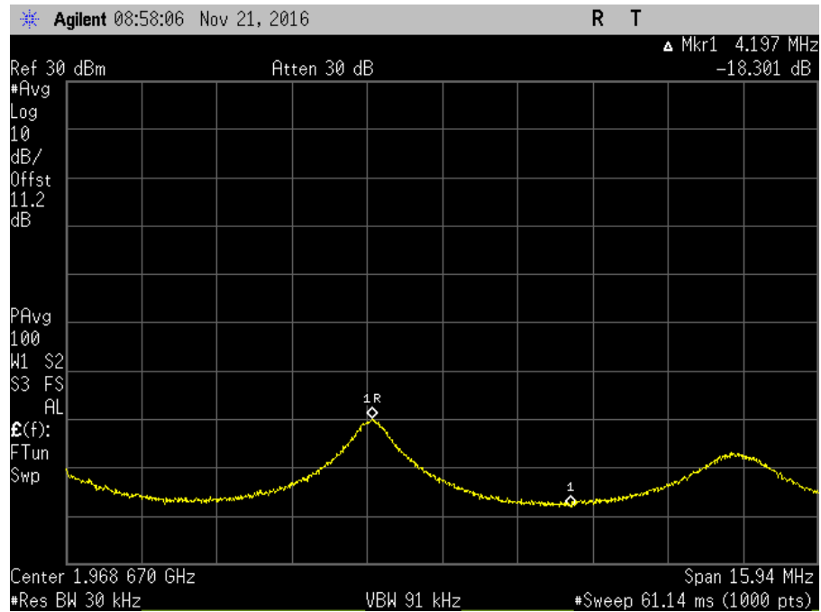
7.11.3_Osc_DL_1930-1995MHz+0_AWGNL
