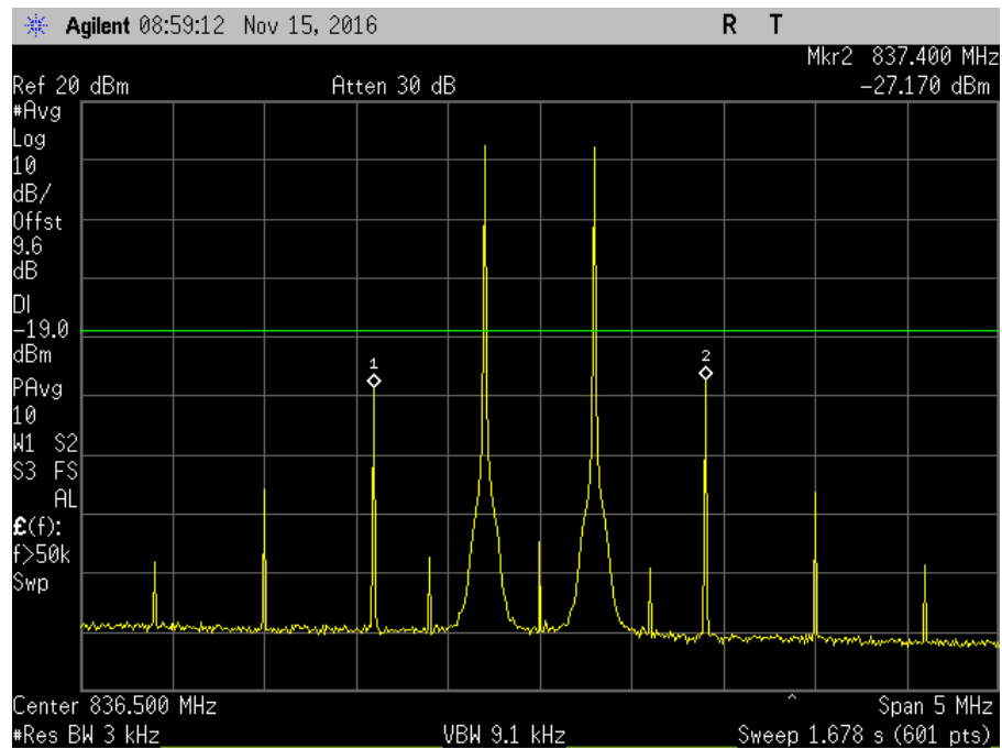
7.4_Intermod_UL_824-849MHz
