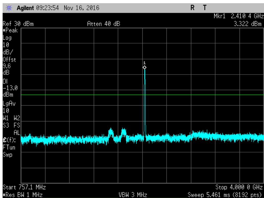
7.6_CSE_DL_746-757MHz_R4
