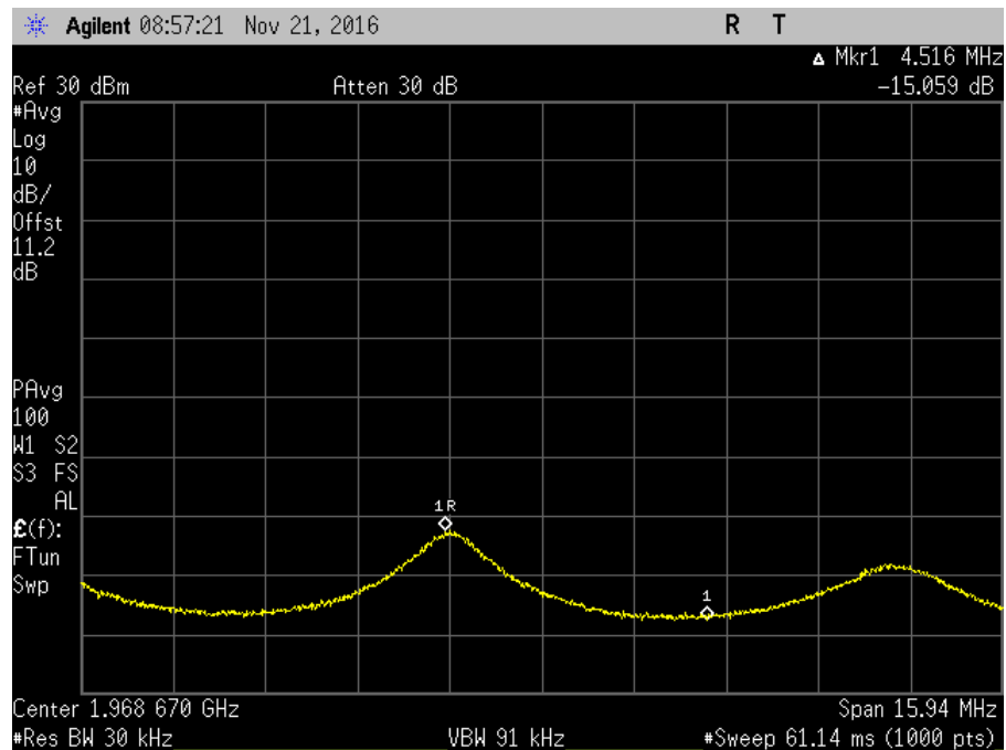
7.11.3_Osc_DL_1930-1995MHz+1_AWGNL
