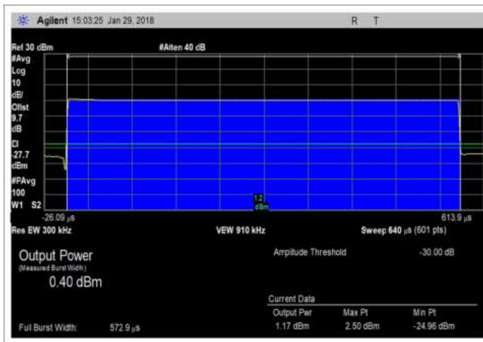
DL_868-894_GSM_max
