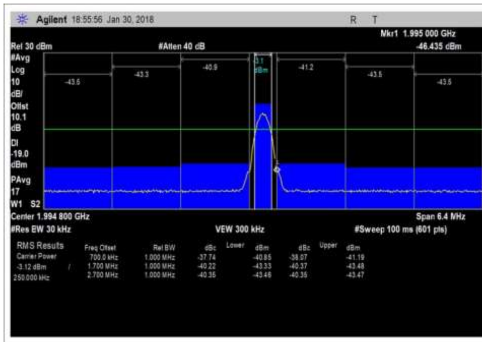
DL_1930-1995MHz_GSM_H
