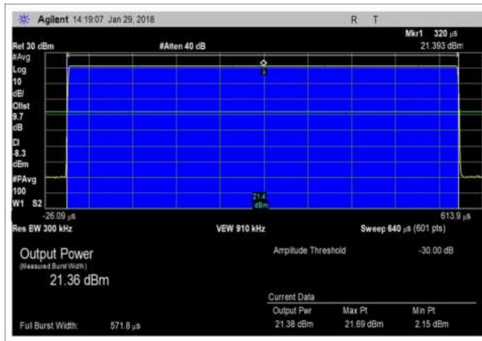
UL_824-849MHz_GSM
