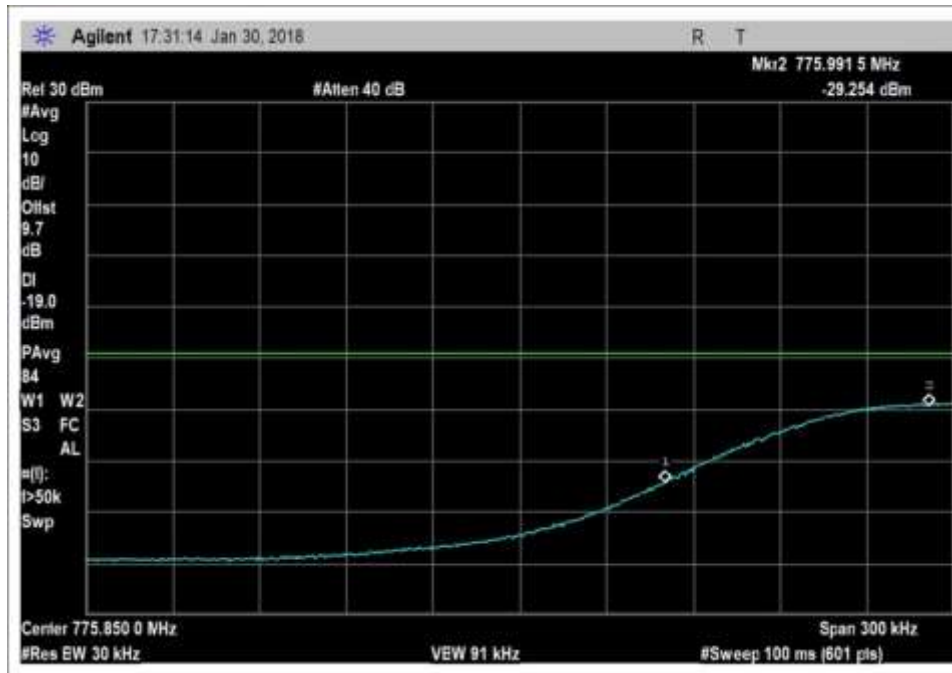
UL_776-787MHz_GSM_L_rbw=30kHz
