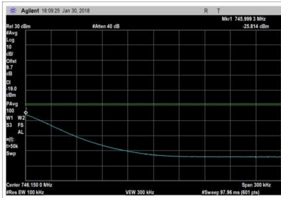
DL_728-746MHz_GSM_H_rbw=100kHz
