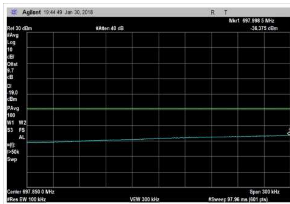
UL_698-716MHz_CDMA_L
