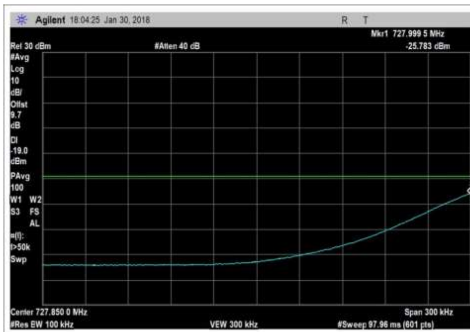
DL_728-746MHz_GSM_L_rbw=100kHz
