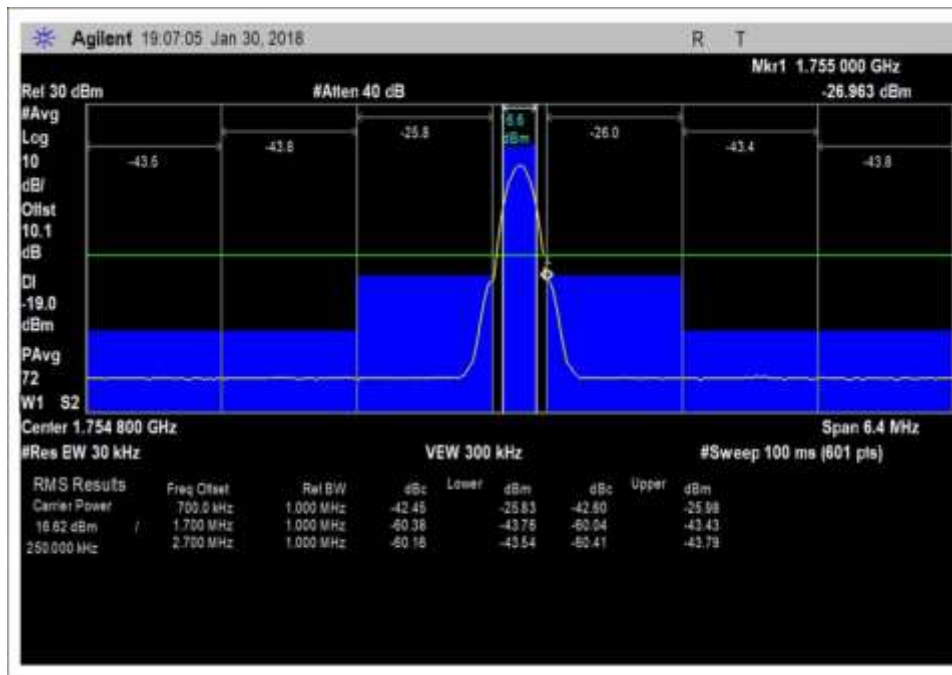
UL_1710-1755MHz_GSM_H
