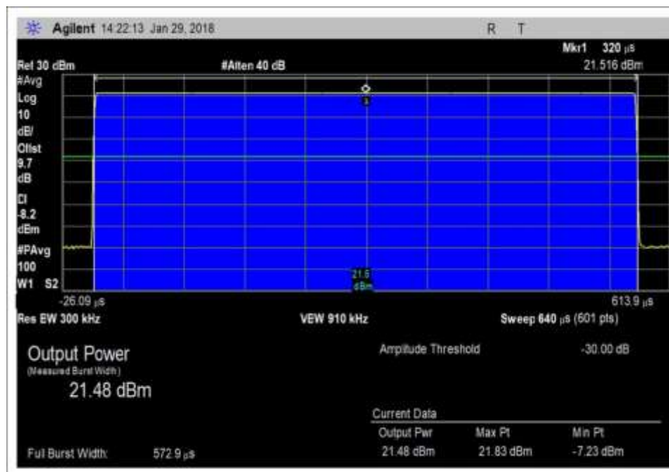
UL_824-849MHz_GSM_Max
