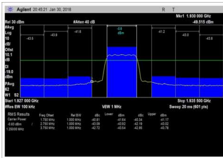
DL_1930-1995MHz_CDMA_L
