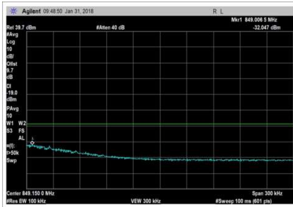
UL_824-849MHz_LTE_H
