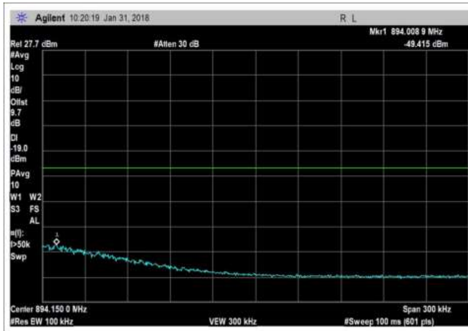
DL_869-894MHz_LTE_H
