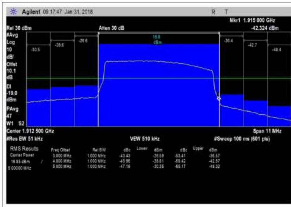
UL_1850-1915MHz_LTE_H
