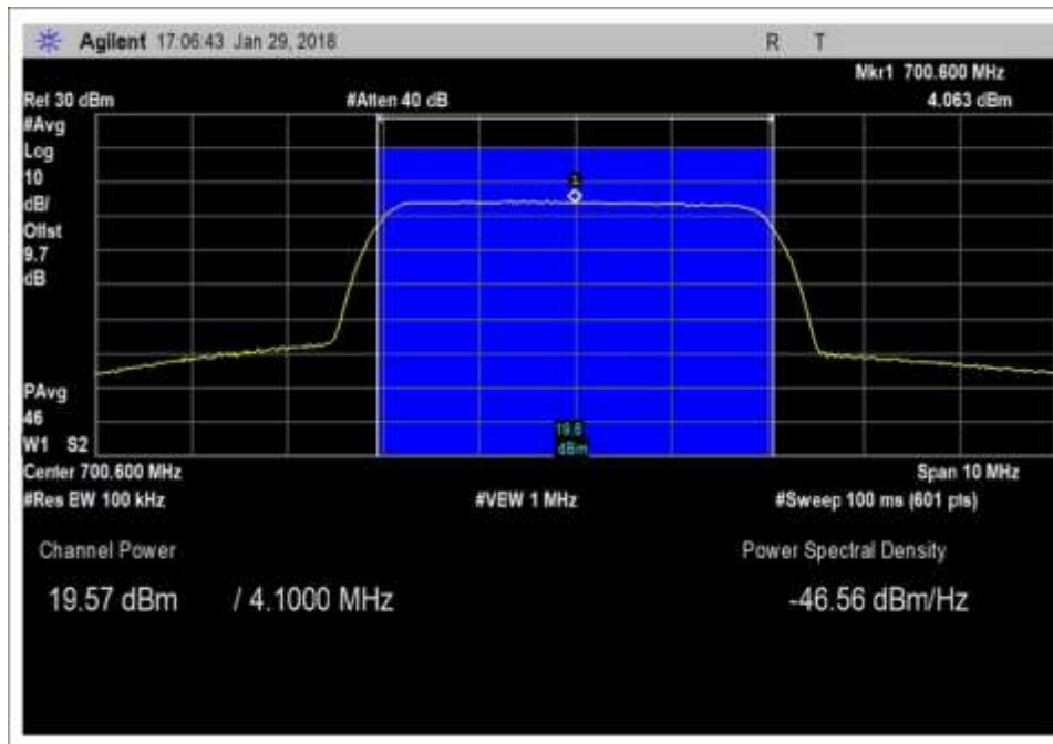
UL_698-716MHz_AWGN
