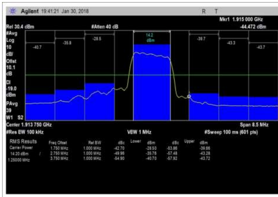
UL_1850-1915MHz_CDMA_H
