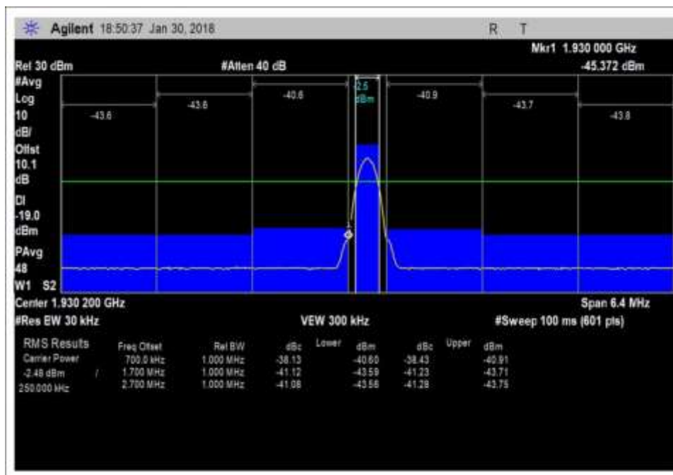
DL_1930-1995MHz_GSM_L
