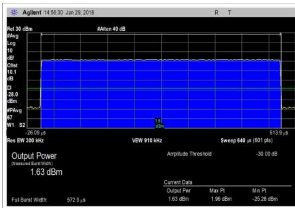
DL_1930-1995_GSM_max
