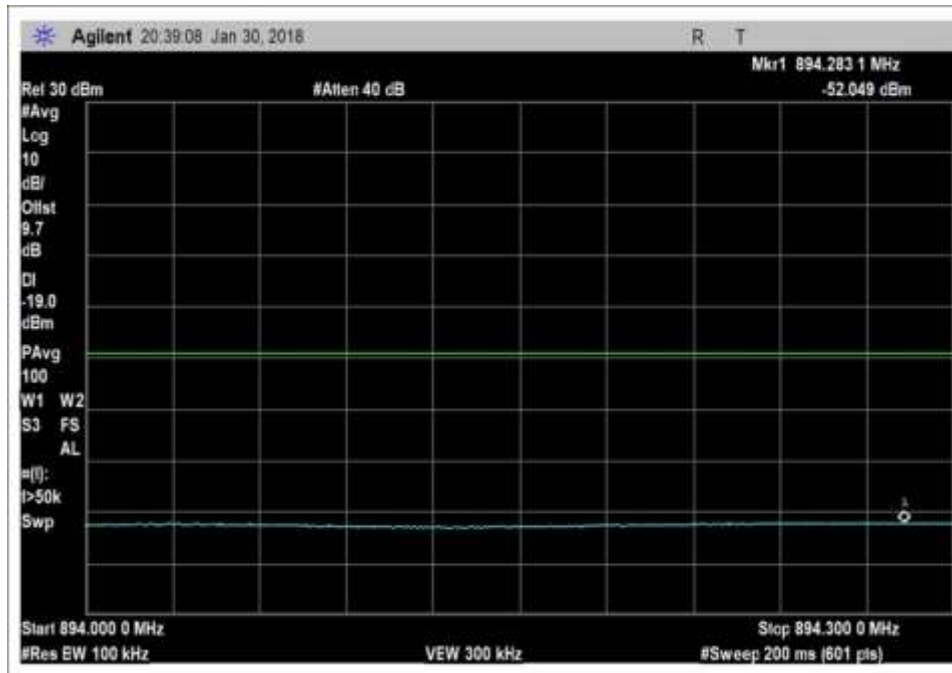
DL_869-894MHz_CDMA_H
