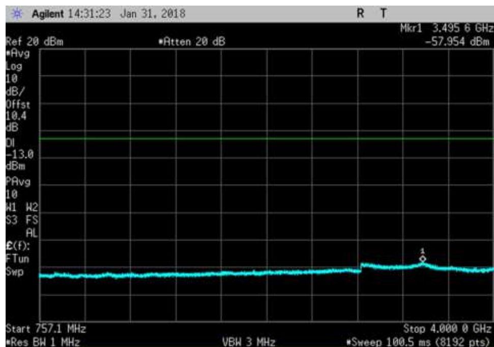
DL_746-757_ 757.1- 4000MHz
