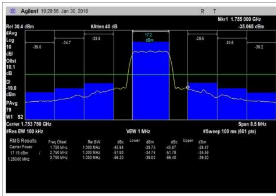
UL_1710-1755MHz_CDMA_H
