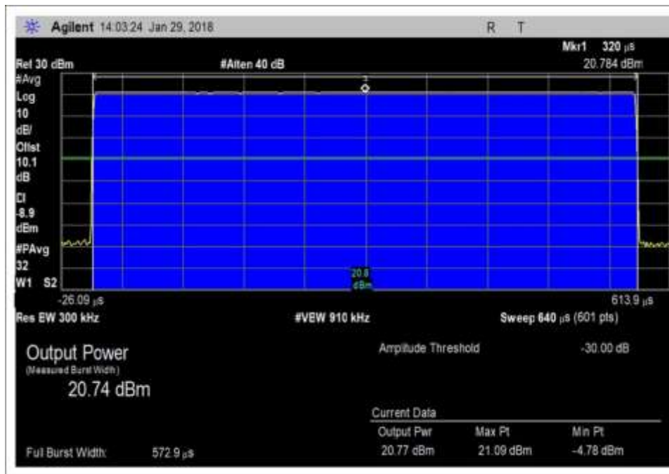
UL_1710-1755MHz_GSM
