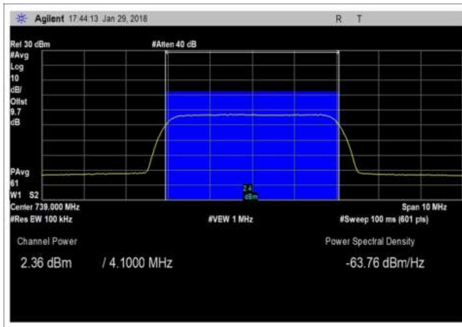
DL_728-746MHz_AWGN
