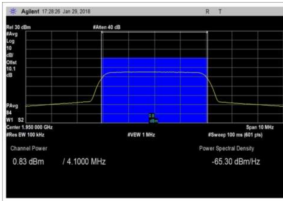
DL_1930-1995MHz_AWGN.
