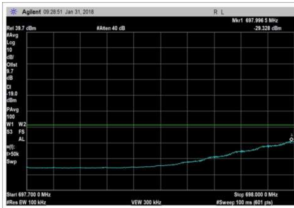
UL_698-716MHz_LTE_L
