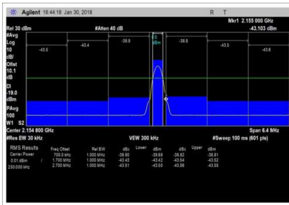
DL_2110-2155MHz_GSM_H
