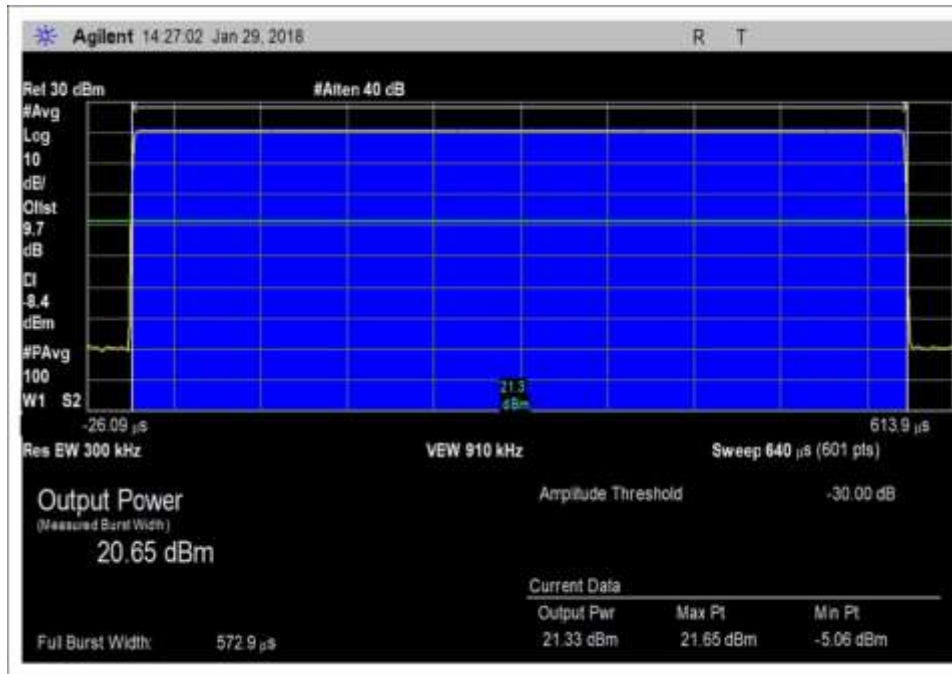
UL_698-716_GSM_max
