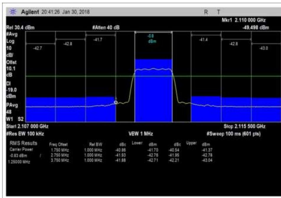
DL_2110-2155MHz_CDMA_L
