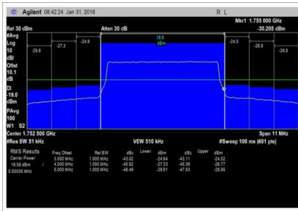
UL_1710-1755MHz_LTE_H
