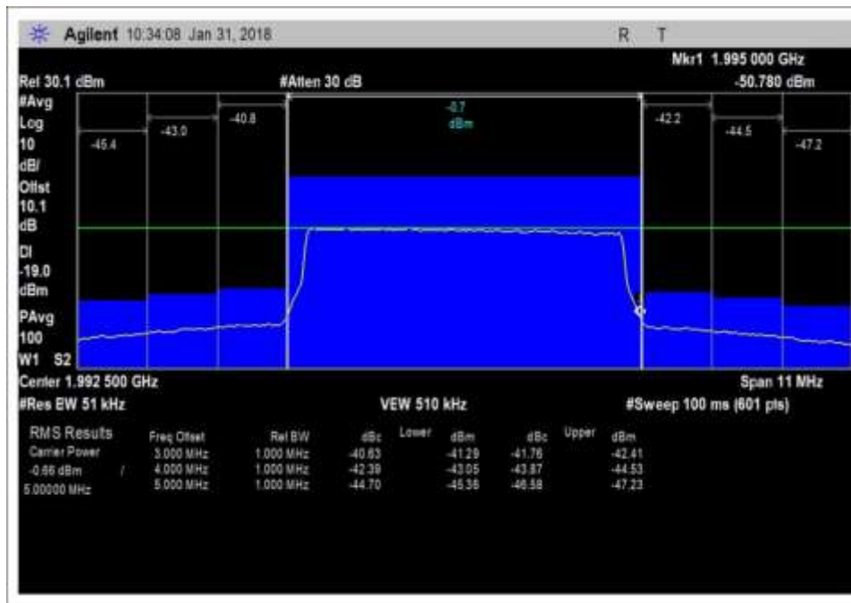
DL_1930-1995MHz_LTE_H
