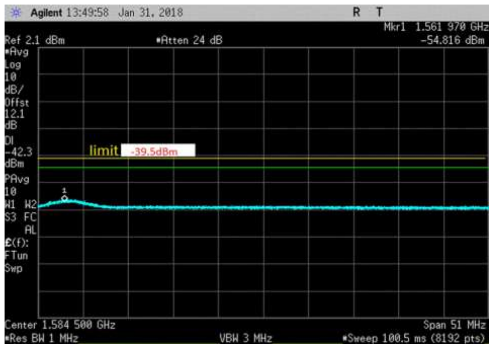
UL_776-787_ 1559- 1610MHz_gps
