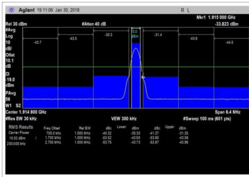
UL_1850-1915MHz_GSM_H
