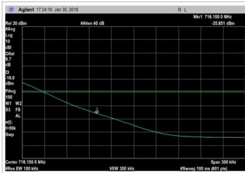
UL_698-716MHz_GSM_H_rbw=100kHz
