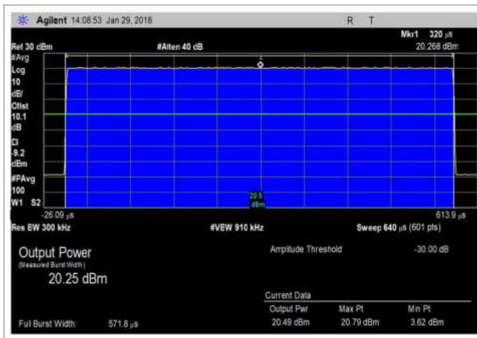
UL_1710-1755MHz_GSM_max
