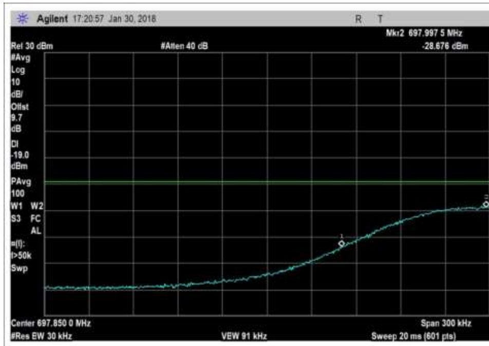
UL_698-716MHz_GSM_L_rbw=30kHz
