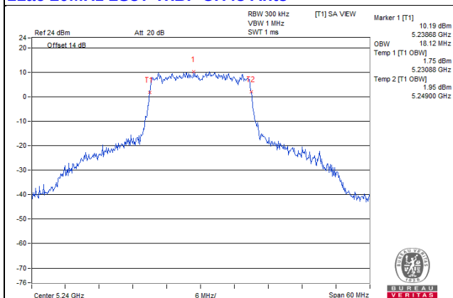
11ac 20MHz 2S3T TxBF CH48 Ant3
