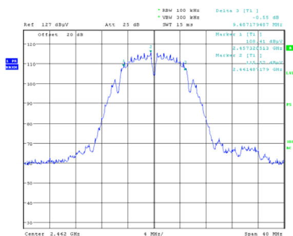
802.11b 2462MHz
