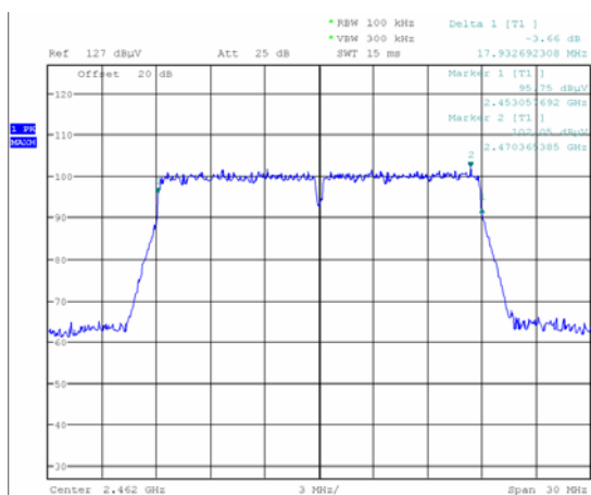
802.11n(HT20) 2462MHz
