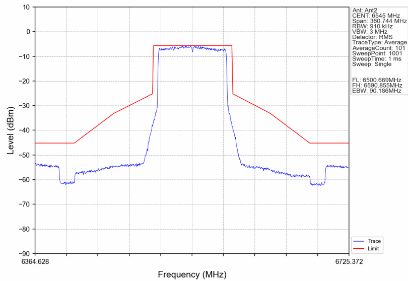
802.11be(EHT80)_HCH_6545MHz_RU996_Left_Ant2_NTNV
