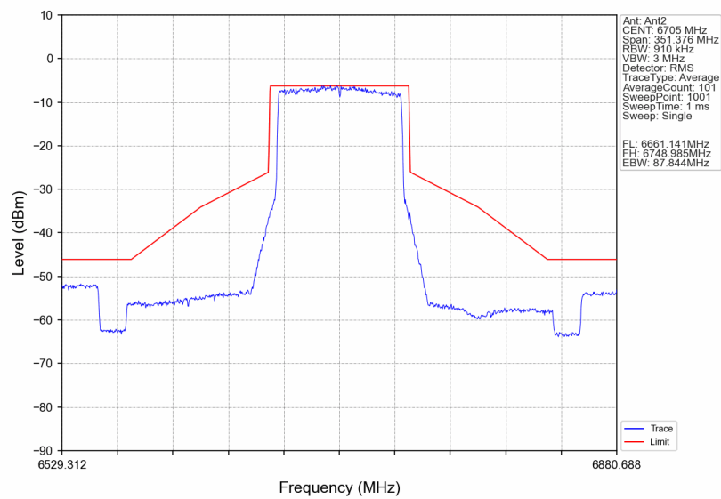
802.11be(EHT80)_MCH_6705MHz_RU996_Left_Ant2_NTNV
