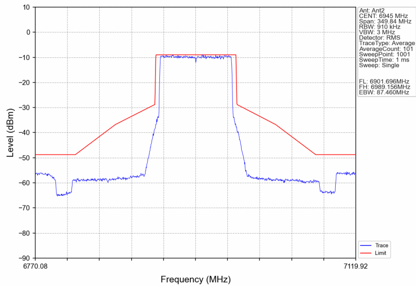
802.11be(EHT80)_LCH_6945MHz_RU996_Left_Ant2_NTNV
