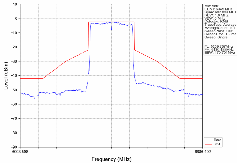
802.11be(EHT160)_HCH_6345MHz_2xRU996_Left_Ant2_NTNV
