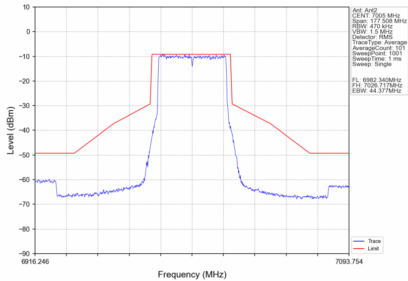
802.11be(EHT40)_MCH_7005MHz_RU484_Left_Ant2_NTNV
