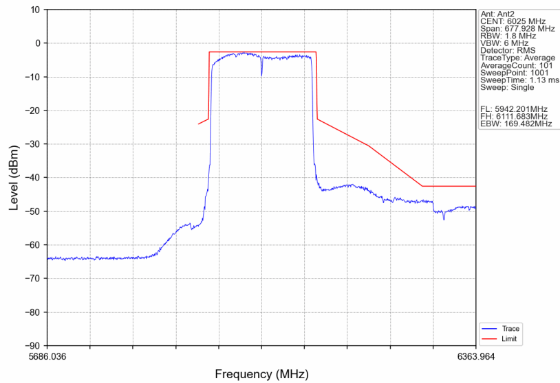
802.11be(EHT160)_LCH_6025MHz_2xRU996_Left_Ant2_NTNV
