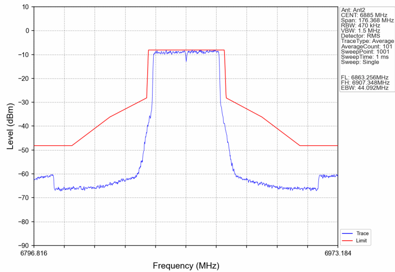
802.11be(EHT40)_HCH_6885MHz_RU484_Left_Ant2_NTNV
