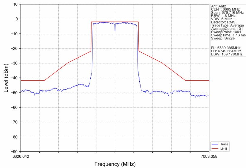
802.11be(EHT160)_MCH_6665MHz_2xRU996_Left_Ant2_NTNV
