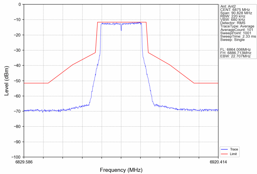
802.11be(EHT20)_HCH_6875MHz_RU242_Left_Ant2_NTNV
