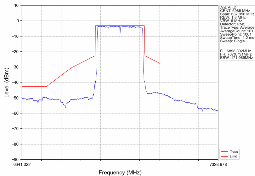
802.11be(EHT160)_MCH_6985MHz_2xRU996_Left_Ant2_NTNV
