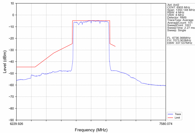
802.11be(EHT320)_HCH_6905MHz_4xRU996_Left_Ant2_NTNV
