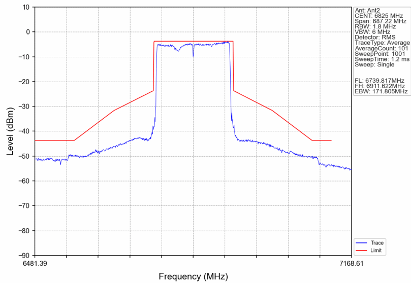
802.11be(EHT160)_HCH_6825MHz_2xRU996_Left_Ant2_NTNV
