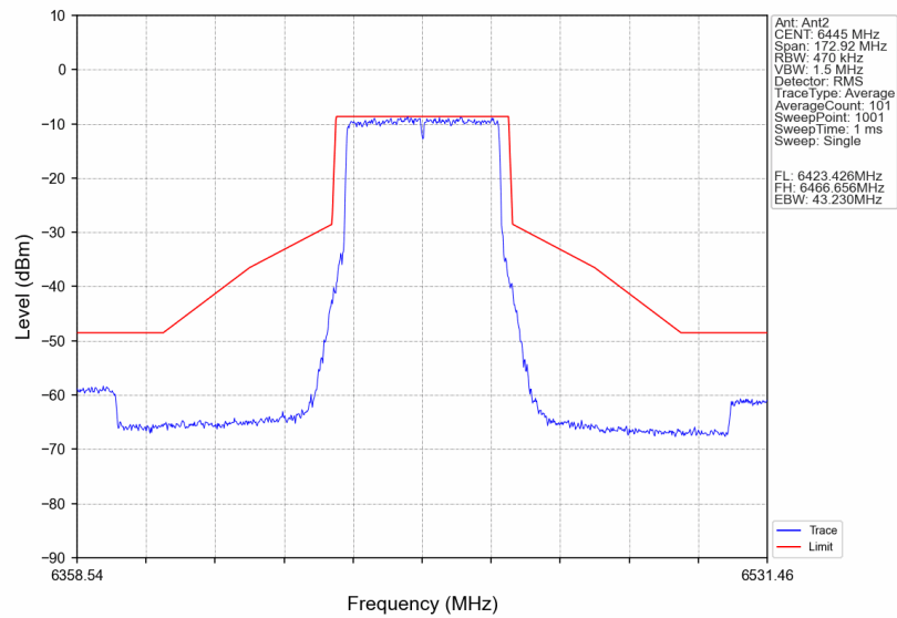
802.11be(EHT40)_LCH_6445MHz_RU484_Left_Ant2_NTNV
