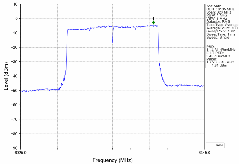
802.11be(EHT160)_MCH_6185MHz_2xRU996_Left_Ant2_NTNV
