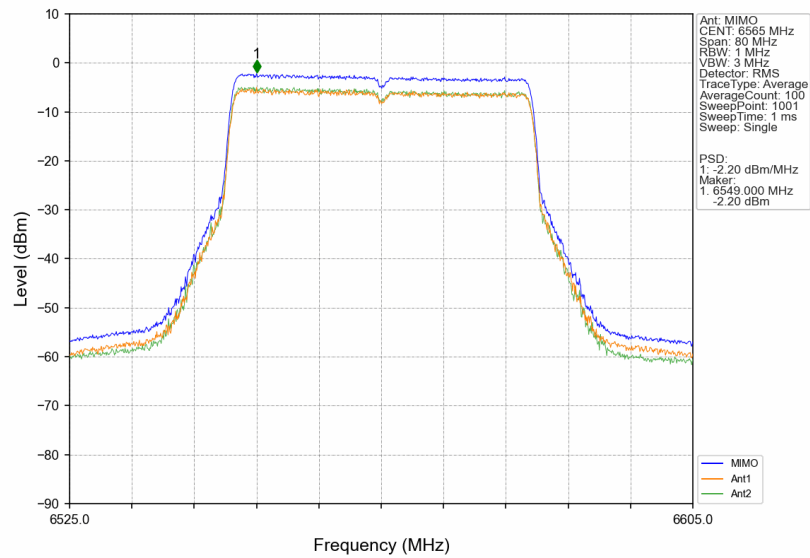
802.11be(EHT40)_LCH_6565MHz_RU484_Left_MIMO_NTNV
