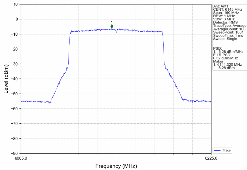
802.11be(EHT80)_MCH_6145MHz_RU996_Left_Ant1_NTNV
