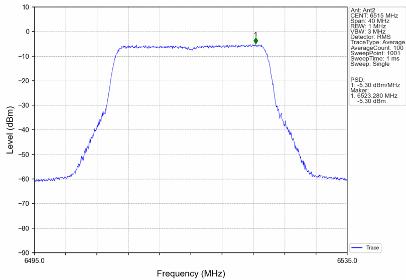
802.11be(EHT20)_HCH_6515MHz_RU242_Left_Ant2_NTNV
