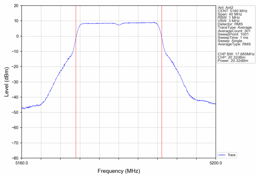
802.11a_LCH_5180MHz_Ant2_NTNV
