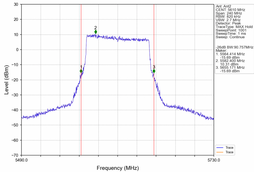
802.11be(EHT80)_HCH_5610MHz_SU_/_Ant2_NTNV
