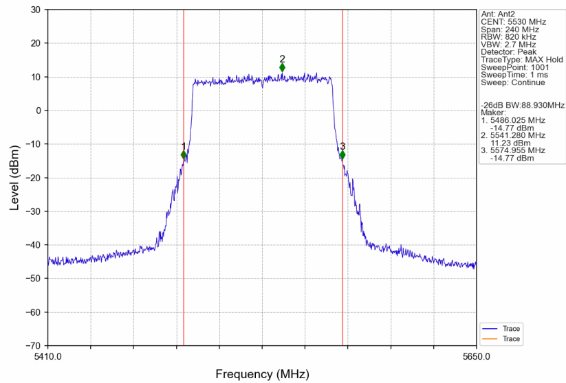
802.11be(EHT80)_LCH_5530MHz_SU_/_Ant2_NTNV
