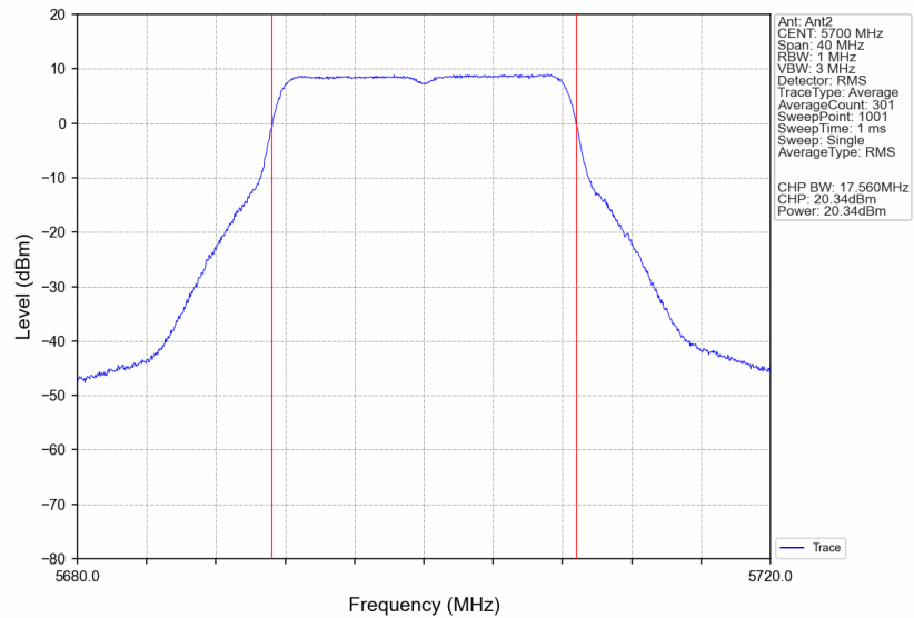
802.11a_HCH_5700MHz_Ant2_NTNV
