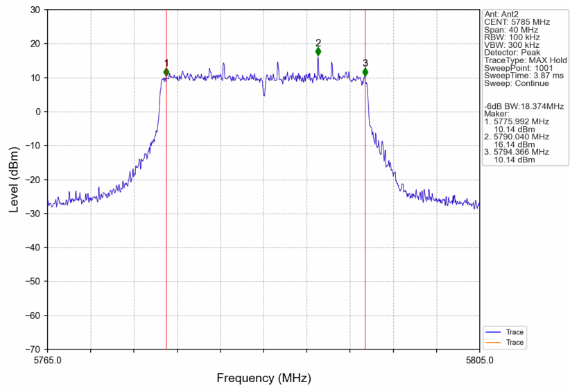
802.11be(EHT20)_MCH_5785MHz_SU_/_Ant2_NTNV
