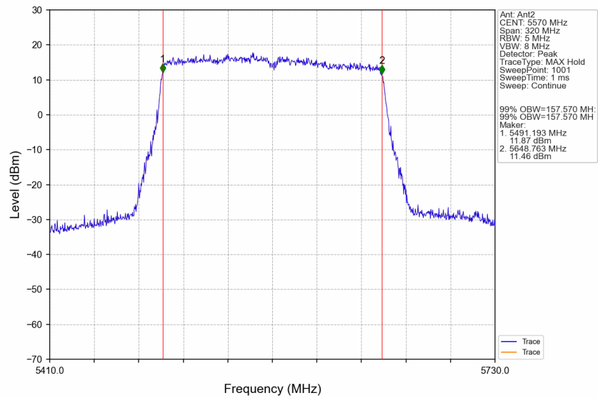
802.11be(EHT160)_MCH_5570MHz_SU_/_Ant2_NTNV
