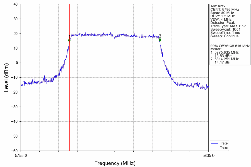
802.11be(EHT40)_HCH_5795MHz_SU_/_Ant2_NTNV
