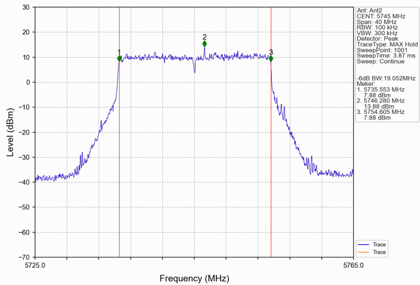
802.11be(EHT20)_LCH_5745MHz_SU_/_Ant2_NTNV
