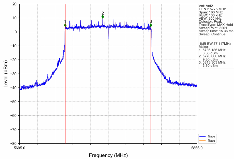
802.11be(EHT80)_MCH_5775MHz_SU_/_Ant2_NTNV
