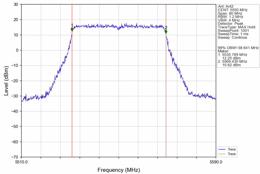
802.11be(EHT40)_MCH_5550MHz_SU_/_Ant2_NTNV
