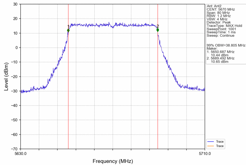
802.11be(EHT40)_HCH_5670MHz_SU_/_Ant2_NTNV
