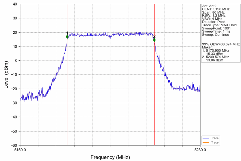
802.11be(EHT40)_LCH_5190MHz_SU_/_Ant2_NTNV
