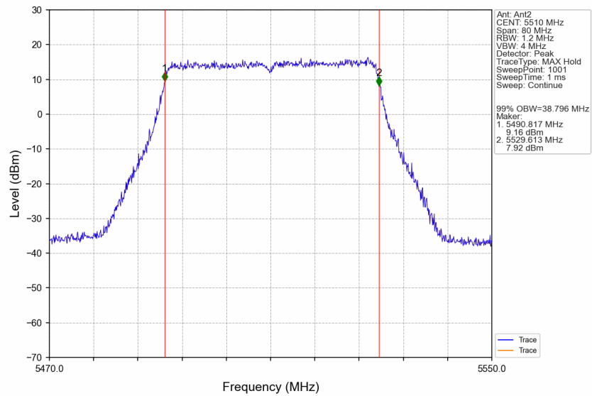
802.11be(EHT40)_LCH_5510MHz_SU_/_Ant2_NTNV
