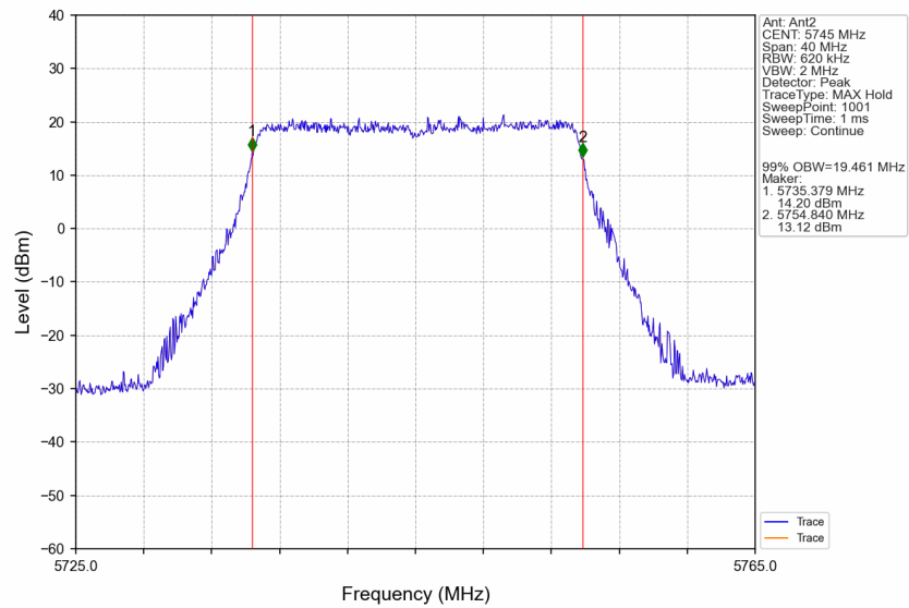
802.11be(EHT20)_LCH_5745MHz_SU_/_Ant2_NTNV
