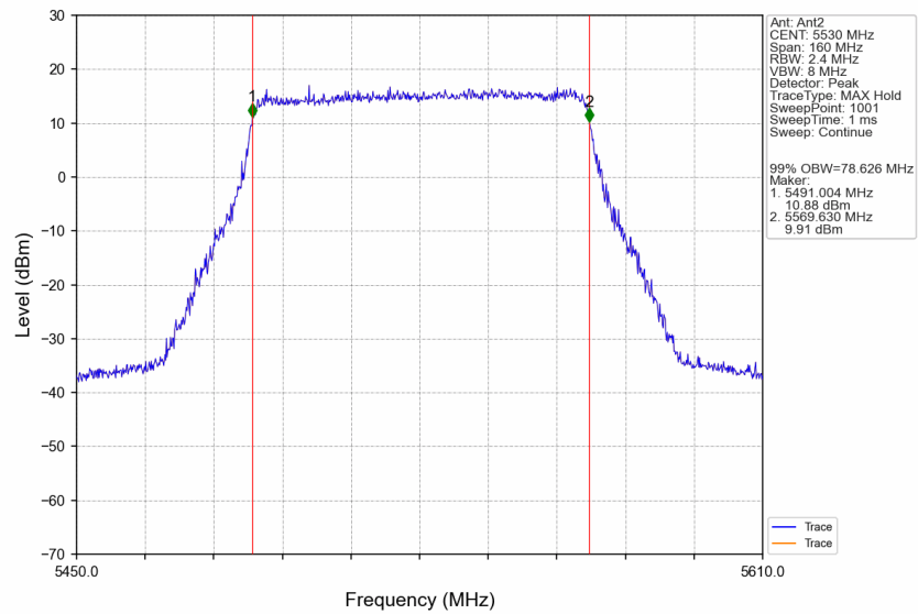
802.11be(EHT80)_LCH_5530MHz_SU_/_Ant2_NTNV
