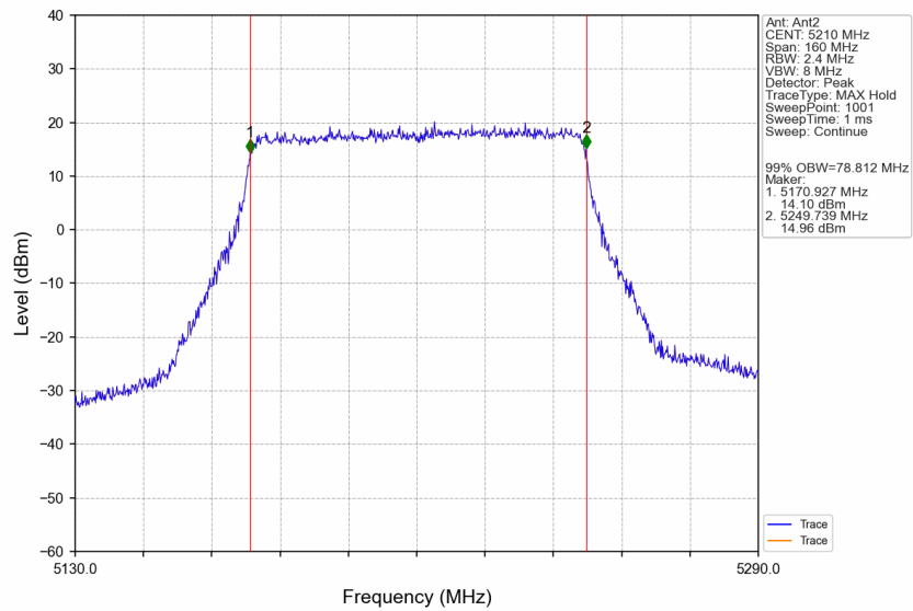
802.11be(EHT80)_MCH_5210MHz_SU_/_Ant2_NTNV
