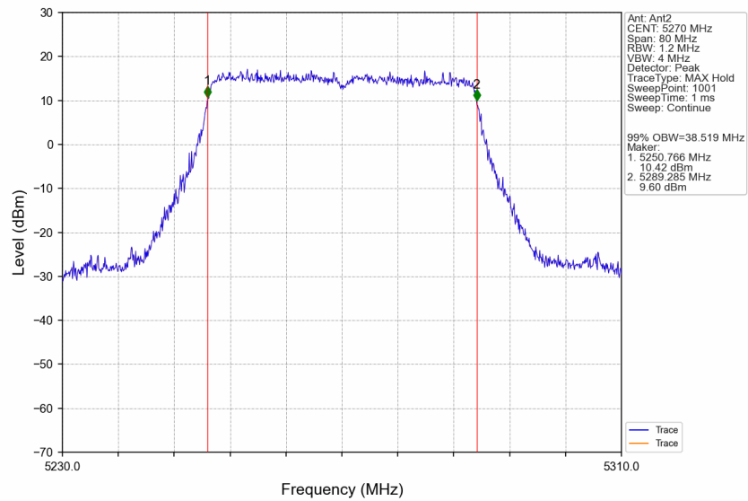
802.11be(EHT40)_LCH_5270MHz_SU_/_Ant2_NTNV
