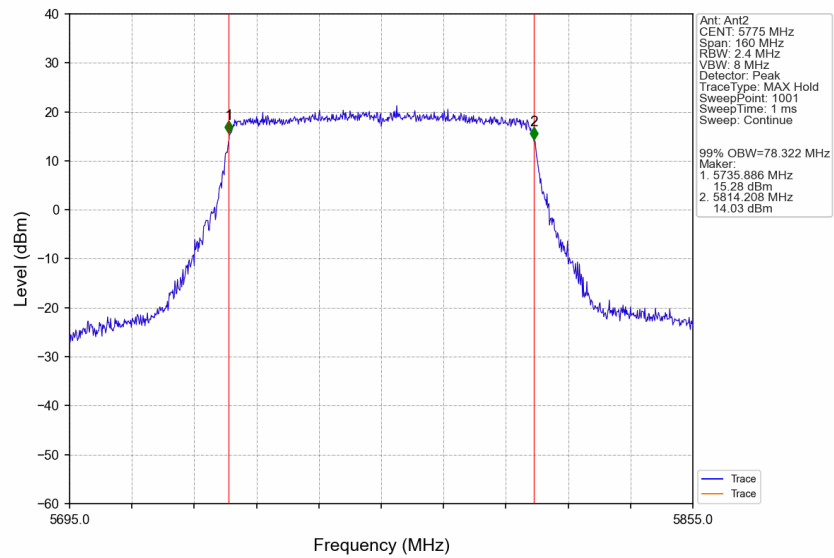
802.11be(EHT80)_MCH_5775MHz_SU_/_Ant2_NTNV
