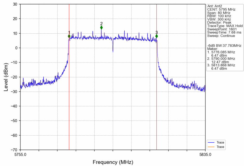
802.11be(EHT40)_HCH_5795MHz_SU_/_Ant2_NTNV
