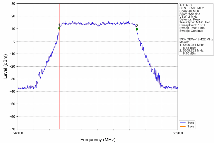
802.11be(EHT20)_LCH_5500MHz_SU_/_Ant2_NTNV
