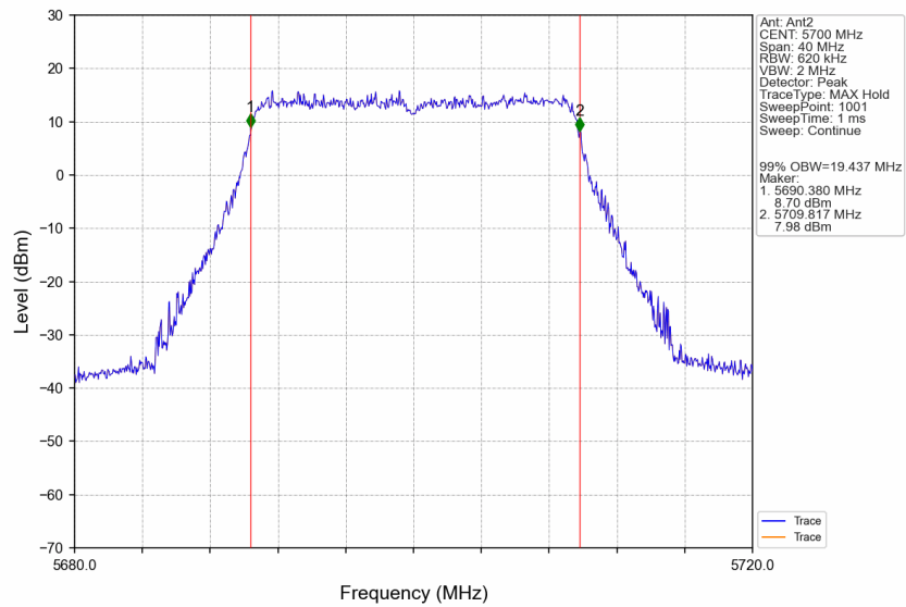
802.11be(EHT20)_HCH_5700MHz_SU_/_Ant2_NTNV
