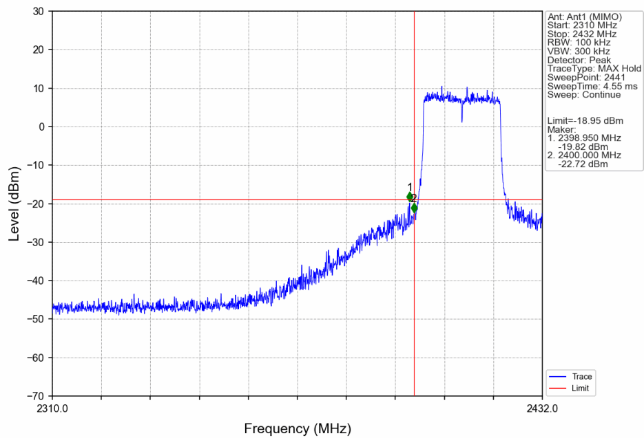
802.11ax(HEW20)_LCH_2412MHz_SU_/_Ant1 (MIMO)_NTNV
