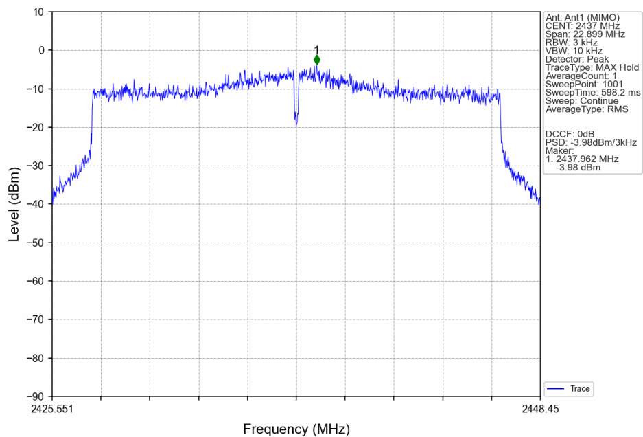
802.11be(EHT20)_MCH_2437MHz_SU_/_Ant1 (MIMO)_NTNV
