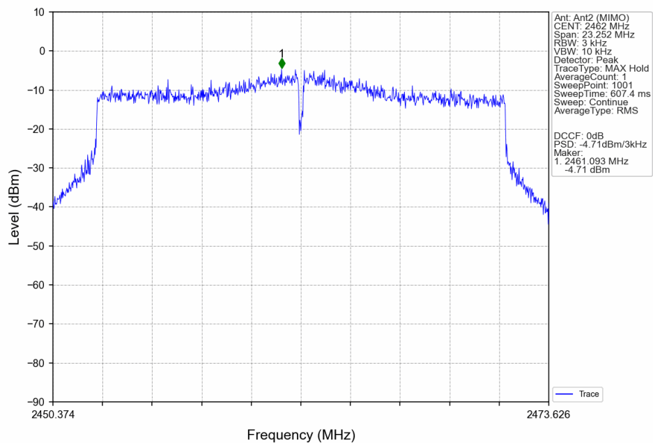
802.11be(EHT20)_HCH_2462MHz_SU_/_Ant2 (MIMO)_NTN
