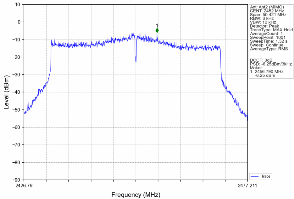
802.11be(EHT40)_HCH_2452MHz_SU / _MIMO_NTN
