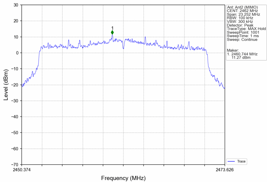
802.11be(EHT20)_HCH_2462MHz_SU_/_Ant2 (MIMO)_NTNV
