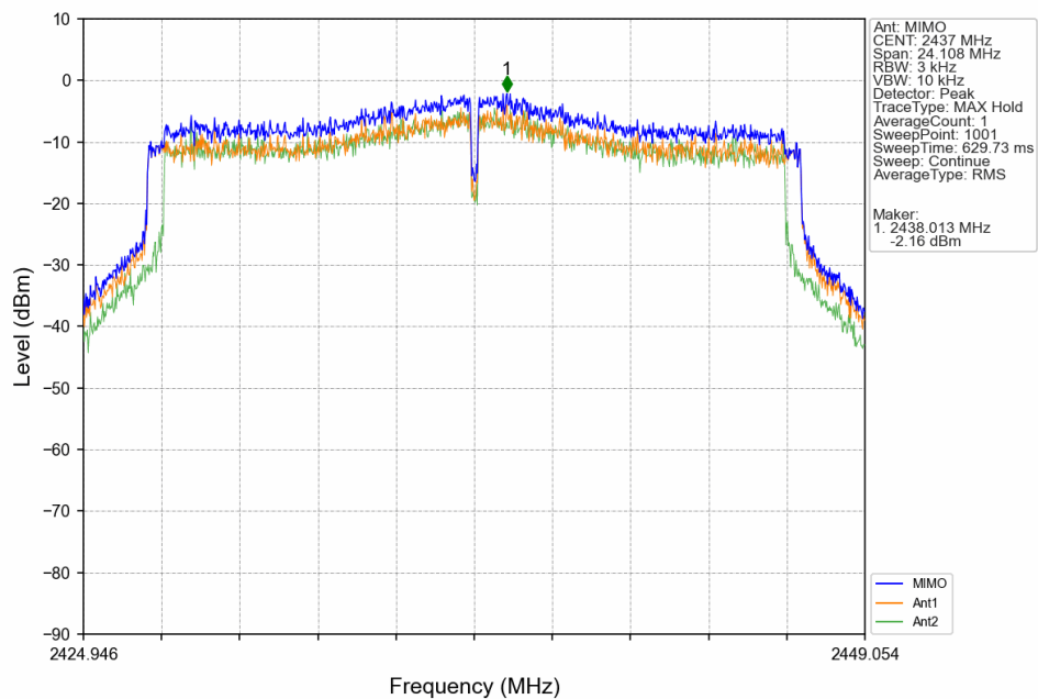
802.11be(EHT20)_MCH_2437MHz_SU / _MIMO_NTN
